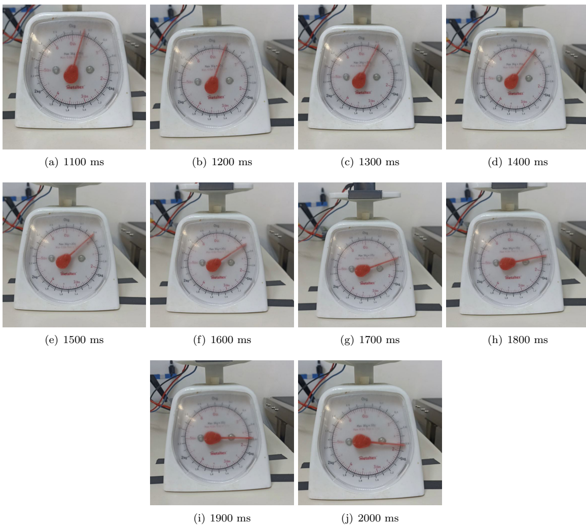
Figura 2: Medición de empuje
