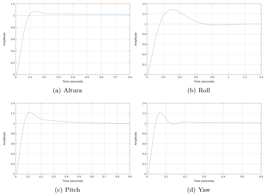
Figura 6: Respuesta escalón PID
