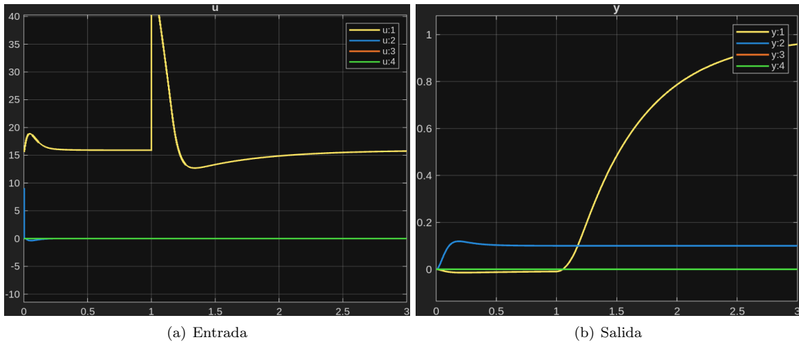
Figura 8: Simulación PD, controlador a 510 Hz
