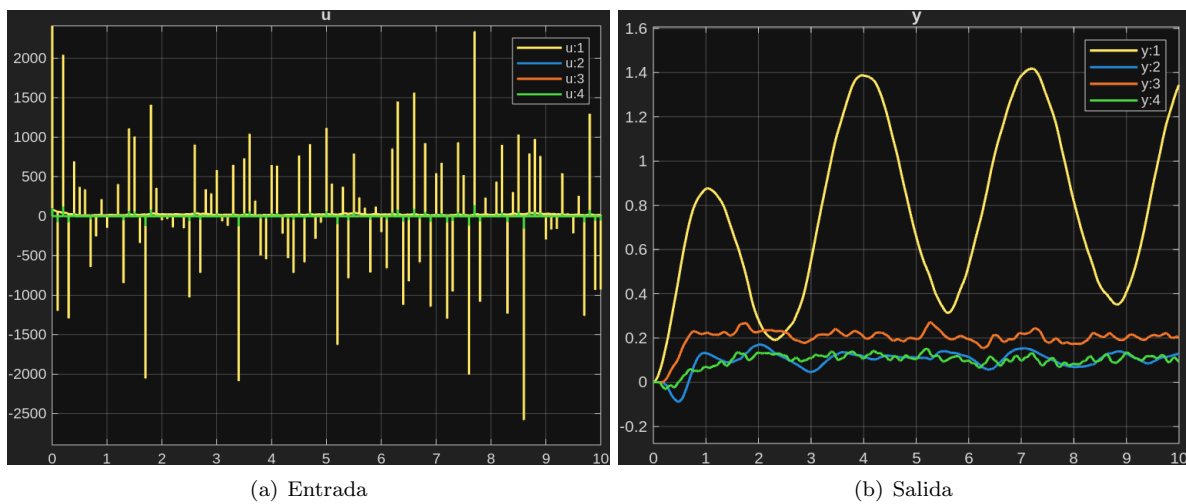
Figura 10: Simulación PID, controlador a 510 Hz
