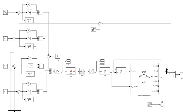
Figura 9: PID en Simulink
