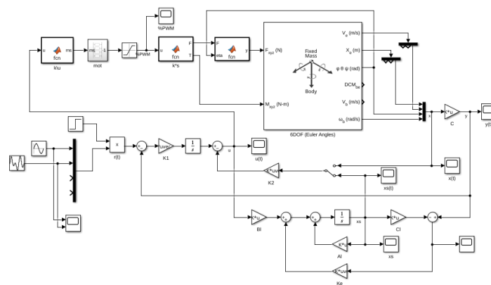
Figura 11: LQI en Simulink
