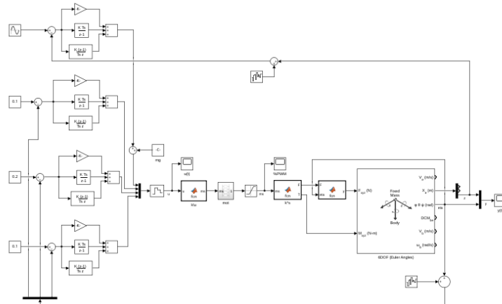
Figura 6: PID en Simulink
