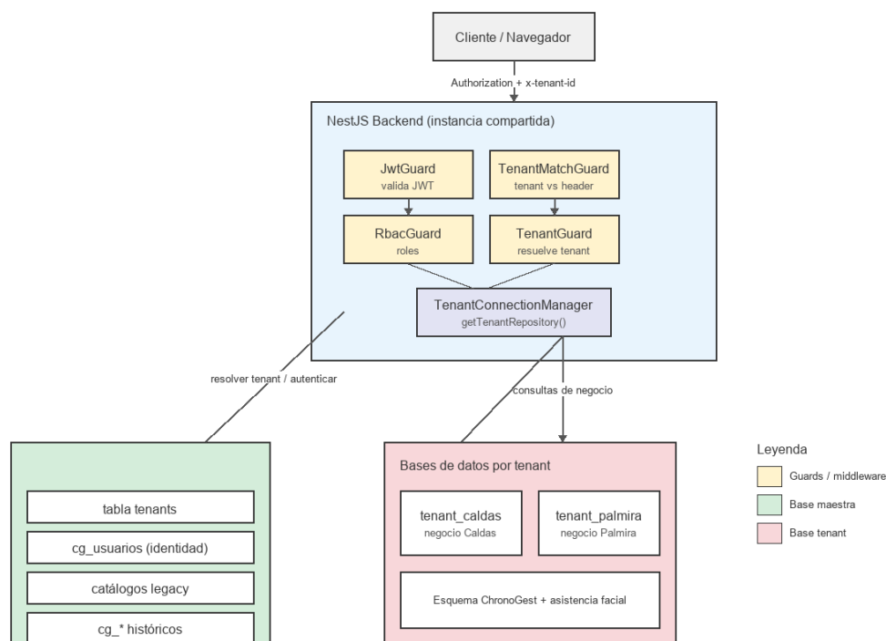
Arquitectura multitenancy — Chronogest
