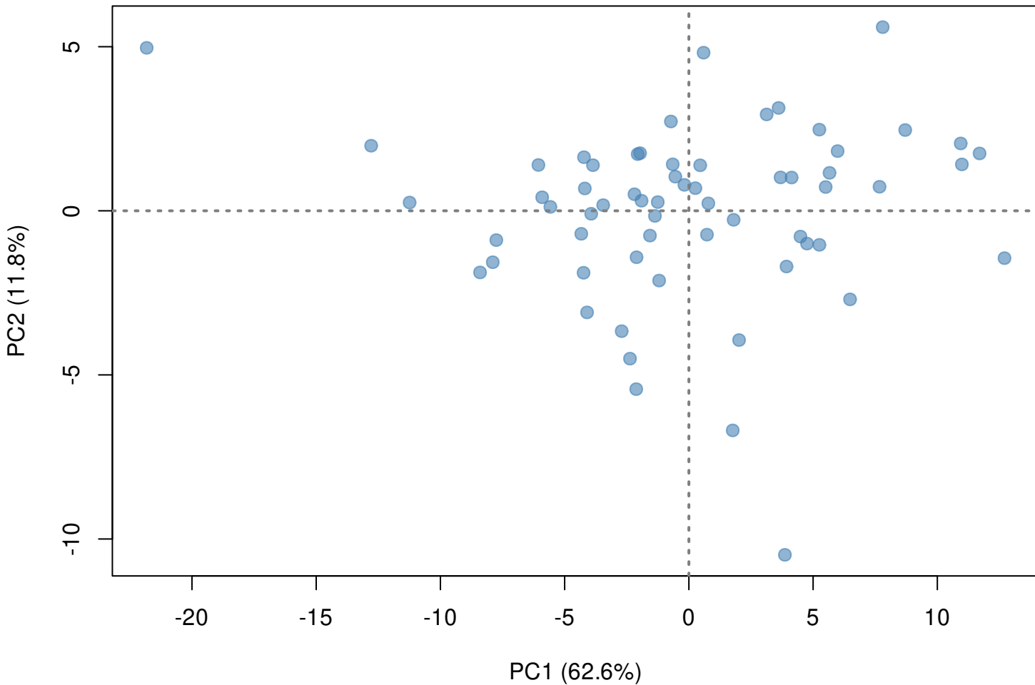
fPCA Scores: PC1 vs PC2
