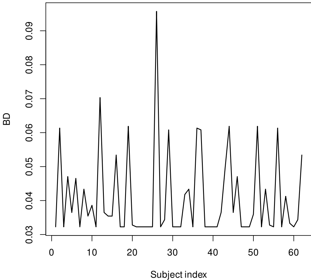
Band Depth (BD)
