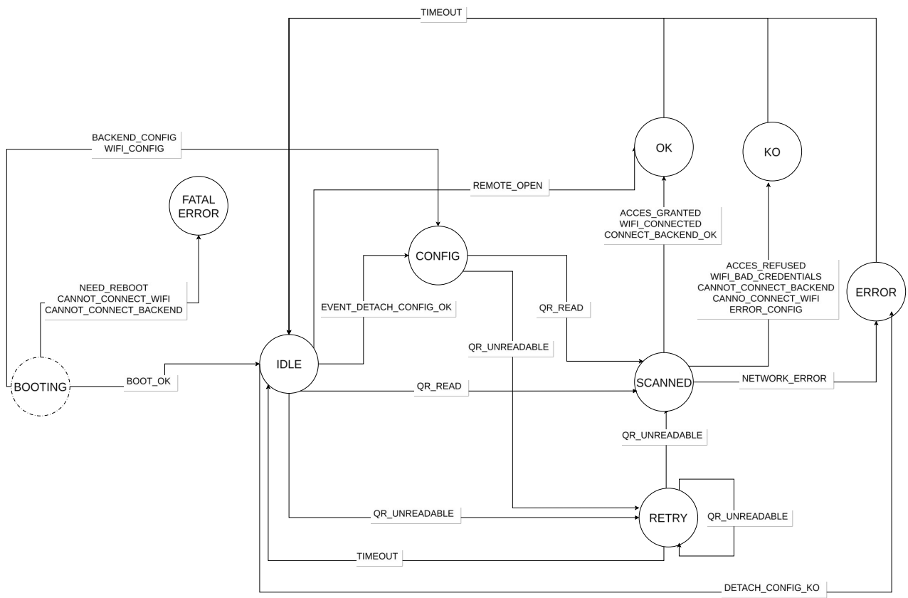
Diagramme de la machine à états et des différentes transitions
