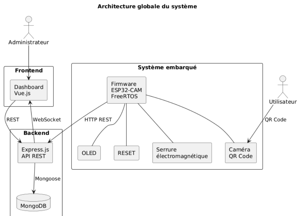
Diagramme des différents composants de la plateforme
