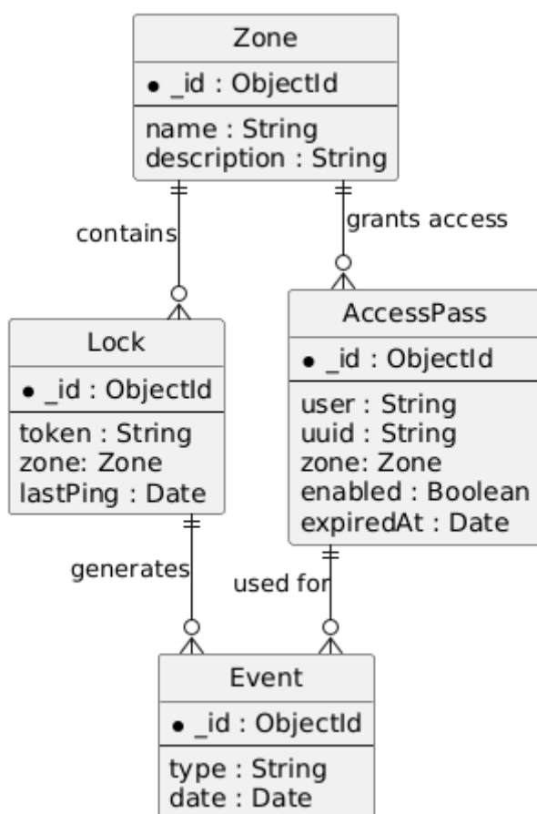
Diagramme ERD du backend
