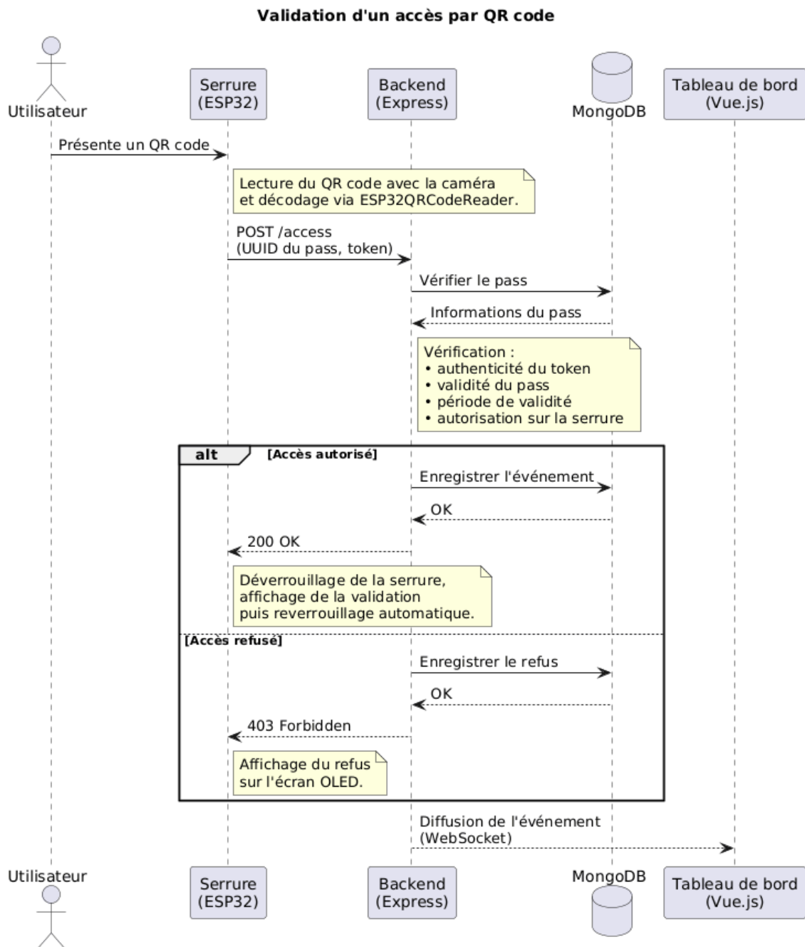
Diagramme de séquence pour le flow d'accès À un espace contrôlé par le dispositif
