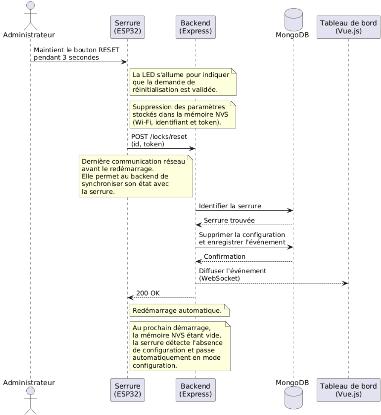
Diagramme de séquence pour le flow De réinitialisation du dispositif
