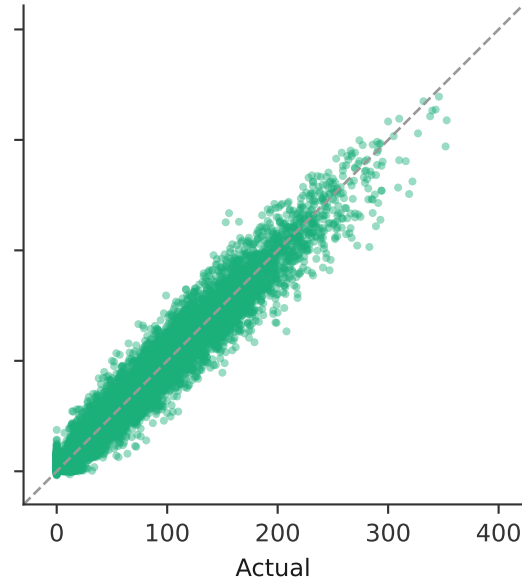
GRU R^2=0.956
