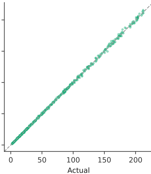
GRU R^2=1.000
