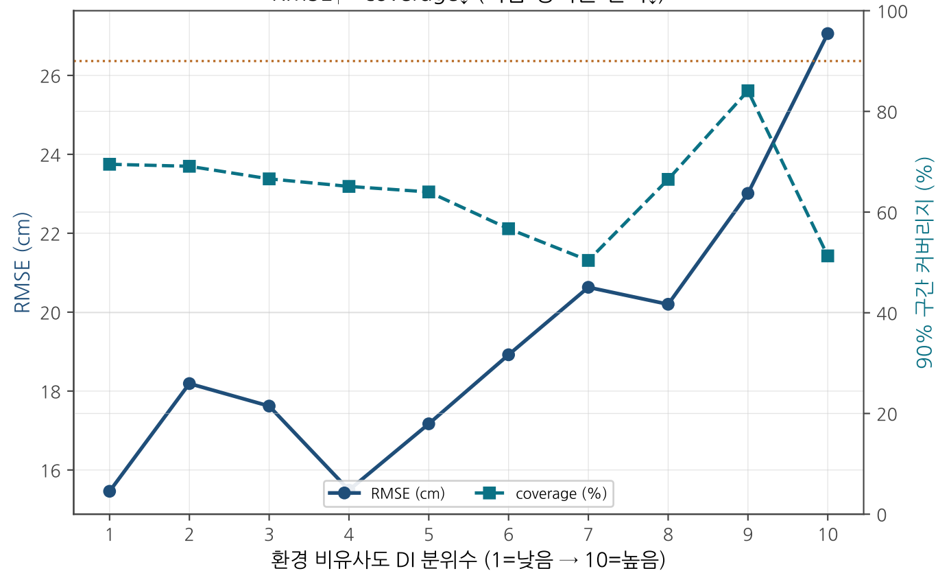
transfer AOA — 학습환경에서 멀어질수록(DI↑) RMSE↑ · coverage↓ (외삽 영역은 신뢰↓)
