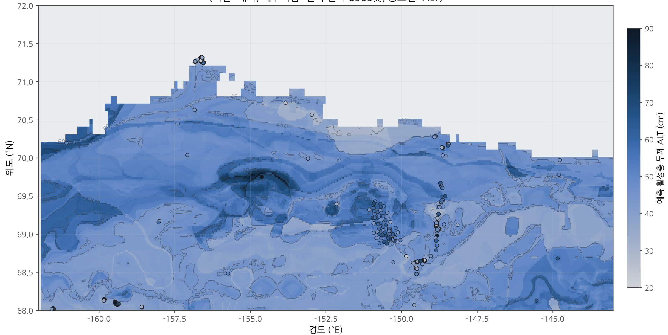
알래스카 북서면 활성층 두께(ALT) 예측 표면 (연속 2D 레이어) (색면=예측, 테두리점=실측 관측 8965곳, 등고선=ALT)
