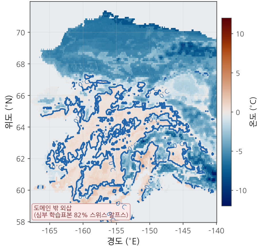
깊이 20 m 연평균 지중온도
