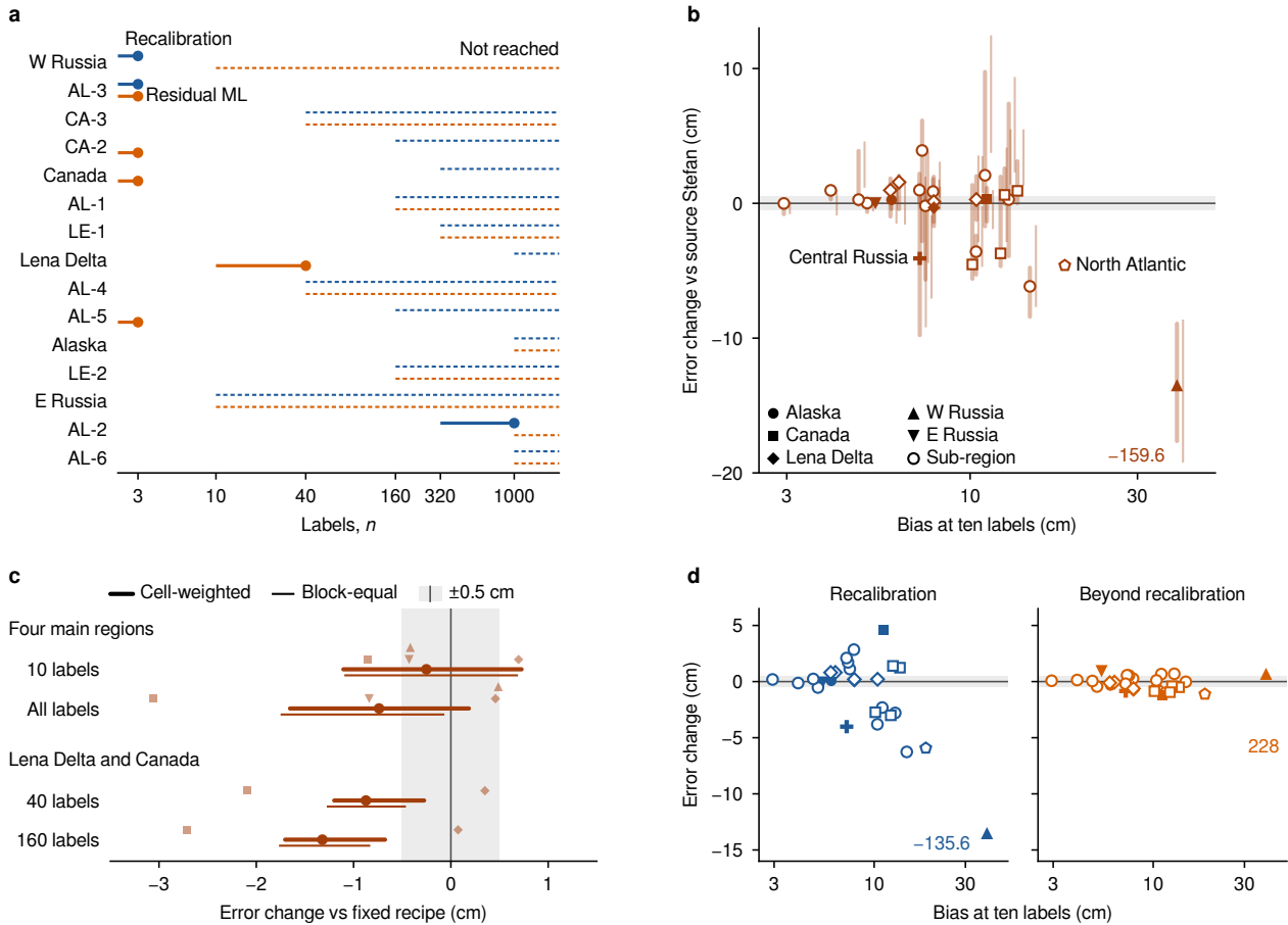
그림 5. 라벨을 쓰는 보정의 오차 감소는 라벨 10 개로 전 원천 계수 편향과 순위상관을 보였다. (a) 재보정이 원천 계수 Stefan 식보다 오차를 낮춘 (Recalibration) 시험 라벨 수의 최솟값 n^* 와, 잔차 ML 이 재보정 모델보다 오차를 낮춘 (Residual ML) n^* (앞 격자 값부터의 구간). 판정은 등록된 세 조건을 따른다 (방법). Not reached 는 시험한 가장 큰 라벨 수까지 n^* 가 없는 대상이다. 행은 b 의 라벨 10 개 편향 순서이며, 하위 지역은 독립이 아니다. (b) 대상 라벨 안 교차검증으로 고른 방법의 오차 변화 (라벨 전량, 원천 계수 Stefan 식 기준) 를 처음 라벨 10 개에서 그 모델이 보인 평균 편향의 절댓값에 대해 그렸다 (Spearman \rho = 0.38 , 95% CI [0.17, 0.55], 28 대상; 부호 있는 편향은 \rho = -0.01 ). 티베트 고원은 축 밖에 있으며 (편향 227.7 cm; 오차 변화는 b 에서 -159.6 cm, d 에서 -135.7 cm 와 -5.9 cm), 북대서양은 점 추정이다. (c) 교차검증 선정에서 고정 잔차 레시피 ( \lambda = 0.25 ) 를 뺀 값. 선정은 레나델타와 캐나다 평균의 라벨 40 개와 160 개에서 비열 등이었고 (한계 0.5 cm), 라벨 160 개에서 오차가 1.3 cm 낮았다. 라벨 40 개의 0.87 cm 감소와 라벨 전량의 비열등은 분할 독립 가정에 의존하며, 라벨 10 개에서는 비열등이 성립하지 않았다. 이득은 캐나다에서 왔고 (2.1 cm 와 2.7 cm), 레나델타의 변화는 +0.35 cm 와 +0.07 cm 였다. (d) 라벨 전량에서 재보정의 오차 변화와, 더 나은 재보정 Stefan 식을 넘어선 잔차 ML 의 오차 변화를 같은 편향에 대해 그렸다. 편향과 재보정 오차 감소의 관계 ( \rho = 0.37 , 95% CI [-0.11, 0.93]) 와 재보정을 넘어선 감소의 관계 ( \rho = 0.28 , [-0.19, 0.80]; 대상 고정 구간 [0.18, 0.54]) 는 확인하지 못했다 (사후 분석). 구간은 0.5° 채점 블록 (d에서는 대상 계열도) 을 10,000 회 재표집한 95% 신뢰구간 (CI) 이며, 범례에 표시한 대로 가중한다. 회색 띠는 \pm 0.5 cm 다. b 와 c 의 분석은 앞선 결과를 본 뒤 설계하였다.
