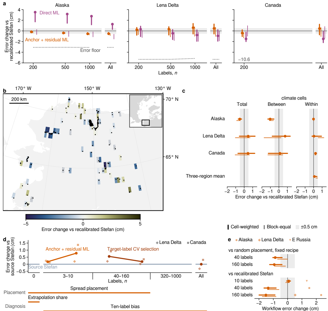
그림 6. 알래스카 안에서 재보정 Stefan 식에 대한 잔차 ML의 이득은 1 cm 미만이었으며, 기후 격자 규모의 편향 보정에서 왔다. (a) 지역 내 시험 (0.5° 블록의 절반을 채점, 분할 25 개). 같은 라벨로 재보정한 Stefan 식 대비 Anchor + residual ML(교차검증 잔차 가중) 과 Direct ML의 오차 변화. Error floor는 공변량 조건부 하한(알래스카 11.31 cm, 레나델타 14.83 cm, 캐나다 17.90 cm)에서 재보정 Stefan RMSE를 뺀 값이며, 캐나다 선 (-10.6 cm부터 -10.8 cm까지)은 축 아래에 있다. 알래스카의 라벨 1000개에서 잔차 모델은 오차가 0.54 cm 낮았다. 라벨 500개와 전량의 감소(0.39 cm와 0.52 cm)는 공통 재표집 구간에서 유지되지 않았다. 레나델타와 캐나다에서는 차이를 확인하지 못했다. (b) 알래스카, 라벨 전량. 채점 블록별 오차 변화(분할 25개 합산)와 라벨 위치 343 곳. 채점 셀이 10개 미만인 블록은 가렸다. (c) ERA5-Land 기후 셀 사이와 안으로 나눈 오차 변화. 알래스카에서 오차 제공 감소의 약 99%는 셀 사이 성분에서 왔고 (-1.03 cm; 셀 안 -0.01 cm), 3 지역 평균에서는 셀 안 예측이 오차를 0.09 cm 키웠다. (d) 라벨 구간별 권장 방법. 원천 계수 Stefan 식 대비 오차 변화, 레나델타와 캐나다 전이 풀(점 추정 2 지역 평균; 라벨 320개와 1000개는 시험하지 않음). 아래에는 배치와 진단 단계를 적었다. 라벨 40개부터의 선정은 고정 레시피에 대한 비열등에 근거한다(그림 5c). (e) 같은 지역을 다시 무작위로 나눈 분할에서 워크플로(d; 배치는 무작위 추출로 바뀜)를 무작위 배치와 고정 레시피(-0.86 cm, -0.93 cm; 라벨 40개, 160개), 재보정 Stefan 식(+0.08 cm, -1.35 cm, -1.51 cm; 라벨 10개, 40개, 160개)과 비교하였다. 기호는 재보정 Stefan 식보다 0.5 cm 넘게 나쁜 지역이다. 앞선 결과를 본 뒤 설계, 재사용 지역의 재검정, 비맹검 부분 포함. 구간은 95% 블록 부트스트랩 신뢰구간(CI; 0.5° 채점 블록 재표집 10,000 회)이며, 셀 가중과 블록 등가중이다(범례). \pm 0.5 cm 띠는 동등 한계다. 패널 a-d는 전이 결과를 본 뒤 설계하였다. 알래스카 중심의 평가 투영, 축적 막대는 70° N 기준. 해안선은 Natural Earth 50 m, Cartopy 0.23.0.
