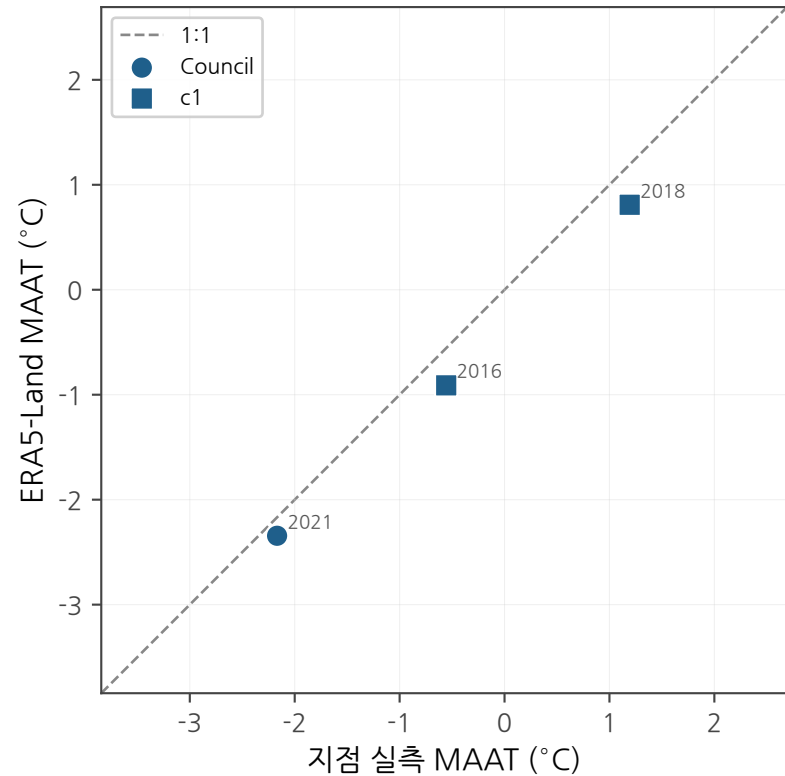
연평균 기온 (bias -0.30°C)
