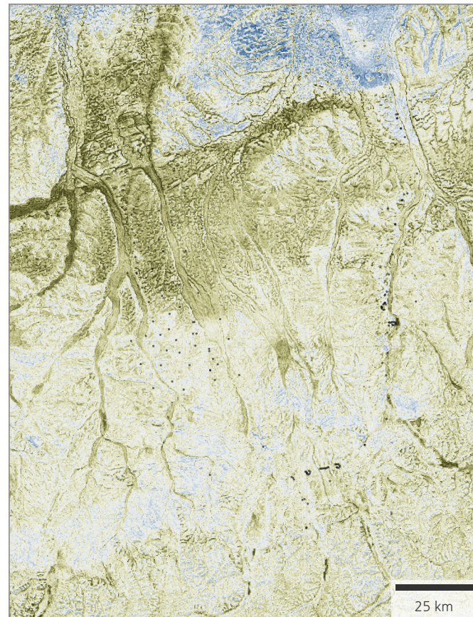
(c) 지형 기여, (b) - (a)
