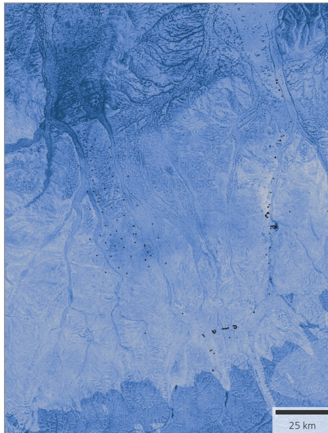
(b) 30 m 지형 공변량 추가, 격자 243 m
