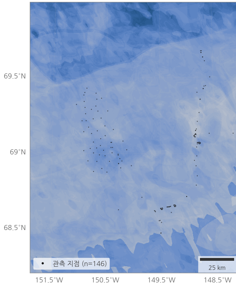
(a) 기후(11 km)·토양(5 km) 공변량만
