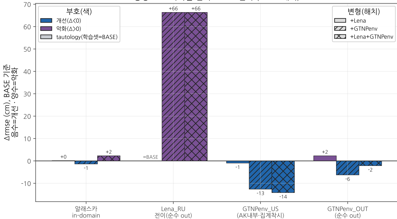
증강 소스·지역별 전이 RMSE 변화 (BASE 대비)
