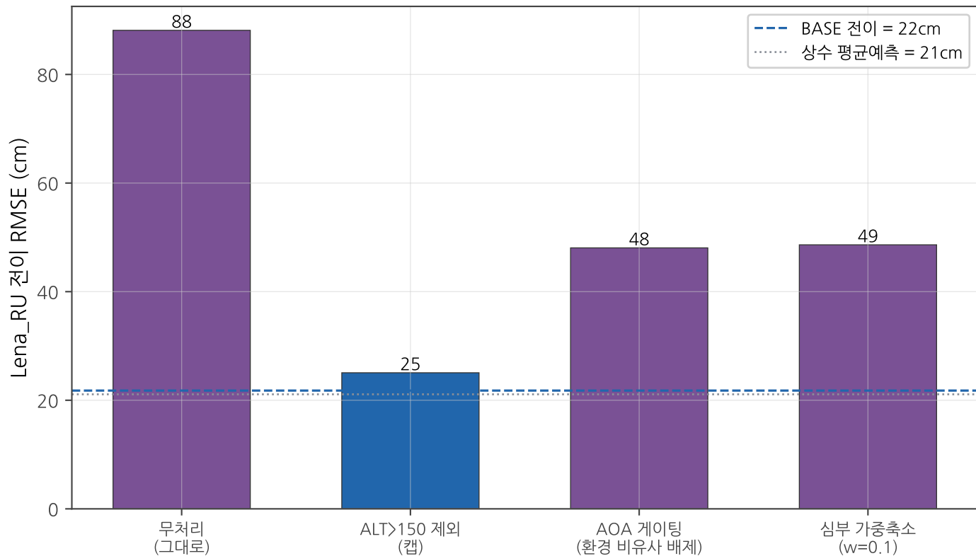
심부 라벨 처리별 전이: 캡(ALT>150 제외)만 회복, 게이팅·가중은 실패
