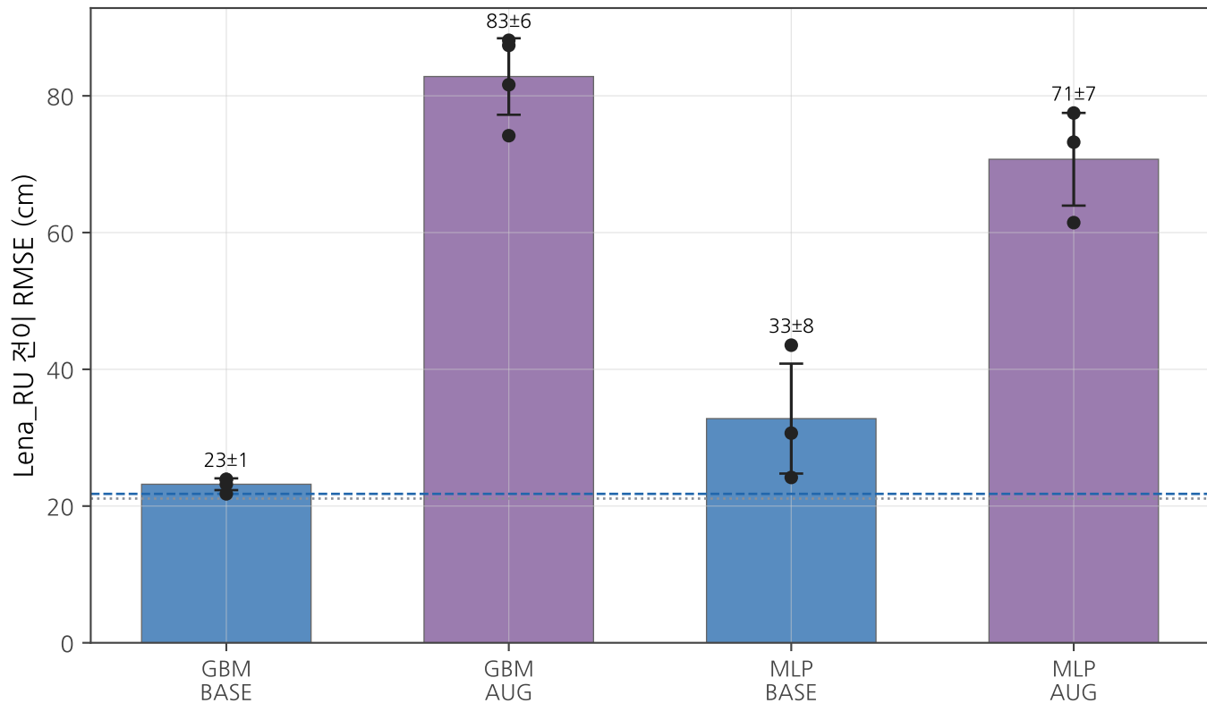
seed 견고성: GBM 붕괴는 견고, MLP BASE는 seed 변동 큼
