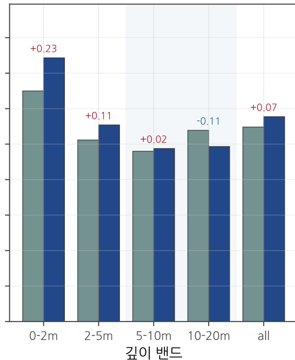
공간블록6 (0.5°분리)
