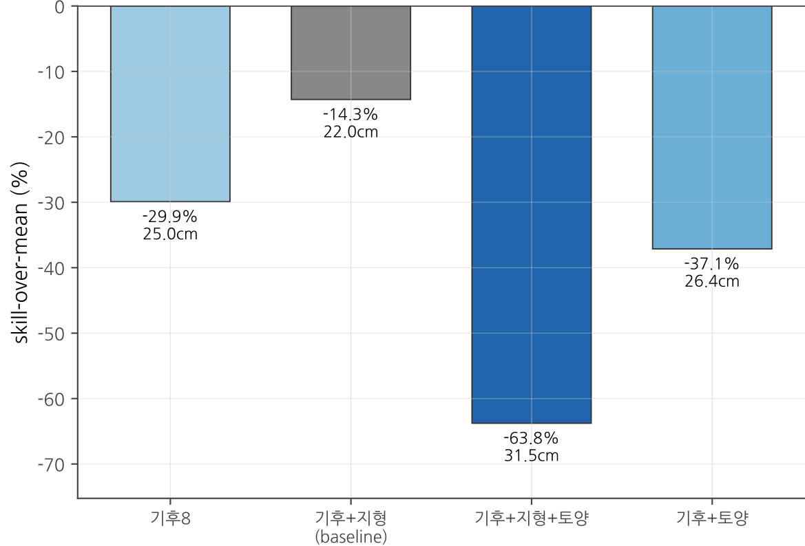
LORO (지역 전이)
