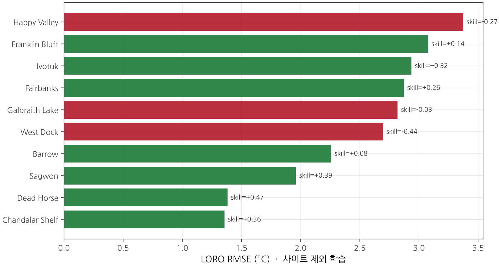
사이트별 전이(LORO) 필드 성능 · 녹색=평균예측 우세, 적색=열세
