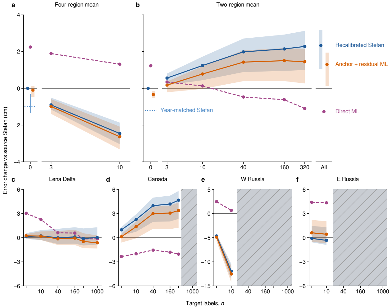
그림 2. 라벨 10 개에서 Stefan 재보정은 4 지역 평균 오차를 낮추었고, 잔차 ML의 추가 차이는 확인하지 못했다. 오차 변화는 학습에서 뺀 각 지역의 채점 블록에서 한 방법의 평균 제공된 오차 (RMSE)에서 원천 계수 Stefan 식 (0 선)의 RMSE를 뺀 값이며, 음수는 오차가 낮다는 뜻이다. Recalibrated Stefan은 대상 라벨 n 개로 계수 E 를 다시 맞추되 원천 계수 쪽으로 수축하고 ( \kappa = 10 ), Anchor + residual ML은 가중 0.25의 CatBoost 잔차를 더하며, Direct ML은 물리 앵커 없는 CatBoost이고, Year-matched Stefan은 라벨 연도의 용해도를 쓴다. (a) 주 4 지역 (레나델타, 캐나다, 러시아 서부, 러시아 동부) 평균, 라벨 10 개까지. (b) 후보 라벨이 40 개 이상인 레나델타와 캐나다의 평균. All은 모든 라벨이며, Year-matched Stefan은 점 추정이다. (c-f) 지역별. 후보 풀보다 큰 라벨 수 (러시아 서부·동부 14–17 셀, 캐나다 325–406 셀)는 가렸고, 패널 e는 세로 범위가 따로다 (–12.5 cm 까지). 선은 분할 5 개의 셀 가중 평균이고, 띠는 재보정 기반 두 방법의 95% 블록 부트스트랩 신뢰구간 (CI)이다 (패널 a, b의 구성 고정 평균은 재표집 10,000 회, 패널 c–f는 1000 회). 라벨 10 개에서 재보정은 4 지역 RMSE를 2.5 cm 낮추었고 (95% CI [1.9, 3.0] cm, Holm 보정 P = 0.001 ), 오차가 낮아진 곳은 러시아 서부뿐이었으며 (12.0 cm, 95% CI [10.5, 13.6] cm), 캐나다에서는 오차가 높아졌다 (2.3 cm, 95% CI [0.7, 2.9] cm). 잔차를 더하면 RMSE가 –0.18 cm 달라졌다 (95% CI [–0.53, –0.01] cm, 보정 전 P = 0.034 , Holm 보정 P = 0.136 ). 그림 모든 대비의 판정은 보충 표 S1에 있다. 라벨 격자 분석은 내부 사전 등록하였고 한 계산 플랫폼에서 실행하였다.
