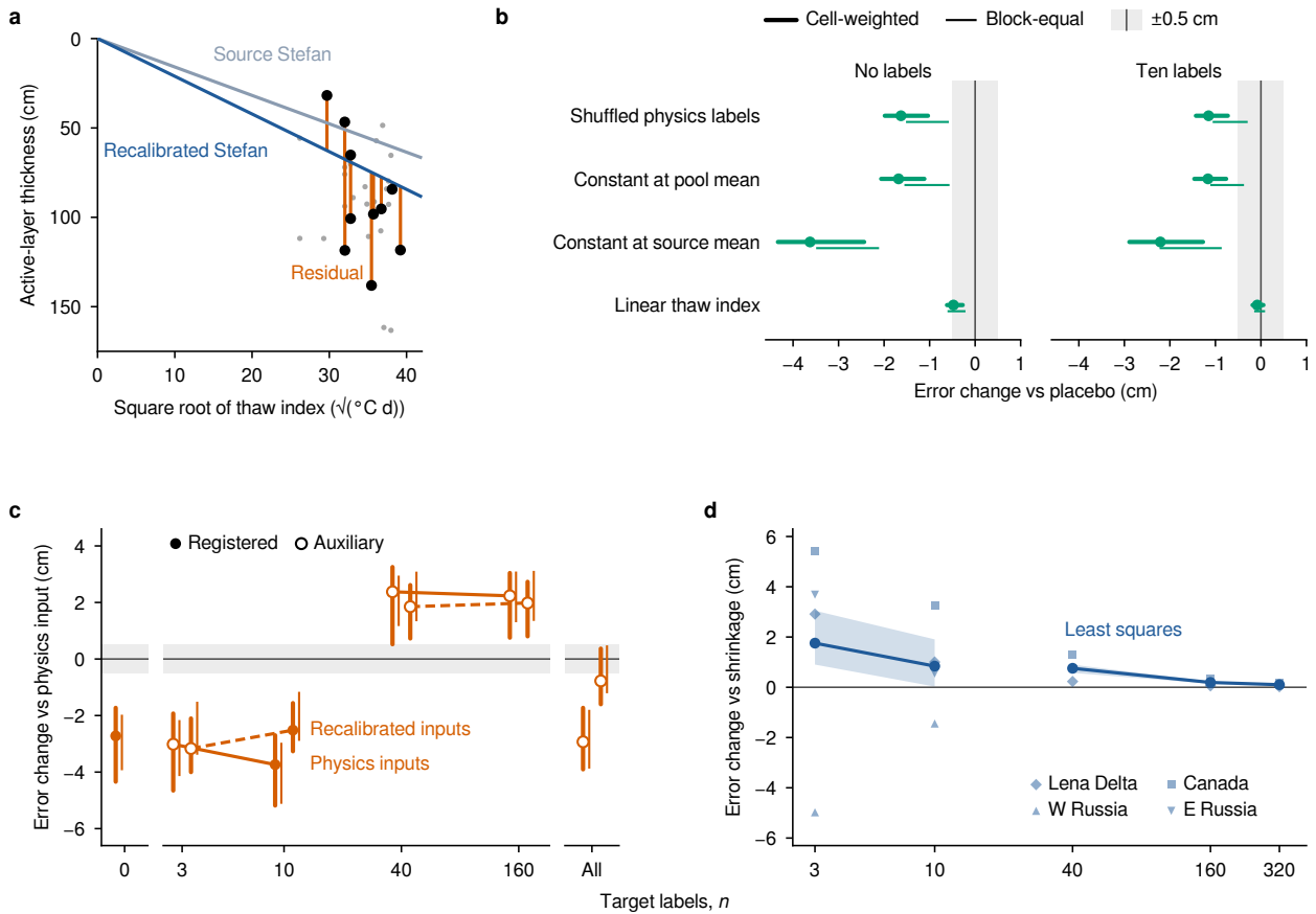
그림 3. 물리 유사라벨은 섞은 유사라벨보다 오차를 낮추었고, 더 나은 결합 구조는 라벨 수에 따라 달랐다. (a) 러시아 서부 라벨 셀 31 개로 그린 개념도. 용해 도일 제공근에 대한 활동층 두께와, 원천 계수 Stefan 직선 (Source Stefan, 1.59 \text{ cm } (^{\circ}\text{C d})^{-1/2} ), 뽑은 라벨 10 개로 재보정한 직선 (Recalibrated Stefan, 2.11), 잔차 ML 이 학습하는 그 라벨들의 편차 (Residual) 를 보인다. 두께는 아래로 갈수록 커진다. (b) 물리 유사라벨로 학습한 직접 ML 에서 위약 유사라벨로 학습한 같은 모델을 뺀 값, 4 지역 평균, 라벨 0 개와 10 개. (c) 잔차 구조에서 물리 입력 구조를 뺀 값을 라벨 수에 대해 그렸다. 입력 집합은 두 가지다 (Physics inputs 는 두 물리 모델의 출력, Recalibrated inputs 는 원천 계수와 재보정 Stefan 예측). 범례는 등록 라벨 수 (0 과 10) 와 보조 라벨 수를 구분하며, 라벨 40 개와 160 개의 값은 레나델타와 캐나다의 평균이다. (d) Stefan 계수의 현지 최소제곱 재보정에서 수축 재보정을 뺀 값 (서술; 양수는 수축이 유리), 라벨 10 개까지는 4 지역 평균, 그 위는 레나델타와 캐나다 평균. 구간은 95% 블록 부트스트랩 신뢰구간 (CI; 0.5^{\circ} 채점 블록 재표집 10,000 회) 이며, 범례에 표시한 대로 셀 가중과 블록 등가중이다 (패널 d 는 셀 가중). 회색 띠는 \pm 0.5 \text{ cm} 다. 패널 b 에서 물리 유사라벨은 섞은 유사라벨보다 라벨 0 개의 오차를 1.6 cm 낮추었고 (95% CI [1.0, 2.0] cm, Holm 보정 P = 0.001 ), 선형 용해 지수 유사라벨과의 차이는 라벨 0 개에서 0.48 cm, 라벨 10 개에서 \pm 0.5 \text{ cm} 안이었다. 패널 c 에서 라벨 10 개까지 잔차 구조의 오차는 두 가중 모두에서 2.5–3.7 cm 낮았고 (라벨 10 개의 물리 입력력에서 Holm 보정 P = 0.001 ), 라벨 40 개와 160 개에서는 물리 입력 구조의 오차가 1.9–2.4 cm 낮았으며 이 차이는 캐나다에서 왔다 (대비 4 개 가운데 1 개는 분할 독립 가정에 의존). 위약과 결합 구조 분석은 내부 사전 등록하였다.
