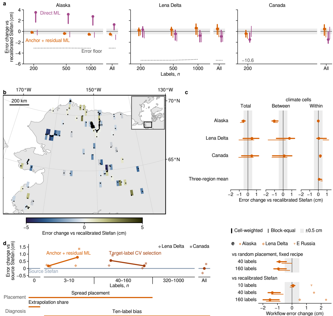
그림 6. 알래스카 안에서 재보정 Stefan 식에 대한 잔차 ML의 이득은 1 cm 미만이었고, 기후 격자 규모의 편향 보정에서 왔다. (a) 지역 내 시험 (0.5° 블록의 절반을 채점, 분할 25 개). 같은 라벨로 재보정한 Stefan 식 대비 Anchor + residual ML(교차검증 잔차 가중) 과 Direct ML의 오차 변화. Error floor는 공변량 조건부 하한(알래스카 11.31 cm, 레나델타 14.83 cm, 캐나다 17.90 cm)에서 재보정 Stefan RMSE를 뺀 값이며, 캐나다 선(-10.6 cm부터 -10.8 cm까지)은 축 아래에 있다. 알래스카의 라벨 1000개에서 잔차 모델은 오차가 0.54 cm 낮았다. 라벨 500개와 전량의 감소(0.39 cm와 0.52 cm)는 공통 재표집 구간에서 유지되지 않았다. 레나델타와 캐나다에서는 차이를 확인하지 못했다. (b) 알래스카, 라벨 전량. 채점 블록별 오차 변화(분할 25개 합산)와 라벨 위치 343 곳. 채점 셀이 10개 미만인 블록은 가렸다. (c) ERA5-Land 기후 셀 사이와 안으로 나눈 오차 변화. 알래스카에서 오차 제공 감소의 약 99%는 셀 사이 성분에서 왔고(-1.03 cm; 셀 안 -0.01 cm), 3 지역 평균에서는 셀 안 예측이 오차를 0.09 cm 키웠다. (d) 라벨 구간별 권장 방법. 원천 계수 Stefan 식 대비 오차 변화, 레나델타와 캐나다 전이 풀(점 추정 2 지역 평균; 라벨 320개와 1000개는 시험하지 않음). 아래에는 배치와 진단 단계를 적었다. 라벨 40개부터의 선정은 고정 레시피에 대한 비열등에 근거한다(그림 5c). (e) 같은 지역을 다시 무작위로 나눈 분할에서 워크플로(d; 배치는 무작위 추출로 바뀜)를 무작위 배치와 고정 레시피(-0.86 cm, -0.93 cm; 라벨 40개, 160개), 재보정 Stefan 식(+0.08 cm, -1.35 cm, -1.51 cm; 라벨 10개, 40개, 160개)과 비교하였다. 기호는 재보정 Stefan 식보다 0.5 cm 넘게 나쁜 지역이다. 앞선 결과를 본 뒤 설계, 재사용 지역의 재검정, 비맹검 부분 포함. 구간은 95% 블록 부트스트랩 신뢰구간(CI; 0.5° 채점 블록 재표집 10,000 회)이며, 셀 가중과 블록 등가중이다(범례). \pm 0.5 cm 띠는 동등 한계다. 패널 a-d는 전이 결과를 본 뒤 설계하였다. 알래스카 중심의 평가 투영, 축적 막대는 70° N 기준. 해안선은 Natural Earth 50 m, Cartopy 0.23.0.
