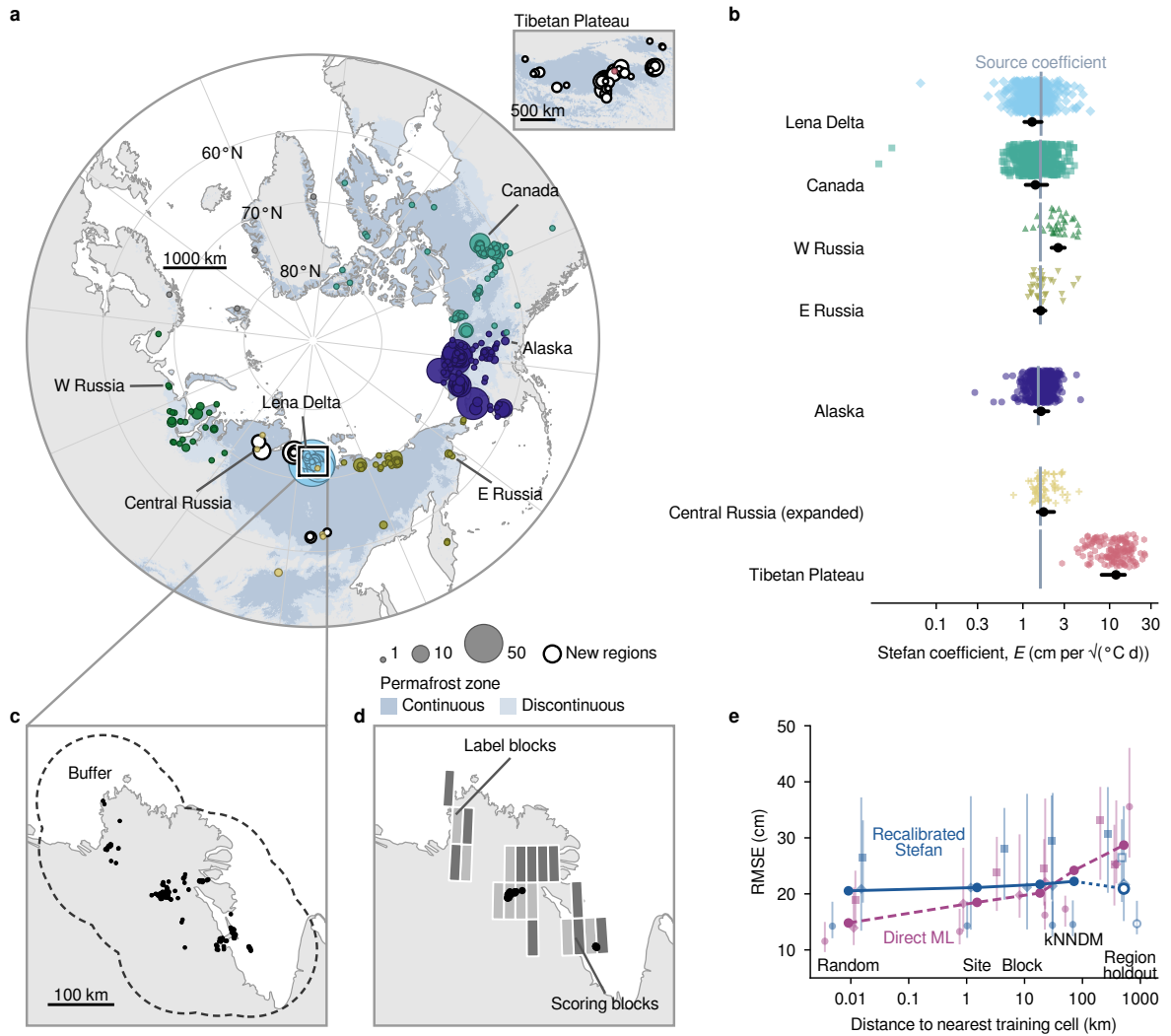
그림 1. 연구 지역, Stefan 계수, 평가 설계. (a) 약관이 확인된 라벨 표의 라벨 셀을 0.5° 블록으로 모았다. 원의 면적은 블록 안 1 km 라벨 위치 수에 비례하고, 색은 b와 같이 지역을 나타내며 (회색은 그린란드, 스발바르, 스칸디나비아), New regions는 라벨 표를 고정한 뒤 더한 지역이다 (러시아 중부 확충판; 티베트 고원은 삽도; 표 1). 음영은 연속 영구동토 (영구동토 비율 \geq 90\% )와 불연속 영구동토 (50–90%)다 (ESA CCI Permafrost fraction v4.0, 1997–2021년 평균). 사각형은 c와 d의 범위다. (b) 지역별 라벨 셀의 Stefan 계수 E = ALT/\sqrt{TDD} (로그 축). ALT는 활동층 두께, TDD는 ERA5-Land 6 기온 융해 지수다 ( ^{\circ}\text{C d} , 2015–2020년 평균). 지역마다 최대 400 셀과 중앙값, 사분위 범위를 보이며, Source coefficient는 그 지역을 학습에서 뺐을 때 원천 풀에서 맞춘 계수다. (c) 지역 홀드아웃. 레나 델타의 라벨 셀과 그로부터 100 km 안의 모든 셀 (Buffer)을 학습 자료에서 뺐다. (d) 같은 지역을 라벨 블록과 채점 블록으로 나눈 분할 (5개 가운데 하나)과 라벨 블록에서 뽑은 라벨 셀 40개. 오차는 채점 블록에서만 잔다. 지역 내 시험은 원천 자료 없이 같은 블록 분할을 쓰며, 전이 결과를 본 뒤 설계하였다. (e) 무작위 셀부터 지역 홀드아웃까지의 검증에서 RMSE를 채점 셀에서 가장 가까운 학습 셀까지의 거리 중앙값에 대해 그렸다 (선은 3 지역 평균, 기호는 셀 가중 95% 구간을 붙인 지역 값, 속이 빈 기호는 원천 계수 Stefan). 무작위 셀 분할에서 kNNNDM 분할로 가면 직접 ML의 RMSE는 5.76 cm, 8.17 cm, 14.20 cm, 재조정 Stefan의 RMSE는 0.29 cm, 0.51 cm, 4.28 cm 늘었다 (알래스카, 레나델타, 캐나다; 셀 가중; 서술, 앞선 결과를 본 뒤 설계). 약관이 확인되지 않은 셀 (캐나다 38, 북대서양 19, 러시아 서부 1)은 그리지 않았다. 북극 평사 투영 (중심 경도 127^{\circ}\text{E} ), 축척 막대는 70^{\circ}\text{N} 기준이며, c와 d도 같은 투영이다. 티베트 고원 삽도는 Lambert 방위 정적 투영이고 축척 막대가 따로 있다. 해안선은 Natural Earth 50 m (c와 d는 10 m), Cartopy 0.23.
