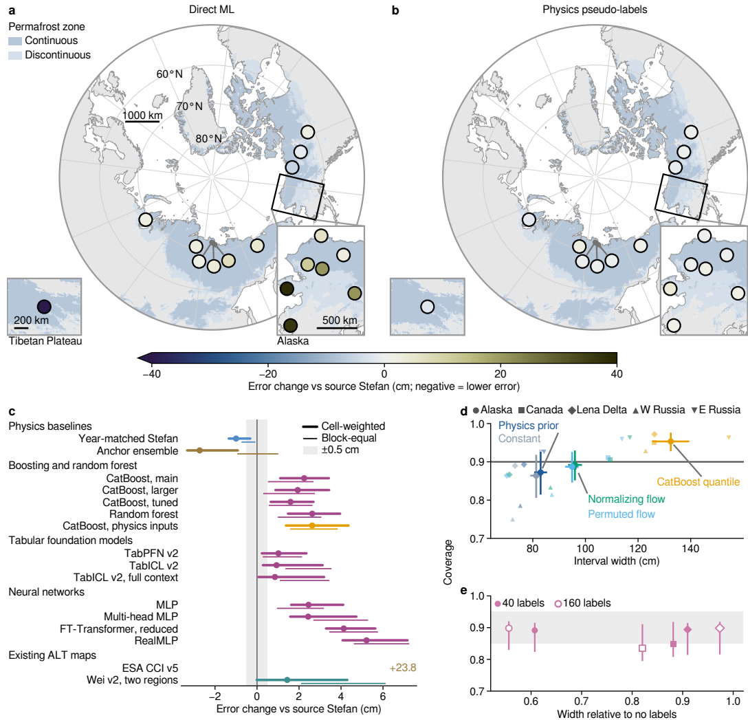
그림 4. 대상 라벨이 없을 때 2 cm 넘게 손해를 본 대상은 30 개 가운데 물리 유사라벨에서 2 개, 직접 ML 에서 18 개였다. (a, b) 각 대상의 라벨 셀 중심에서 직접 ML(a) 과 물리 유사라벨을 쓴 직접 ML(b) 의 원천 계수 Stefan 식 대비 오차 변화 (대상 17 개; 원천에서 상위 지역을 뺌). -40 cm 보다 작은 값은 끝 색으로 칠한다 (a 의 티베트 고원, -60.0 cm). 알래스카 대상은 확대하였고, 레나델타 대상은 지시선으로 옮겨 그렸다. 제목의 개수는 대상 30 개에 대한 사후 집계다 (지역 안 하위 지역과 라벨 확충판 3 개를 더함; 점 추정 문턱). (c) 학습기별 직접 ML 과 두 물리 기준선, 4 지역 평균. 랜덤 포레스트, 물리 모델 입력을 받는 CatBoost, 원천 지역 하나 제외 교차검증으로 설정한 신경망 4 종은 오차가 높았다 (2.4–5.2 cm). 주 CatBoost 학습기 (2.2 cm, 95% CI [1.1, 3.4] cm, Holm 보정 P = 0.023 ) 를 포함한 나머지 학습기 5 종도 주 구간에서 오차가 높았고, 이는 분할 독립 가정에 의존한다. Year-matched Stefan 은 오차가 1.0 cm 낮았고, 이것도 같은 가정에 의존한다. Anchor ensemble 은 척도 보정 Stefan, Kudryavtsev, ESA CCI 앵커의 평균이다. 기존 ALT 지도 (등록 이탈; 앞선 결과를 본 뒤 설계; 제품 학습 지점 5 km 블록 제거): CCI v5 는 오차가 높았고 (+23.79 cm, 축 끝에 표시, 95% CI [15.34, 30.16]), Wei v2(레나델타와 캐나다; 결측 대체 47.4%) 는 차이를 확인하지 못했다. (d) 라벨이 없을 때 구간 척도 다섯 가지에서 90% 예측 구간의 포함률을 평균 폭에 대해 그렸다. 4 지역 평균 (95% 부트스트랩 구간, 재표집 1000 회) 과 지역 값이며, 겹쳐 적은 이름은 거의 같은 두 평균이고 위쪽이 포함률이 높다. 선은 명목 0.90 이다. (e) 라벨 40 개와 160 개에서 잔차 모델 구간의 포함률을 라벨 0 개 대비 폭에 대해 그렸다. 띠는 0.85–0.95 다. c 와 e 의 구간은 95% 블록 부트스트랩 신뢰구간 (0.5° 채점 블록 재표집 10,000 회) 이며, c 는 셀 가중과 블록 등가중이다 (범례). ±0.5 cm 띠는 동등 한계다. 북극 평사 투영 (중심 경도 127° E; 알래스카 확대도 157° W), 축척 막대는 70° N 기준. 티베트 고원 삽도는 Lambert 방위 정적 투영. 영구동토 구역은 ESA CCI Permafrost fraction v4.0(1997–2021 년 평균), 해안선은 Natural Earth 50 m, Cartopy 0.23.0.
