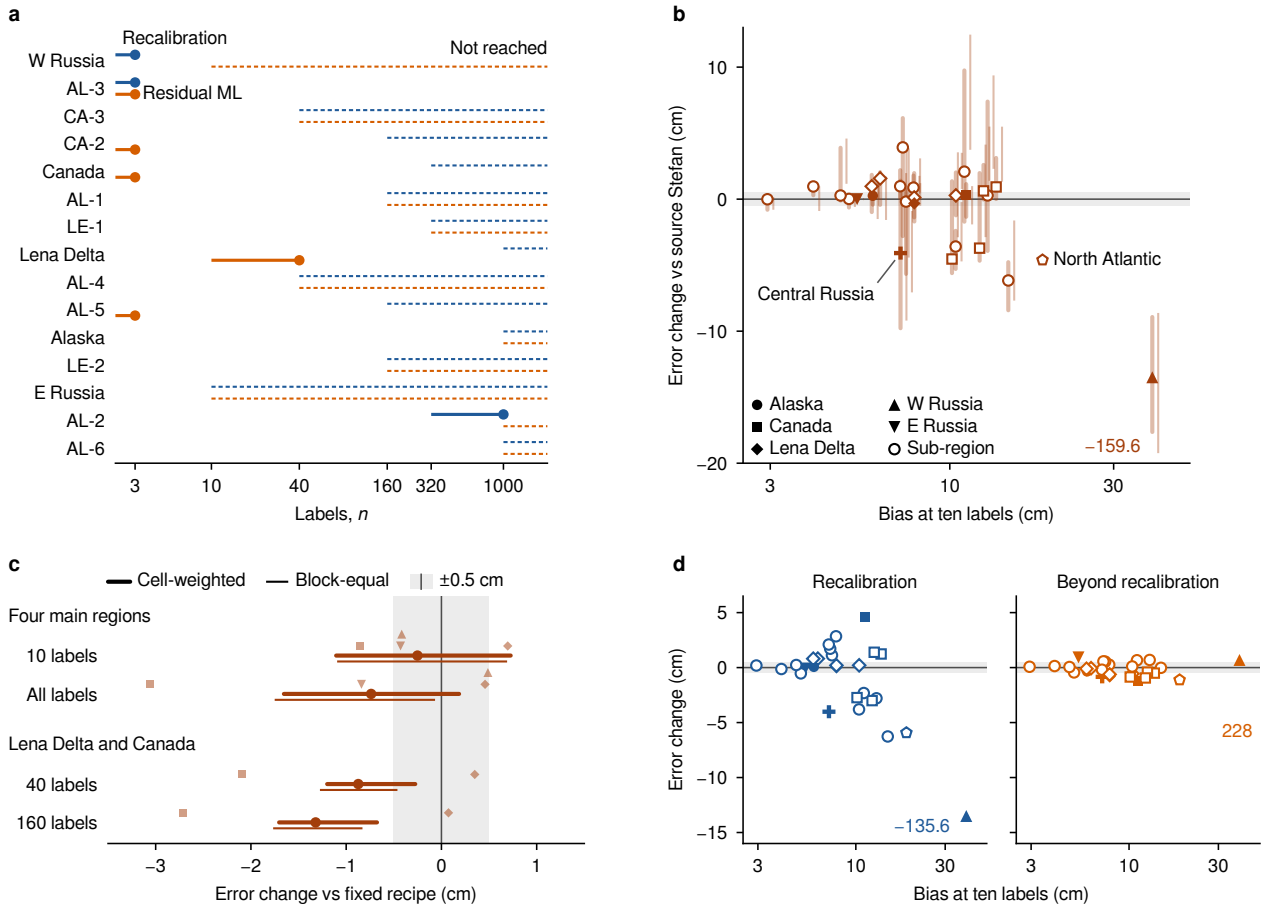
그림 5. 라벨을 쓰는 보정의 오차 감소는 라벨 10 개로 갯 원천 계수 편향과 순위상관을 보였다. (a) 재보정이 원천 계수 Stefan 식보다 오차를 낮춘 (Recalibration) 시험 라벨 수의 최솟값 n^* 와, 잔차 ML 이 재보정 모델보다 오차를 낮춘 (Residual ML) n^* (앞 격자 값부터의 구간). 판정은 등록된 세 조건을 따른다 (방법). Not reached 는 시험한 가장 큰 라벨 수까지 n^* 가 없는 대상이다. 행은 b 의 라벨 10 개 편향 순서이며, 하위 지역은 독립이 아니다. (b) 대상 라벨 안 교차검증으로 고른 방법의 오차 변화 (라벨 전량, 원천 계수 Stefan 식 기준) 를 처음 라벨 10 개에서 그 모델이 보인 평균 편향의 절댓값에 대해 그렸다 (Spearman \rho = 0.38 , 95% CI [0.17, 0.55], 28 대상; 부호 있는 편향은 \rho = -0.01 ). 티베트 고원은 축 밖에 있으며 (편향 227.7 cm; 오차 변화는 b 에서 -159.6 cm, d 에서 -135.7 cm 와 -5.9 cm), 북대서양은 점 추정이다. (c) 교차검증 선정에서 고정 잔차 레시피 ( \lambda = 0.25 ) 를 뺀 값. 선정은 레나델타와 캐나다 평균의 라벨 40 개와 160 개에서 비열 등이었고 (한계 0.5 cm), 라벨 160 개에서 오차가 1.3 cm 낮았다. 라벨 40 개의 0.87 cm 감소와 라벨 전량의 비열등은 분할 독립 가정에 의존하며, 라벨 10 개에서는 비열등이 성립하지 않았다. 이득은 캐나다에서 왔고 (2.1 cm 와 2.7 cm), 레나델타의 변화는 +0.35 cm 와 +0.07 cm 였다. (d) 라벨 전량에서 재보정의 오차 변화와, 더 나은 재보정 Stefan 식을 넘어선 잔차 ML 의 오차 변화를 같은 편향에 대해 그렸다. 편향과 재보정 오차 감소의 관계 ( \rho = 0.37 , 95% CI [-0.11, 0.93]) 와 재보정을 넘어선 감소의 관계 ( \rho = 0.28 , [-0.19, 0.80]; 대상 고정 구간 [0.18, 0.54]) 는 확인하지 못했다 (사후 분석). 구간은 0.5° 채점 블록 (d 에서는 대상 계열도) 을 10,000 회 재표집한 95% 신뢰구간 (CI) 이며, 범례에 표시한 대로 가중한다. 회색 띠는 \pm 0.5 cm 다. b 와 c 의 분석은 앞선 결과를 본 뒤 설계하였다.
