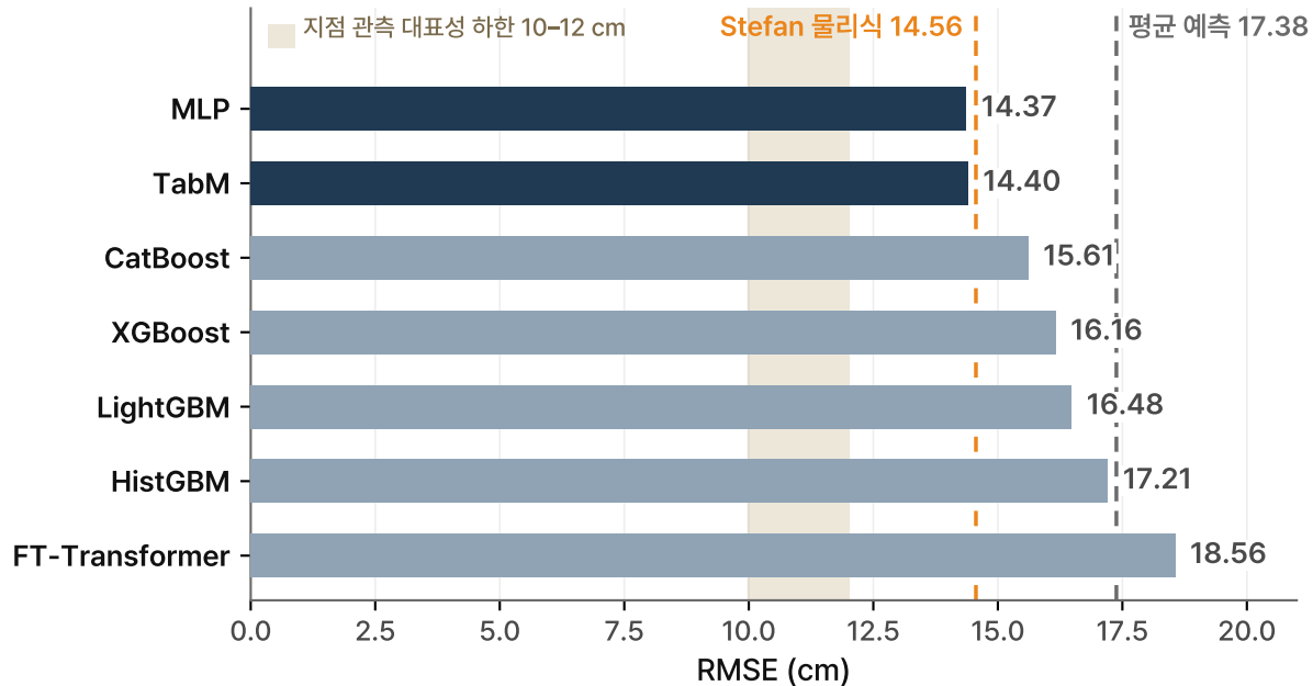
기계학습·딥러닝 7종의 지역 내 예측 오차 (입력 34종, 3-seed 앙상블)
