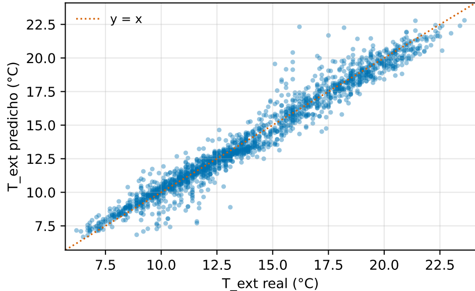
RMSE = 0.81 °C | MAE = 0.57 °C
