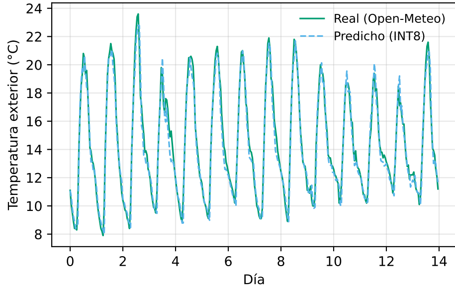
Predicción T_ext a 1 h — 14 días de test (datos reales)
