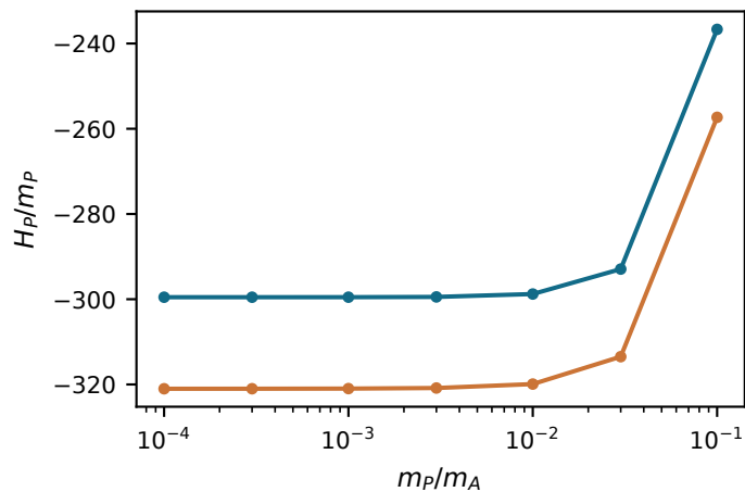
(d) Exact correction at m_P = 0.01
