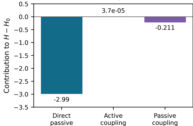
(d) Exact correction at m_P = 0.01
