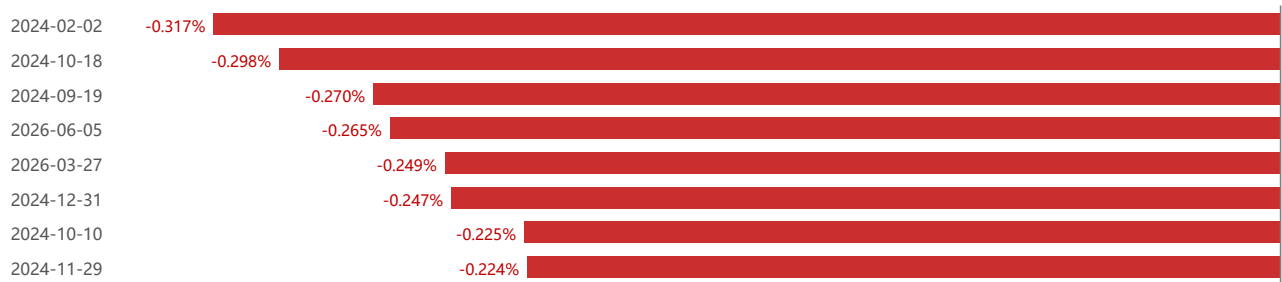
全样本最差的8个交易日
