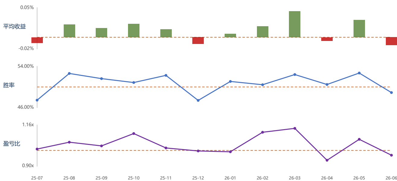
近12个月：收益、胜率和平均盈亏比
