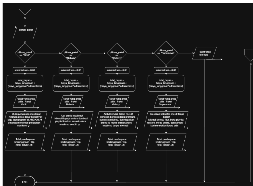
Gambar 1.1 Flowchart bagian 1 dari sistem aplikasi streaming musik “Angkasa”
