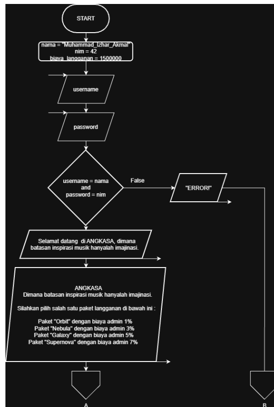
Gambar 1.1 Flowchart bagian 1 dari sistem aplikasi streaming musik “Angkasa”
