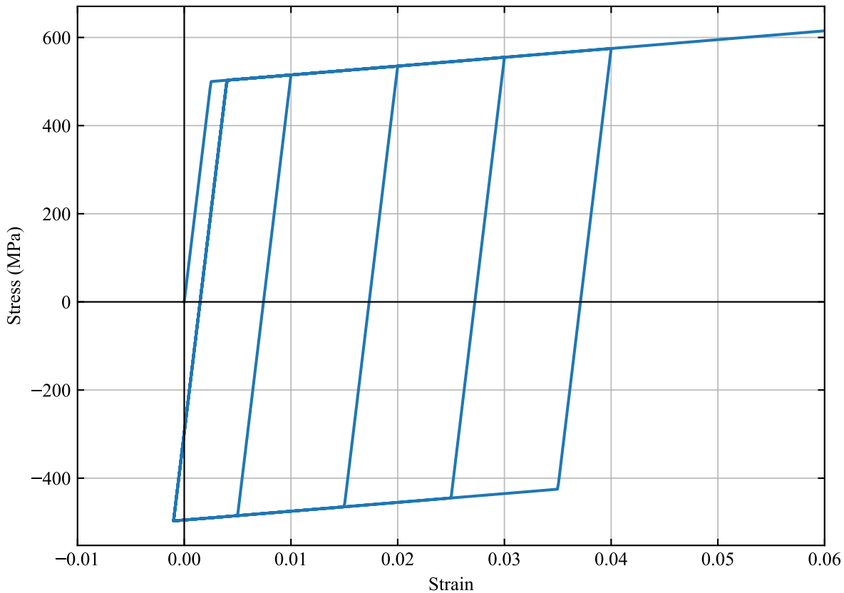
Steel01
