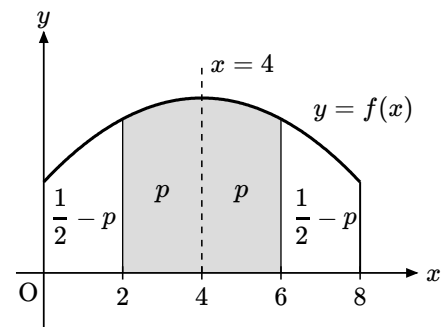
대칭인 그래프의 한 예
