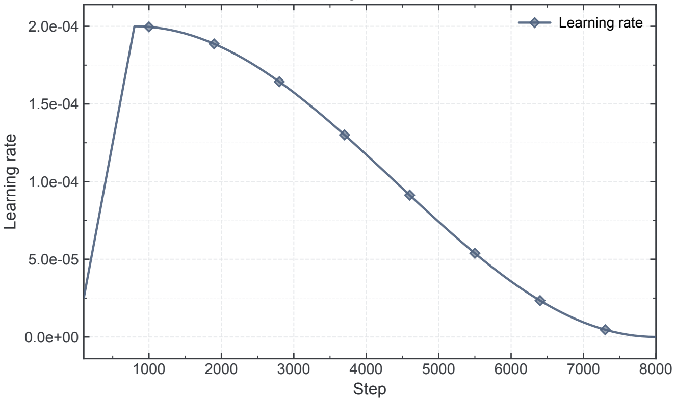
(d) Learning Rate Schedule
