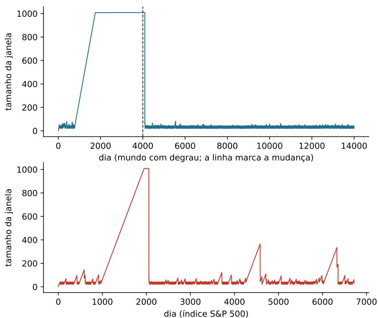
Figura 20.5: O tamanho que o dado escolhe, dia a dia: acima, um mundo com degrau (a linha pontilhada marca a mudança) — a janela despenca do máximo e nunca mais envelhece: oscila rente ao chão declarado; abaixo, o índice real — a janela quase não consegue crescer, e termina colada perto do chão de 21 dias.
