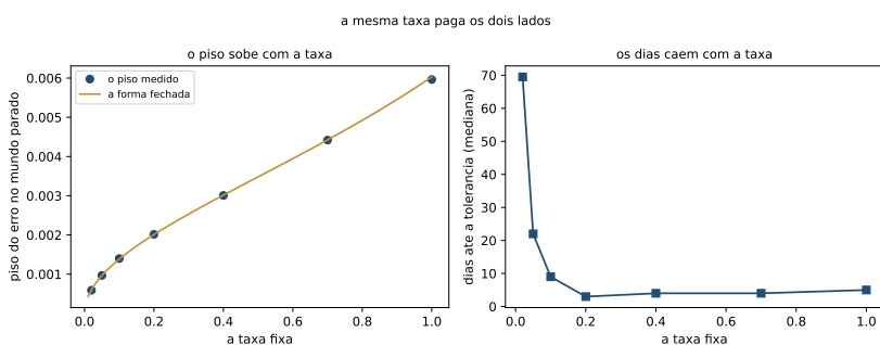
Figura 19.4: À esquerda, o piso medido no mundo parado contra a forma fechada, na grade de taxas; à direita, os dias até a tolerância depois de um degrau. As duas curvas andam em sentidos opostos: o que a taxa compra em dias, ela paga em piso.
