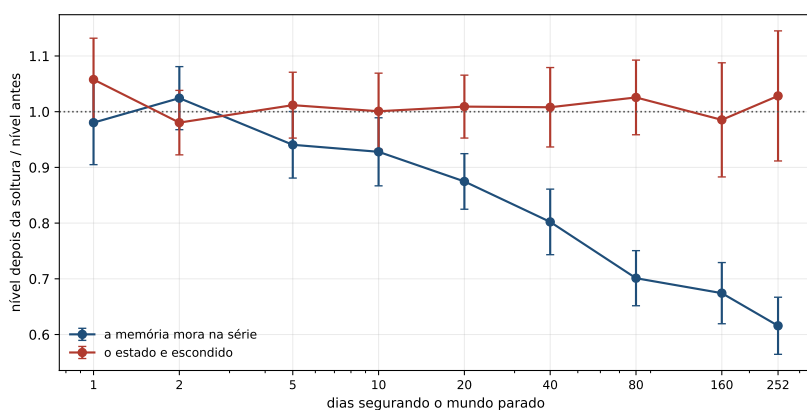
Figura 16.3: A resposta dos dois mundos contra o tempo de contenção, com as barras de dispersão desenhadas sobre 60 replicatas por ponto. A linha pontilhada é a resposta de um mundo que volta ao que era. O eixo horizontal é logarítmico, de modo que a distância entre as últimas marcas vale mais dias do que a figura sugere.
