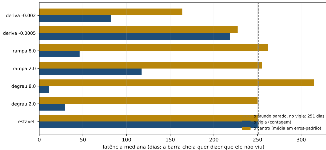
Figure 2.4: A latência mediana de cada instrumento, forma por forma: a contagem de rompimentos contra a média da janela em erros-padrão dela mesma. A linha tracejada é o que o mundo parado produz no primeiro deles, e uma barra que a alcança quer dizer que o instrumento não viu a mudança dentro do horizonte. O que vê a deriva é cego ao degrau, e o que vê o degrau é cego à deriva.
