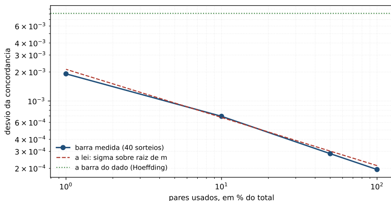
Figura 7.3: A barra do sorteio contra a fração dos pares que se conta, nas duas escalas logarítmicas, com a lei ao lado, e a barra do dado como linha no alto. A linha medida quase coincide com a lei em toda a extensão, e a linha do dado fica acima das duas: o que a economia de pares custa é pequeno diante do que o mercado já cobra.
