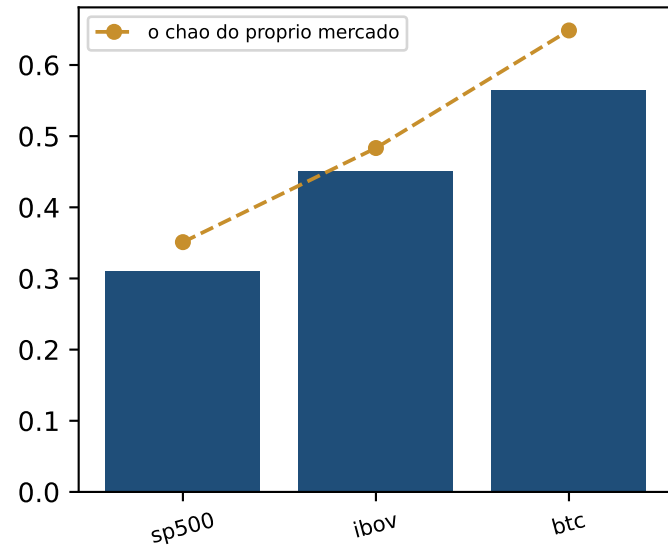
Wasserstein-1
