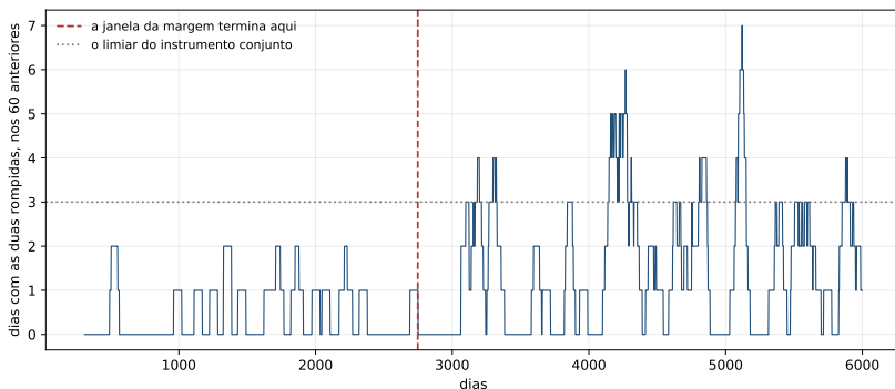
Figura 12.1: A contagem conjunta, dia a dia, com a janela da margem e o limiar do instrumento conjunto. Antes da linha, a série é quase colada no chão; depois, os picos ficam mais altos e mais próximos. A mudança não aparece como degrau: aparece como mais dentes na linha, e quem procura um salto na figura não o encontra.
