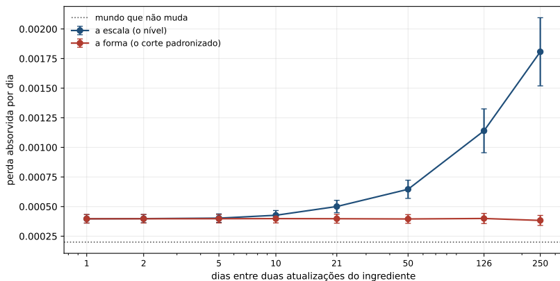
Figura 14.1: A perda absorvida contra o tempo entre duas atualizações, atualizando um ingrediente por vez. O eixo dos tempos é logarítmico, de modo que a distância entre as últimas marcas vale muito mais dias do que a figura sugere. A linha pontilhada é o mesmo desenho num mundo que não muda.
