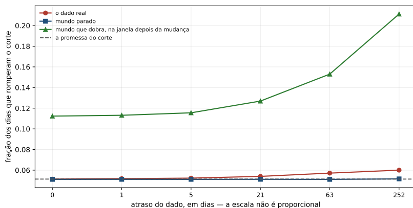
Figura 23.1: A entrega do corte contra a idade do dado, nas três situações: o dado real, o mundo que não muda e a janela que segue uma mudança. As duas de baixo ficam em cima da promessa em qualquer atraso; a de cima é a que segue a mudança.
