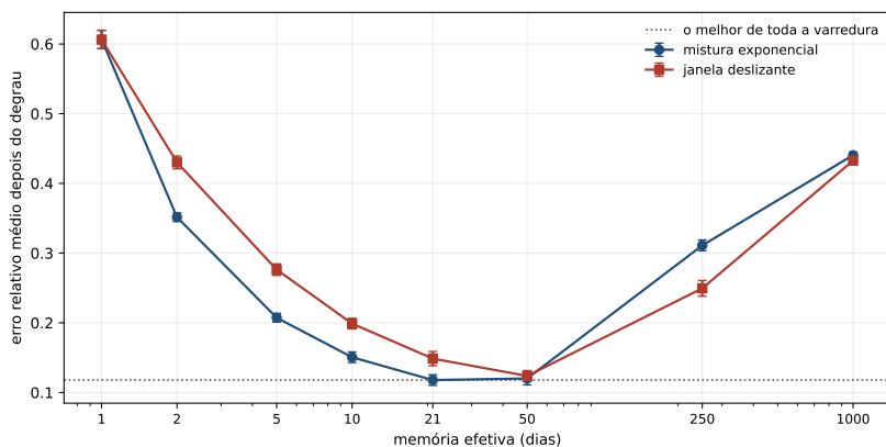
Figura 15.1: O erro depois do degrau contra a memória efetiva, nas duas formas de esquecer. A linha pontilhada é o melhor erro de toda a varredura. O eixo da memória é logarítmico: distâncias iguais no papel são multiplicações iguais no tempo de memória.
