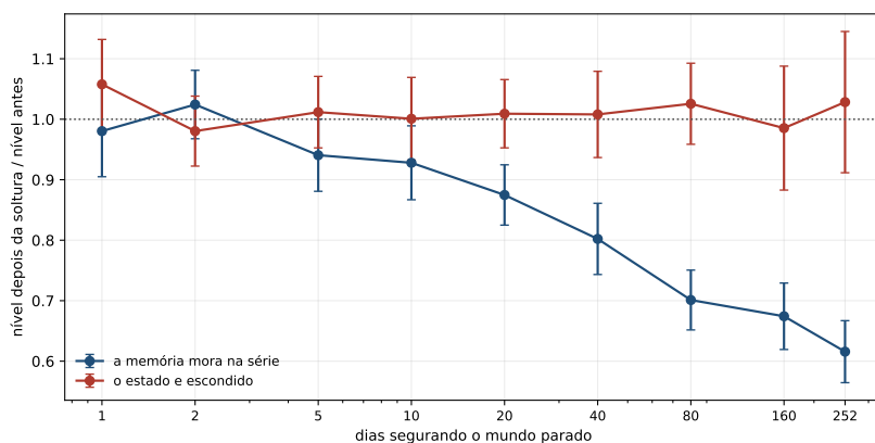
Figura 13.1: A resposta dos dois mundos contra o tempo de contenção, com as barras de dispersão desenhadas sobre 60 replicatas por ponto. A linha pontilhada é a resposta de um mundo que volta ao que era. O eixo horizontal é logarítmico, de modo que a distância entre as últimas marcas vale mais dias do que a figura sugere.
