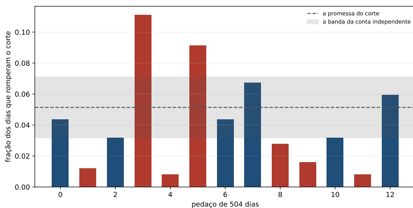
Figura 22.1: A entrega do corte em cada pedaço de 504 dias. A linha tracejada é a conta do corte e a faixa cinza é a banda de quem supõe dias independentes. As barras em vermelho são os pedaços que caem fora da banda.
