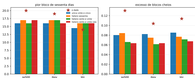
Figura 11.2: A mediana do pior bloco e a do excesso, por configuração e por mercado, com o valor do dado como estrela. As barras são medianas e as estrelas são pontos, sem dispersão desenhada. No painel do pior bloco as faixas de dez a noventa por cento se sobrepõem, de modo que a distância aparente entre barra e estrela é maior do que a distância entre as distribuições.
