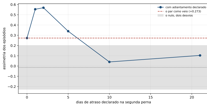
Figura 17.1: A assimetria contra o atraso declarado na segunda perna. A faixa cinza é o nulo a dois desvios sem deslocamento, a linha tracejada é o par como veio, e a curva é o par com o atraso declarado — que o nulo também sofre, e é o que o texto mede.
