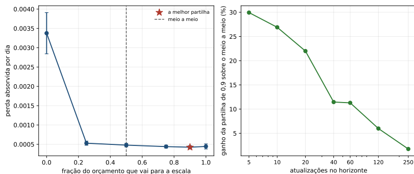
Figura 14.2: À esquerda, a perda contra a fração do orçamento que vai para a escala, com a dispersão entre mundos. O eixo da fração é linear, de modo que os três últimos pontos ficam amontoados à direita. À direita, o ganho da melhor partilha de 0,9 do orçamento para a escala contra o tamanho do orçamento: a vantagem de escolher bem encolhe quando o orçamento engorda.
