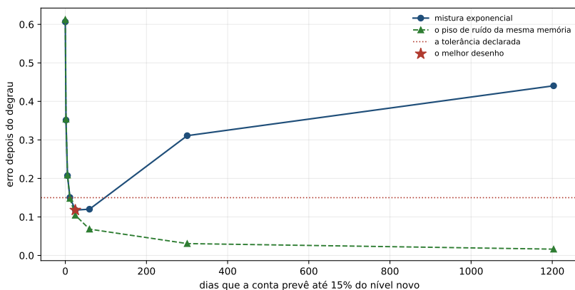
Figura 15.2: O erro depois do degrau contra os dias que a conta do cruzamento prevê até 0,15 do nível novo. A curva tracejada é o piso de ruído da mesma memória: onde ela alcança a curva de cima, o erro deixou de ser atraso e passou a ser tamanho de amostra.
