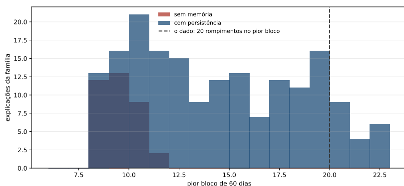
Figura 10.1: Até onde cada família alcança o agrupamento do dado. A linha tracejada é o pior bloco que a série produziu; as barras são quantos membros de cada família chegam a cada valor. O vazio entre as barras da esquerda e a linha parece margem apertada na escala do desenho; é um muro, e não uma folga — e onde as duas famílias caem no mesmo valor, a barra mais alta esconde a outra.
