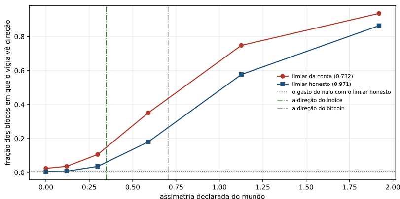
Figura 16.1: O acerto do vigia contra a direção declarada do mundo, nos dois limiares. As linhas verticais marcam a direção medida no índice e no Bitcoin, e a linha pontilhada é o que o vigia gasta à toa com o limiar honesto.
