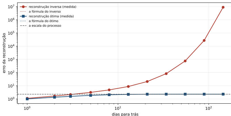
Figura 19.1: O erro das duas reconstruções contra os dias para trás, com a escala do processo como linha de referência. Os pontos são medidos e as linhas pontilhadas são as formas fechadas da proposição 19.1. Os dois eixos são logarítmicos, de modo que a reta do desenho vale uma potência.
