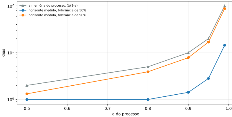
Figura 19.2: A memória do processo e os dois horizontes de recuperação, contra a . São três medidas do mesmo sistema, e cada uma responde a uma pergunta diferente — a curva mais alta é a da memória, e as outras duas são horizontes de recuperação. O eixo dos dias é logarítmico, porque a grandeza só age no fim da escala.
