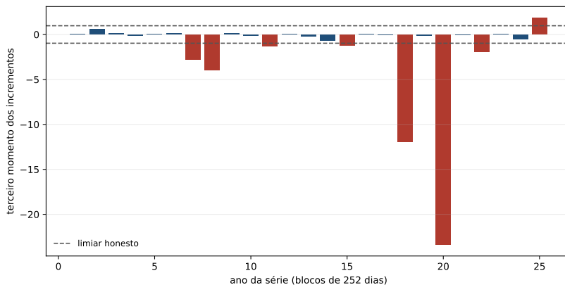
Figura 16.2: O terceiro momento dos incrementos, ano a ano, no índice americano, com o limiar honesto. As barras em vermelho são os anos em que o vigia alarmaria.
