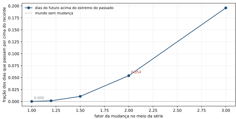
Figura 18.2: A fração dos dias seguintes que passam por cima do recorde de tudo o que veio antes, contra o tamanho da mudança. A linha pontilhada é o mundo que não muda.
