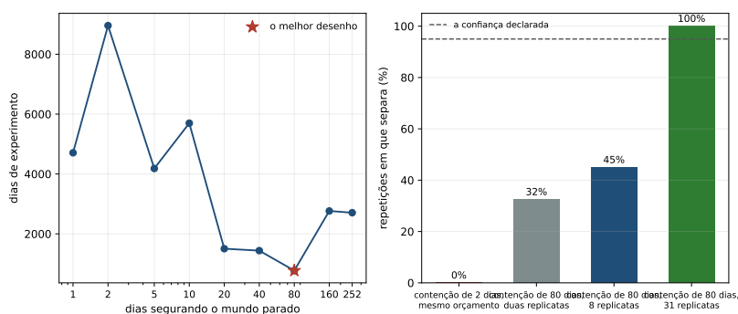
Figura 13.2: À esquerda, o preço do desenho que declara exatamente a diferença medida. À direita, a promessa do desenho verificada por repetição do experimento inteiro: a fração das repetições em que os dois intervalos de fato deixam de se cruzar.
