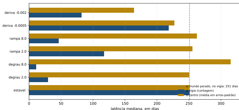
Figura 6.2: A latência mediana de cada instrumento, forma por forma: a contagem de rompimentos contra a média da janela em erros-padrão dela mesma. A linha tracejada é o que o mundo parado produz no primeiro deles, e duas barras que terminam no mesmo lugar merecem cuidado: o mundo parado não é uma forma de mudança, e é ele que reaparece em toda forma.
