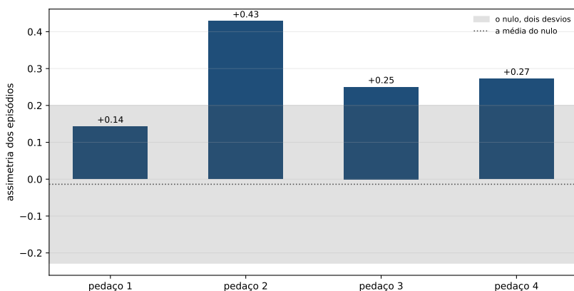
Figura 17.2: A assimetria em cada pedaço do par, contra a faixa do nulo. Os quatro pedaços do par têm 1613, 1613, 1612 e 1612 dias de série, e o primeiro perde a janela inicial, em que o corte ainda não existe.
