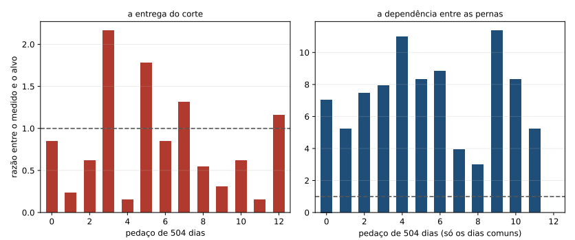
Figura 22.2: As duas conclusões no mesmo tamanho de pedaço, cada uma em razão do seu alvo. À esquerda, a entrega do corte, que atravessa a linha da promessa para os dois lados. À direita, a dependência, que fica sempre bem acima da independência.
