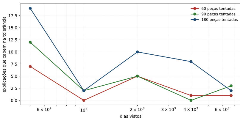
Figura 24.1: As explicações que cabem, contra os dias vistos, uma curva por tamanho de família. O eixo dos dias é logarítmico. A queda é a tendência, e não a regra: entre mil e quatro mil dias as curvas sobem e descem, e no extremo longo a família de 90 peças passa a de 180 — 3 contra 2.
