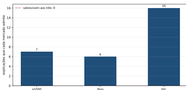
Figura 11.1: Quantas explicações cada mercado admite sozinho, numa varredura, e a linha da interseção. Cada barra é uma varredura só: a do mercado com mais dados vai de 0 a 7 em 10 sementes. A linha colada no eixo é a interseção — nenhuma explicação serve aos três —, e não uma barra que faltou.
