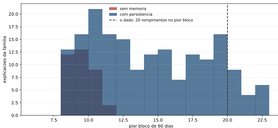
Figure 6.1: Até onde cada família alcança o agrupamento do dado. A linha tracejada é o pior bloco que a série produziu; as barras são quantos membros de cada família chegam a cada valor. A linha colada na borda faz o vazio à esquerda parecer margem apertada; é um muro, e não uma folga.
