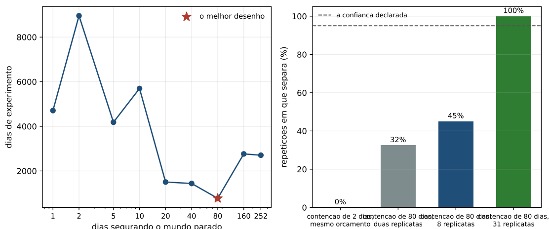
Figure 9.2: À esquerda, o preço do desenho que declara exatamente a diferença medida. À direita, a promessa do desenho verificada por repetição do experimento inteiro: a fração das repetições em que os dois intervalos de fato deixam de se cruzar.
