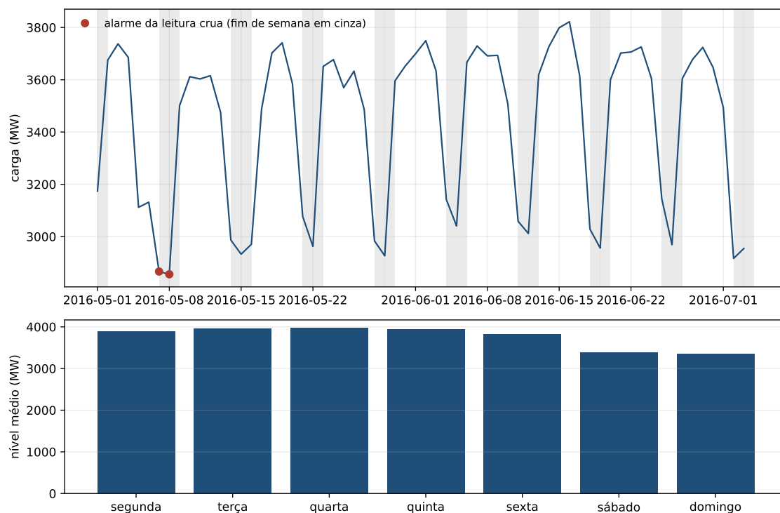
Figura 5.1: Nove semanas de carga dinamarquesa. Os fins de semana estão em cinza, e os dois pontos são os alarmes da leitura crua: os dois caem no cinza. Embaixo, o perfil semanal médio dos cinco anos — o desenho que a leitura crua estava medindo sem saber.
