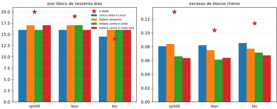
Figura 9.2: A mediana do pior bloco e a do excesso, por configuração e por mercado, com o valor do dado como estrela. As barras são medianas e as estrelas são pontos, sem dispersão desenhada. No painel do pior bloco as faixas de dez a noventa por cento se sobrepõem, de modo que a distância aparente entre barra e estrela é maior do que a distância entre as distribuições.
