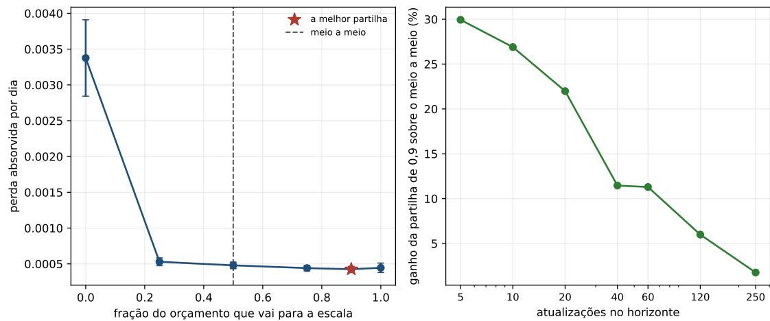
Figura 12.2: À esquerda, a perda contra a fração do orçamento que vai para a escala, com a dispersão entre mundos. O eixo da fração é linear, de modo que os três últimos pontos ficam amontoados à direita. À direita, o ganho da melhor partilha de 0,9 do orçamento para a escala contra o tamanho do orçamento: a vantagem de escolher bem encolhe quando o orçamento engorda.
