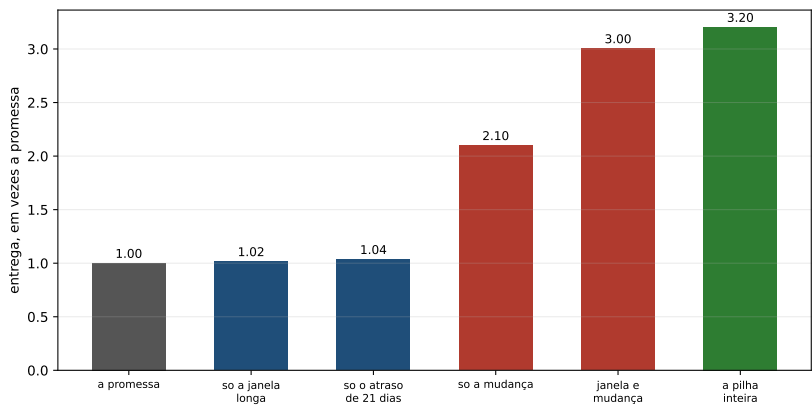
Figura 31.2: A entrega de cada buraco sozinho e a da pilha inteira, em vezes a promessa. A barra verde é a mais alta das seis, e o que essa altura diz é o que o livro inteiro perseguiu: os buracos não se somam, eles se encaixam.
