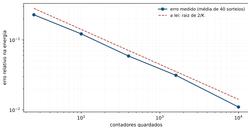
Figura 30.2: O erro do esboço contra o número de contadores guardados, nas duas escalas logarítmicas, com a reta da lei ao lado. As duas linhas são paralelas , e a medida fica abaixo da lei em toda a extensão: a média de uma estimativa simétrica custa cerca de oito décimos do desvio dela, e é isso que a distância entre as duas linhas mede.
