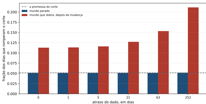
Figura 29.2: O mundo parado e o mundo que dobra, por atraso — o parado medido na série inteira e o que dobra na janela que segue a mudança. A barra azul é o controle: ela fica na promessa em todos os atrasos.
