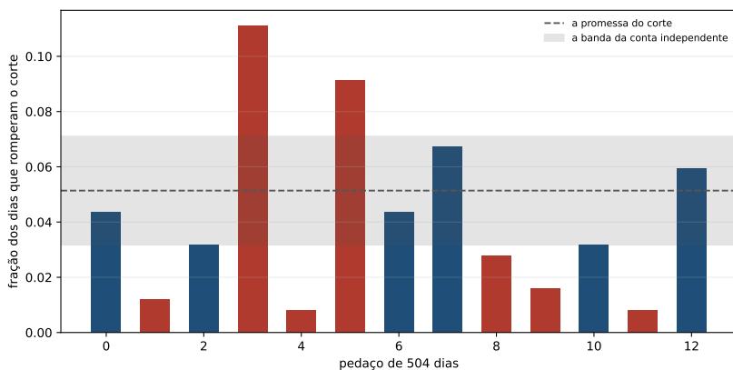
Figura 28.1: A entrega do corte em cada pedaço de 504 dias. A linha tracejada é a conta do corte e a faixa cinza é a banda de quem supõe dias independentes. As barras em vermelho são os pedaços que caem fora da banda.
