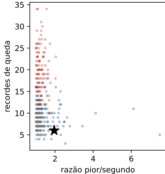
btc
