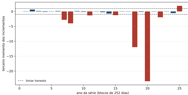
Figura 20.2: O terceiro momento dos incrementos, ano a ano, no índice americano, com o limiar honesto. As barras em vermelho são os anos em que o vigia alarmaria.
