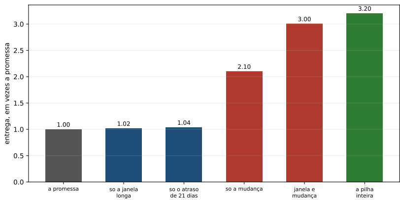
Figura 29.2: A entrega de cada buraco sozinho e a da pilha inteira, em vezes a promessa. A barra verde é a mais alta das seis, e o que essa altura diz é o que o livro inteiro perseguiu: os buracos não se somam, eles se encaixam.
