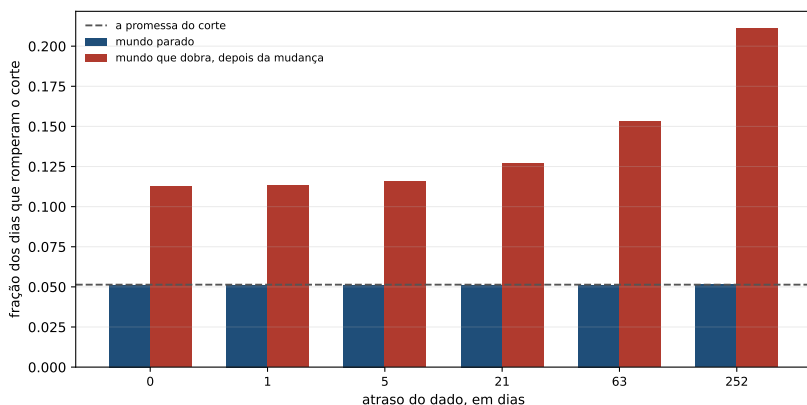
Figura 27.2: O mundo parado e o mundo que dobra, por atraso — o parado medido na série inteira e o que dobra na janela que segue a mudança. A barra azul é o controle: ela fica na promessa em todos os atrasos.
