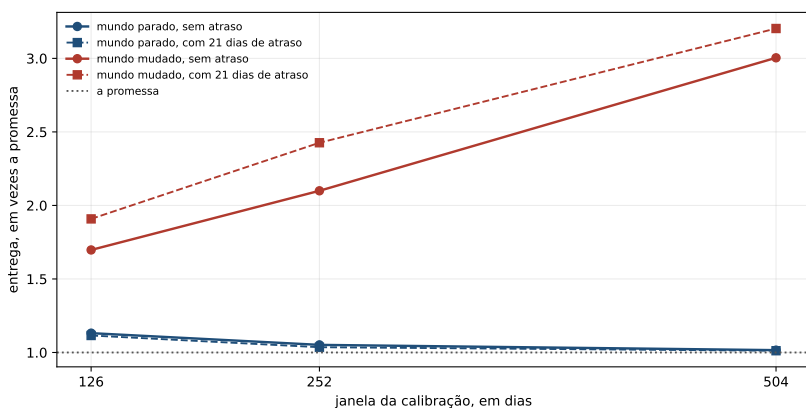
Figura 29.1: A entrega contra a janela da calibração, nos dois mundos e com e sem atraso. As duas curvas do mundo parado descem e as duas do mundo que muda sobem: o mesmo eixo, o sentido trocado.
