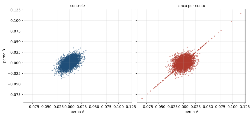
Figura 24.2: A nuvem das duas pernas no mundo gaussiano e no mundo com choque comum. O miolo se abre para que a correlação do conjunto continue a mesma, e o que o segundo tem a mais são dois braços na diagonal, um para cada canto.
