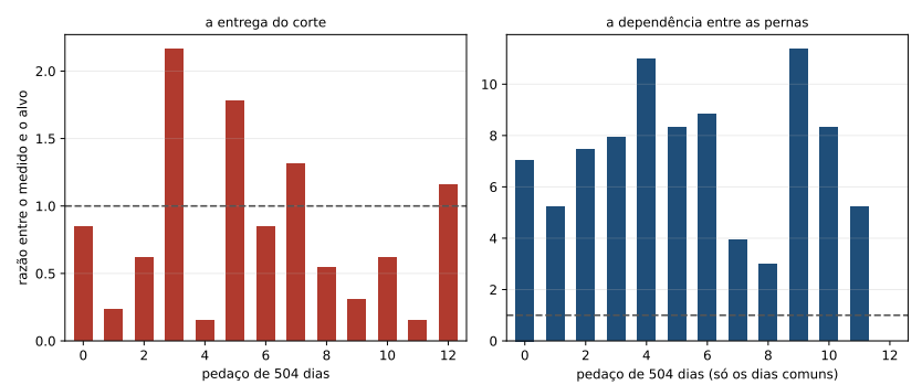
Figura 26.2: As duas conclusões no mesmo tamanho de pedaço, cada uma em razão do seu alvo. À esquerda, a entrega do corte, que atravessa a linha da promessa para os dois lados. À direita, a dependência, que fica sempre bem acima da independência.
