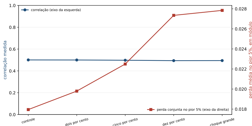
Figura 24.1: A correlação medida e a perda conjunta, contra os cinco mundos. Os dois eixos são diferentes de propósito, e as duas linhas se cruzam no meio do caminho: a reta é a correlação, que anda de 0,4941 a 0,5006, e a que sobe é a perda, que começa abaixo dela e termina acima.
