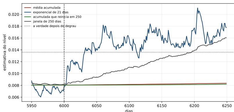
Figura 25.2: Os quatro estimadores em torno do dia do degrau, contra a verdade. Depois dele a exponencial de vinte e um dias reage e oscila em volta da linha; a janela sobe em rampa, porque vai sendo preenchida por dias novos; e a média acumulada e a que reinicia ficam paradas — elas carregam tanto passado que o degrau quase não as move dentro do horizonte da decisão.
