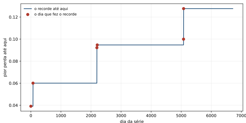
Figura 22.1: A escada do recorde no índice: a pior perda até cada dia, e os dias que ergueram o recorde. São poucos degraus, e cada um deles é um mundo que ainda não tinha sido visto.
