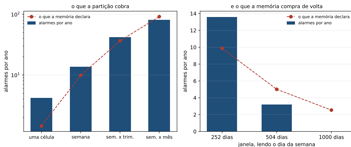
Figura 5.2: À esquerda, o que a partição cobra: alarmes por ano contra o que a memória declara, para as quatro leituras da tabela 5.2. O eixo dos alarmes é logarítmico, de modo que distâncias iguais no papel são multiplicações iguais no preço. À direita, o que a memória compra de volta, com a janela crescendo e a partição semanal fixa.
