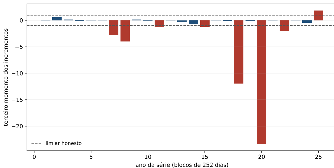
Figura 14.2: O terceiro momento dos incrementos, ano a ano, no índice americano, com o limiar honesto. As barras em vermelho são os anos em que o vigia alarmaria.
