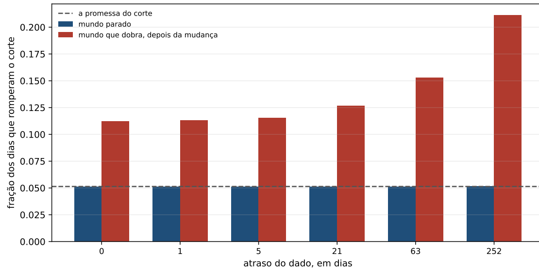
Figura 20.2: O mundo parado e o mundo que dobra, por atraso — o parado medido na série inteira e o que dobra na janela que segue a mudança. A barra azul é o controle: ela fica na promessa em todos os atrasos.
