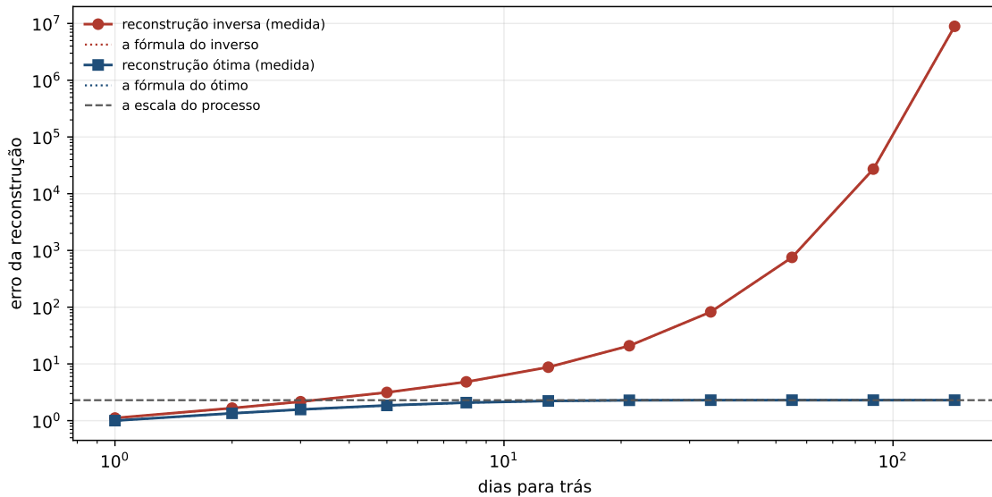
Figura 17.1: O erro das duas reconstruções contra os dias para trás, com a escala do processo como linha de referência. Os pontos são medidos e as linhas pontilhadas são as formas fechadas da proposição 17.1. Os dois eixos são logarítmicos, de modo que a reta do desenho vale uma potência.
