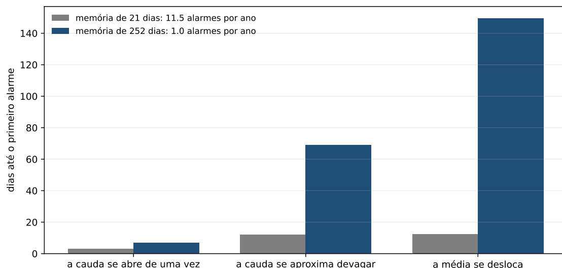
Figura 4.1: Dias até o primeiro alarme, por forma de mudança, em dois orçamentos: a memória de um mês, à esquerda de cada par, e a de um ano, à direita. O orçamento mais raro paga a diferença entre as formas.
