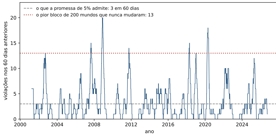
Figura 2.1: Violações nos 60 dias anteriores, dia a dia. A linha tracejada marca o que a promessa de 5% admite; a pontilhada marca o pior bloco que apareceu em 200 mundos que nunca mudam.
