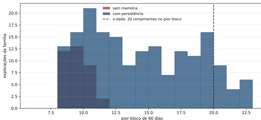
Figura 8.1: Até onde cada família alcança o agrupamento do dado. A linha tracejada é o pior bloco que a série produziu; as barras são quantos membros de cada família chegam a cada valor. O vazio entre as barras da esquerda e a linha parece margem apertada na escala do desenho; é um muro, e não uma folga — e onde as duas famílias caem no mesmo valor, a barra mais alta esconde a outra.
