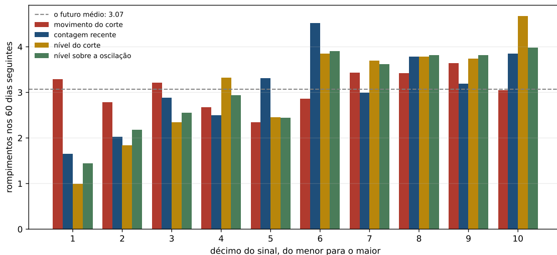
Figura 7.1: O futuro médio em cada décimo dos quatro sinais, com a média geral como linha. Três dos quatro sobem; o do movimento do corte atravessa o gráfico de lado. A leitura é seguir uma cor de ponta a ponta: comparar décimos vizinhos perde a tendência, que é o que a figura mostra.
