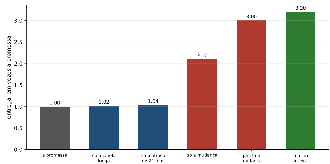
Figura 21.2: A entrega de cada buraco sozinho e a da pilha inteira, em vezes a promessa. A barra verde é a mais alta das seis, e o que essa altura diz é o que o livro inteiro perseguiu: os buracos não se somam, eles se encaixam.
