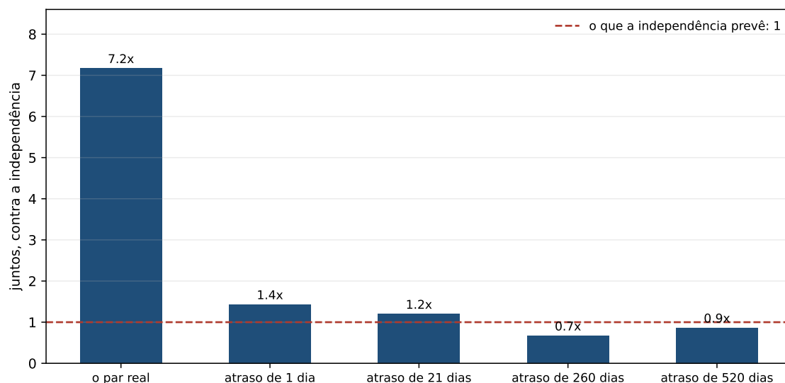
Figura 6.2: A barra da esquerda é o par como o mundo fez; as outras quatro são o mesmo par com o segundo mercado deslocado, e a linha tracejada é o que a independência prevê. Quase toda a dependência morre com um único dia de deslocamento.
