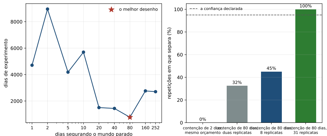
Figura 11.2: À esquerda, o preço do desenho que declara exatamente a diferença medida. À direita, a promessa do desenho verificada por repetição do experimento inteiro: a fração das repetições em que os dois intervalos de fato deixam de se cruzar.
