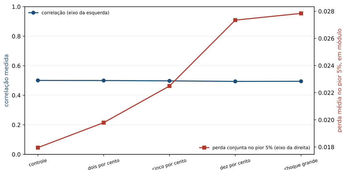
Figura 18.1: A correlação medida e a perda conjunta, contra os cinco mundos. Os dois eixos são diferentes de propósito, e as duas linhas se cruzam no meio do caminho: a reta é a correlação, que anda de 0,4941 a 0,5006, e a que sobe é a perda, que começa abaixo dela e termina acima.
