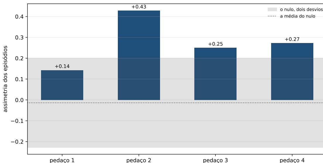
Figura 15.2: A assimetria em cada pedaço do par, contra a faixa do nulo. Os quatro pedaços do par têm 1613, 1613, 1612 e 1612 dias de série, e o primeiro perde a janela inicial, em que o corte ainda não existe.
