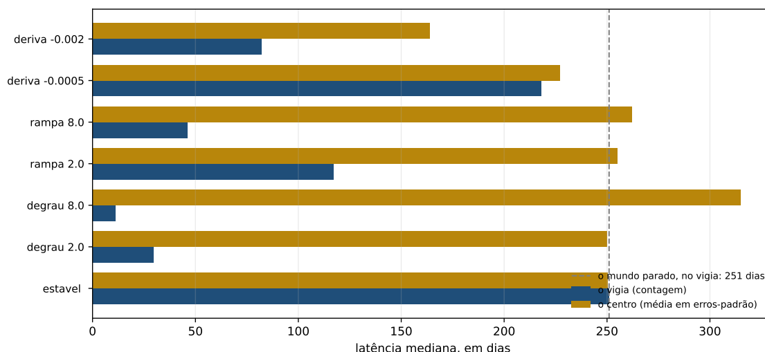
Figura 4.2: A latência mediana de cada instrumento, forma por forma: a contagem de rompimentos contra a média da janela em erros-padrão dela mesma. A linha tracejada é o que o mundo parado produz no primeiro deles, e duas barras que terminam no mesmo lugar merecem cuidado: o mundo parado não é uma forma de mudança, e é ele que reaparece em toda forma.
