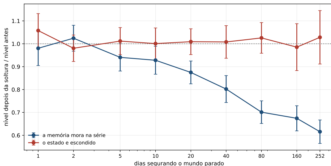
Figura 11.1: A resposta dos dois mundos contra o tempo de contenção, com as barras de dispersão desenhadas sobre 60 replicatas por ponto. A linha pontilhada é a resposta de um mundo que volta ao que era. O eixo horizontal é logarítmico, de modo que a distância entre as últimas marcas vale mais dias do que a figura sugere.
