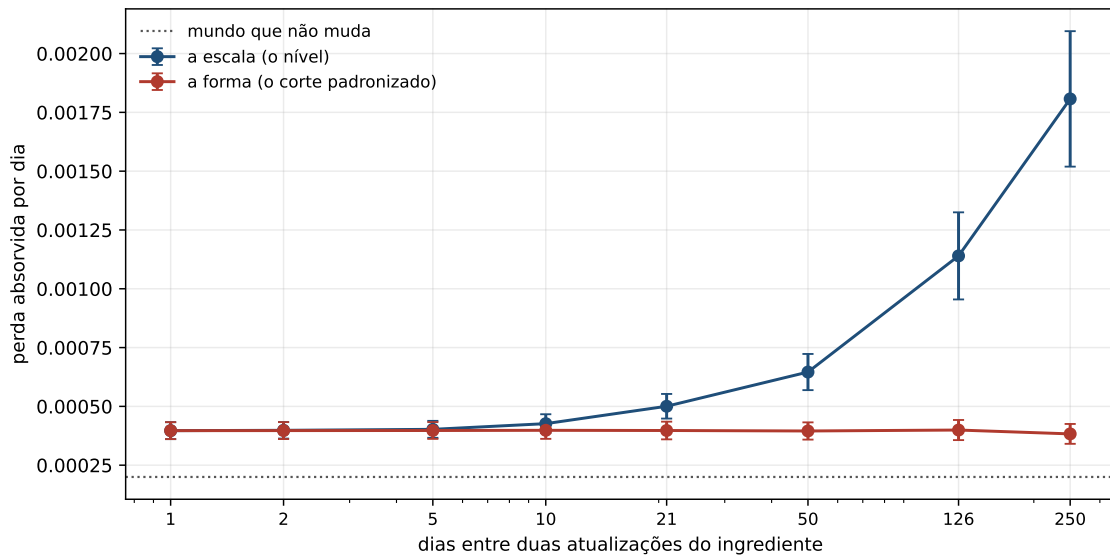
Figura 12.1: A perda absorvida contra o tempo entre duas atualizações, atualizando um ingrediente por vez. O eixo dos tempos é logarítmico, de modo que a distância entre as últimas marcas vale muito mais dias do que a figura sugere. A linha pontilhada é o mesmo desenho num mundo que não muda.
