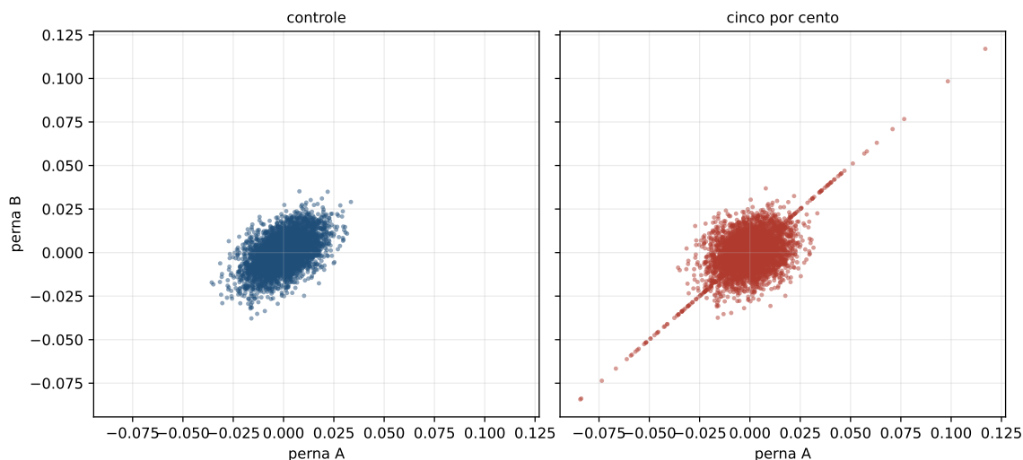
Figura 18.2: A nuvem das duas pernas no mundo gaussiano e no mundo com choque comum. O miolo se abre para que a correlação do conjunto continue a mesma, e o que o segundo tem a mais são dois braços na diagonal, um para cada canto.
