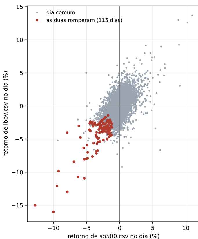
Figura 6.1: Os dois mercados, dia a dia. Cada ponto é um dia, com o retorno de um no eixo horizontal e o do outro no vertical; as linhas em zero partem o plano em quadrantes. Os 115 dias em que as duas pernas romperam estão todos no quadrante de baixo à esquerda, e nenhum em qualquer outro lugar do plano.
