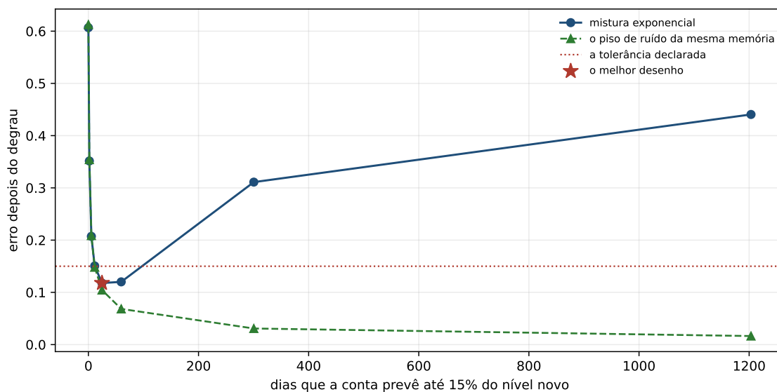
Figura 13.2: O erro depois do degrau contra os dias que a conta do cruzamento prevê até 0,15 do nível novo. A curva tracejada é o piso de ruído da mesma memória: onde ela alcança a curva de cima, o erro deixou de ser atraso e passou a ser tamanho de amostra.
