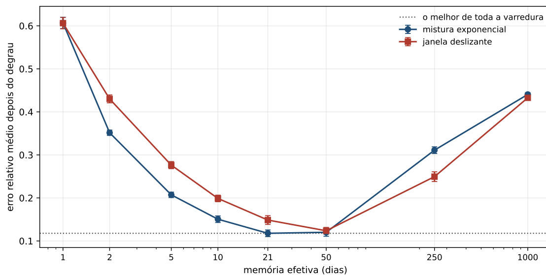
Figura 13.1: O erro depois do degrau contra a memória efetiva, nas duas formas de esquecer. A linha pontilhada é o melhor erro de toda a varredura. O eixo da memória é logarítmico: distâncias iguais no papel são multiplicações iguais no tempo de memória.
