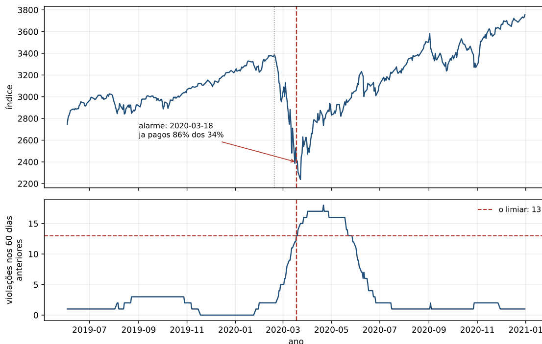
Figura 3.2: O alarme de 18 de março de 2020 visto dos dois lados. Em cima, o índice; embaixo, as violações dos 60 dias anteriores, com o limiar. As duas linhas contam a mesma história — e a de baixo conta depois da de cima.
