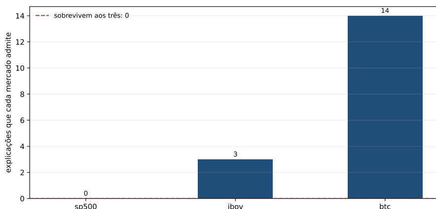
Figura 9.1: Quantas explicações cada mercado admite sozinho, e a linha da interseção. A primeira barra não aparece porque o valor dela é o zero: o mercado com mais dados é o que não admite explicação nenhuma. Barra ausente e barra que faltou têm a mesma cara, e a linha colada no eixo some.
