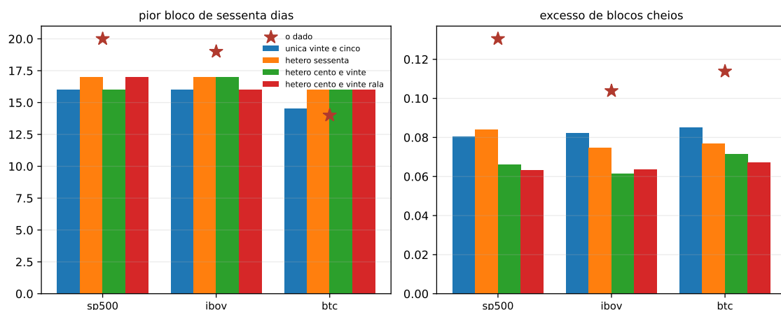
Figura 9.2: A mediana do pior bloco e a do excesso, por configuração e por mercado, com o valor do dado como estrela. As barras são medianas e as estrelas são pontos, sem dispersão desenhada. No painel do pior bloco as faixas de dez a noventa por cento se sobrepõem, de modo que a distância aparente entre barra e estrela é maior do que a distância entre as distribuições.
