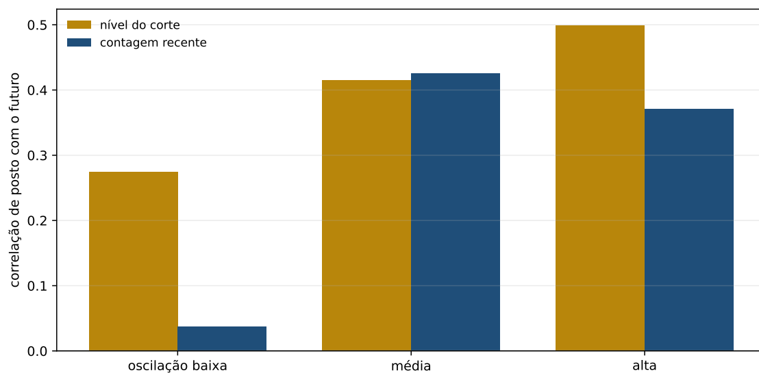
Figura 7.2: O nível do corte e a contagem recente medidos dentro de três faixas de oscilação, onde a oscilação de agora é quase a mesma. O nível não desaparece ao dividir por ela. A barra quase ausente da contagem na faixa calma não é defeito: a contagem é cega justamente onde nada acontece.
