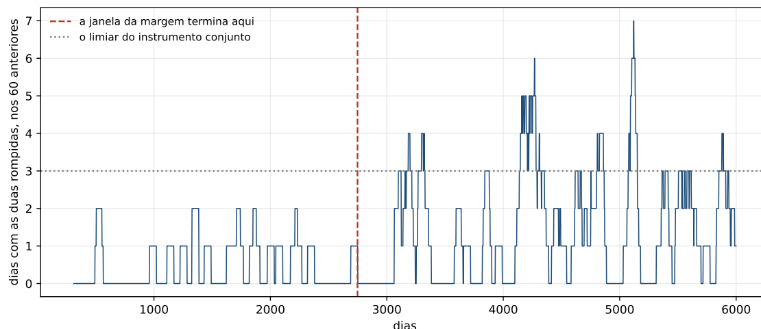
Figura 10.1: A contagem conjunta, dia a dia, com a janela da margem e o limiar do instrumento conjunto. Antes da linha, a série é quase colada no chão; depois, os picos ficam mais altos e mais próximos. A mudança não aparece como degrau: aparece como mais dentes na linha, e quem procura um salto na figura não o encontra.
