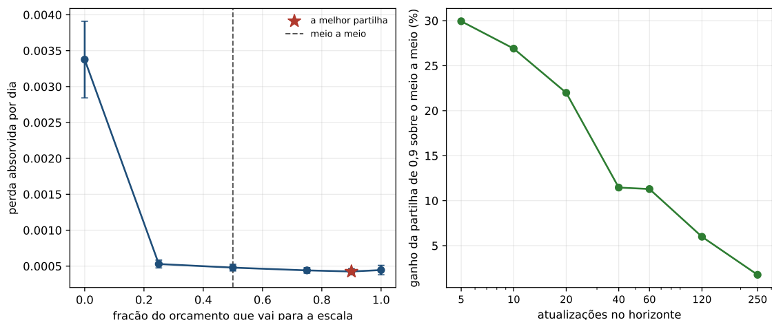
Figura 12.2: À esquerda, a perda contra a fração do orçamento que vai para a escala, com a dispersão entre mundos. O eixo da fração é linear, de modo que os três últimos pontos ficam amontoados à direita. À direita, o ganho da melhor partilha de 0,9 do orçamento para a escala contra o tamanho do orçamento: a vantagem de escolher bem encolhe quando o orçamento engorda.
