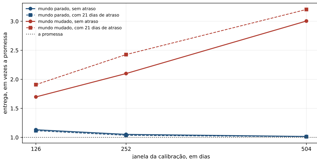
Figura 21.1: A entrega contra a janela da calibração, nos dois mundos e com e sem atraso. As duas curvas do mundo parado descem e as duas do mundo que muda sobem: o mesmo eixo, o sentido trocado.
