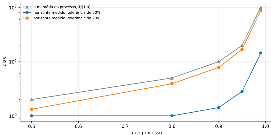
Figura 17.2: A memória do processo e os dois horizontes de recuperação, contra a . São três medidas do mesmo sistema, e cada uma responde a uma pergunta diferente — a curva mais alta é a da memória, e as outras duas são horizontes de recuperação. O eixo dos dias é logarítmico, porque a grandeza só age no fim da escala.
