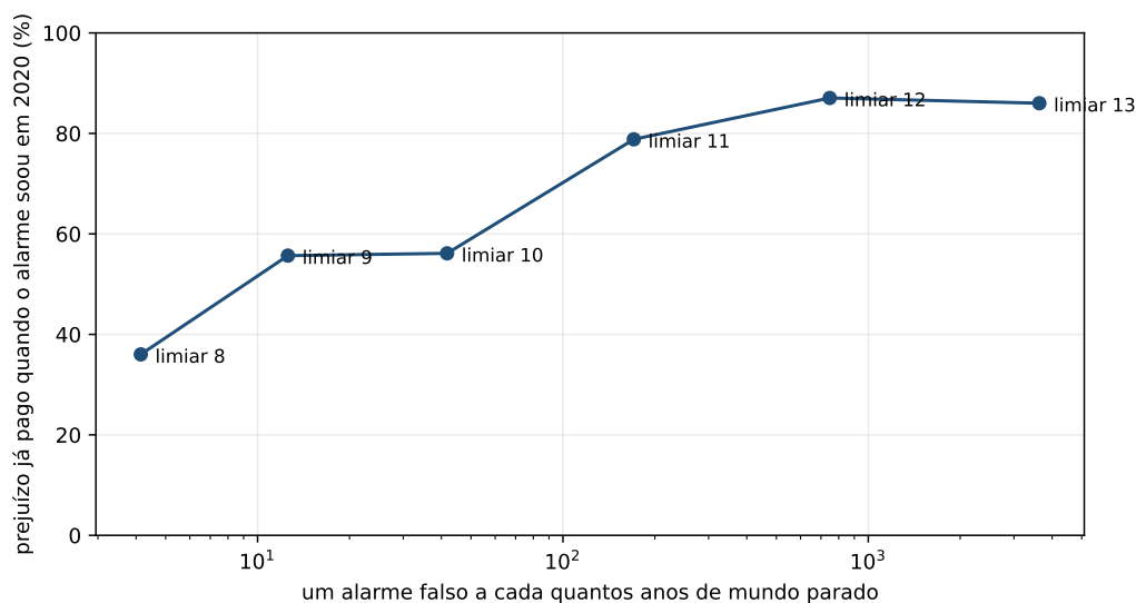
Figura 3.1: A troca em forma de curva: o eixo horizontal é a raridade do falso alarme, em escala logarítmica, e o vertical é o prejuízo já pago no tombo recente. A curva sobe depressa na esquerda e achata na direita.
