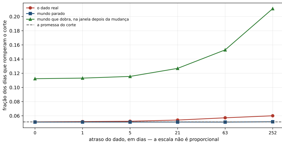
Figura 20.1: A entrega do corte contra a idade do dado, nas três situações: o dado real, o mundo que não muda e a janela que segue uma mudança. As duas de baixo ficam em cima da promessa em qualquer atraso; a de cima é a que segue a mudança.
