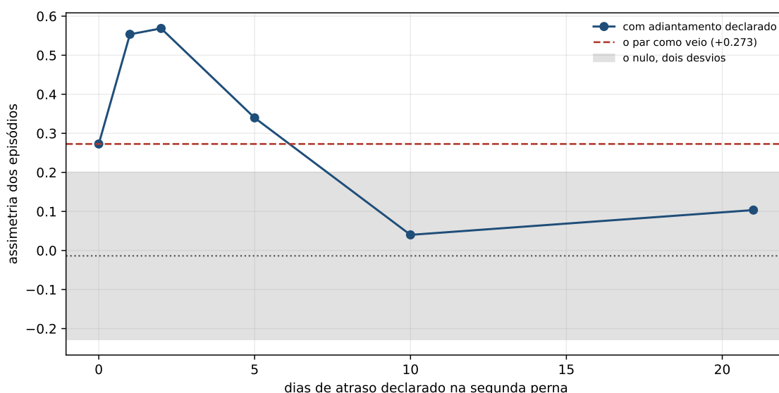
Figura 15.1: A assimetria contra o atraso declarado na segunda perna. A faixa cinza é o nulo a dois desvios, a linha tracejada é o par como veio, e a curva mostra onde o par se alinha melhor.
