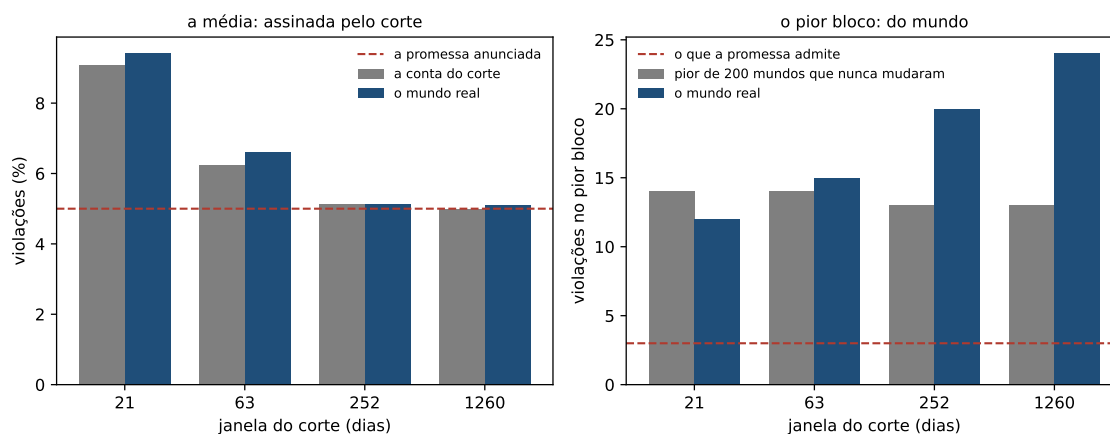
Figura 2.2: As duas leituras, nas quatro janelas. À esquerda, a média: a conta do corte e o mundo real andam juntos. À direita, o pior bloco: o mundo real contra o pior dos 200 mundos que nunca mudam.
