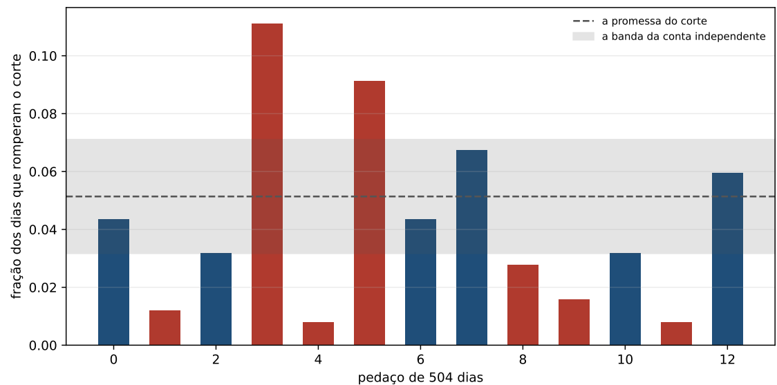
Figura 19.1: A entrega do corte em cada pedaço de 504 dias. A linha tracejada é a conta do corte e a faixa cinza é a banda de quem supõe dias independentes. As barras em vermelho são os pedaços que caem fora da banda.
