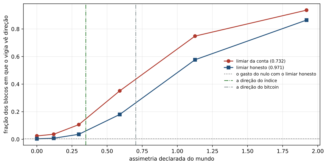
Figura 14.1: O acerto do vigia contra a direção declarada do mundo, nos dois limiares. As linhas verticais marcam a direção medida no índice e no Bitcoin, e a linha pontilhada é o que o vigia gasta à toa com o limiar honesto.
