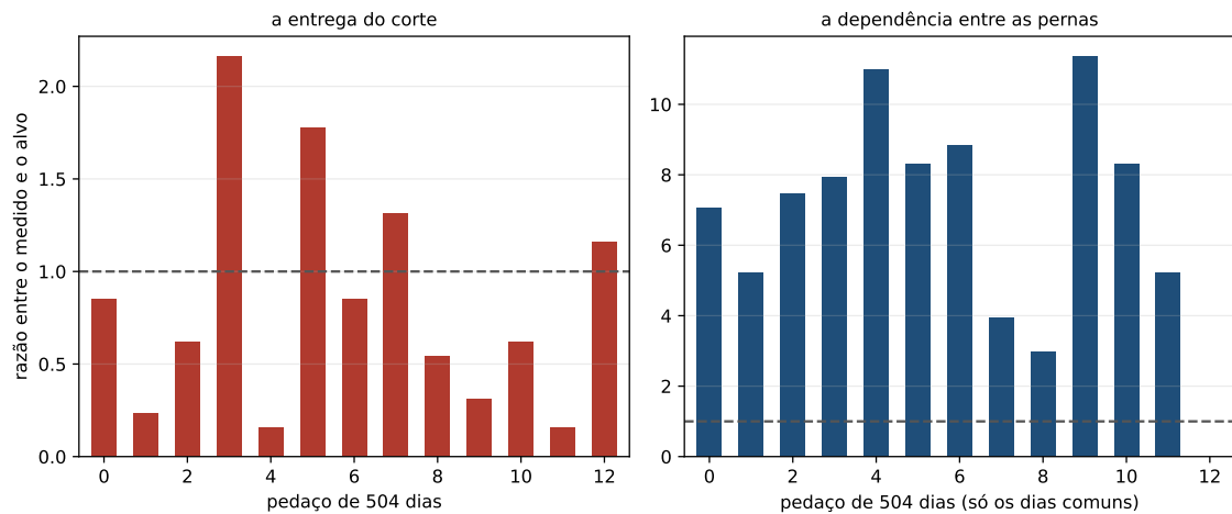
Figura 19.2: As duas conclusões no mesmo tamanho de pedaço, cada uma em razão do seu alvo. À esquerda, a entrega do corte, que atravessa a linha da promessa para os dois lados. À direita, a dependência, que fica sempre bem acima da independência.
