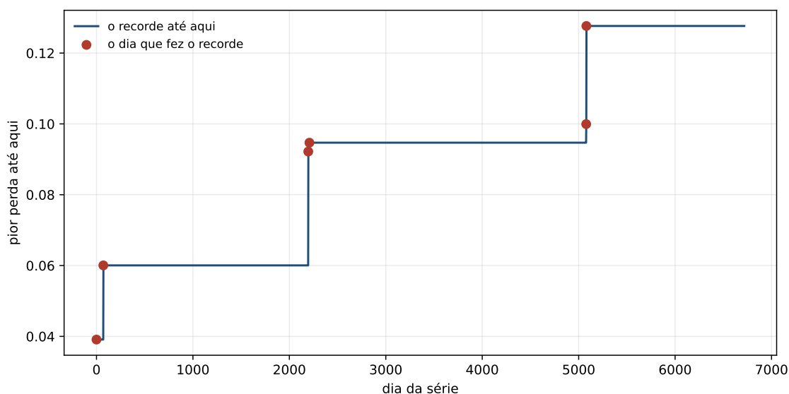
Figura 16.1: A escada do recorde no índice: a pior perda até cada dia, e os dias que ergueram o recorde. São poucos degraus, e cada um deles é um mundo que ainda não tinha sido visto.
