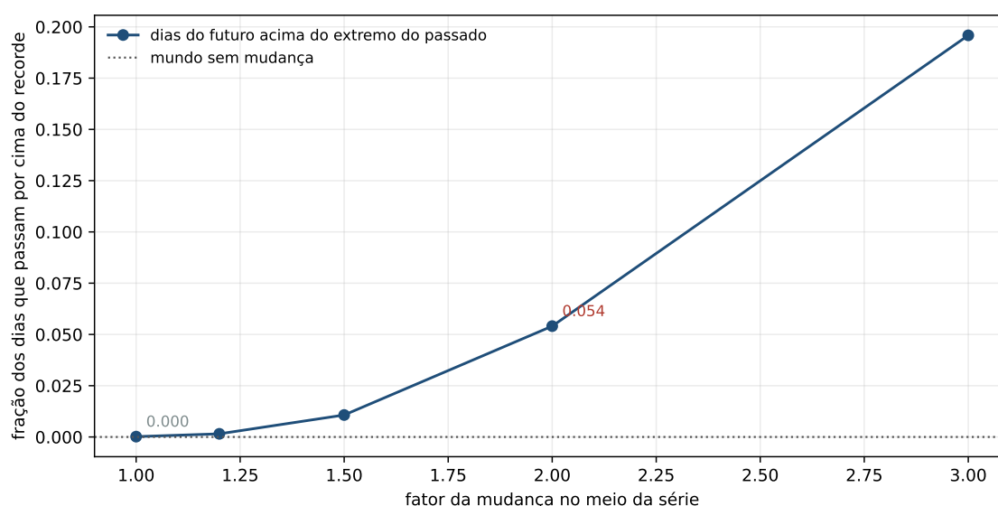
Figura 16.2: A fração dos dias seguintes que passam por cima do recorde de tudo o que veio antes, contra o tamanho da mudança. A linha pontilhada é o mundo que não muda.
