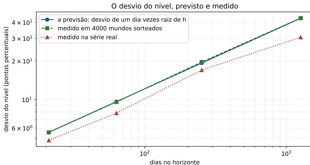
Figura 2.1: O desvio do nível contra o horizonte, nas três leituras. Os dois eixos estão em escala logarítmica, de modo que uma raiz aparece como reta de inclinação meio; a previsão e os mundos sorteados caem juntos, e a série real fica abaixo dos dois.
