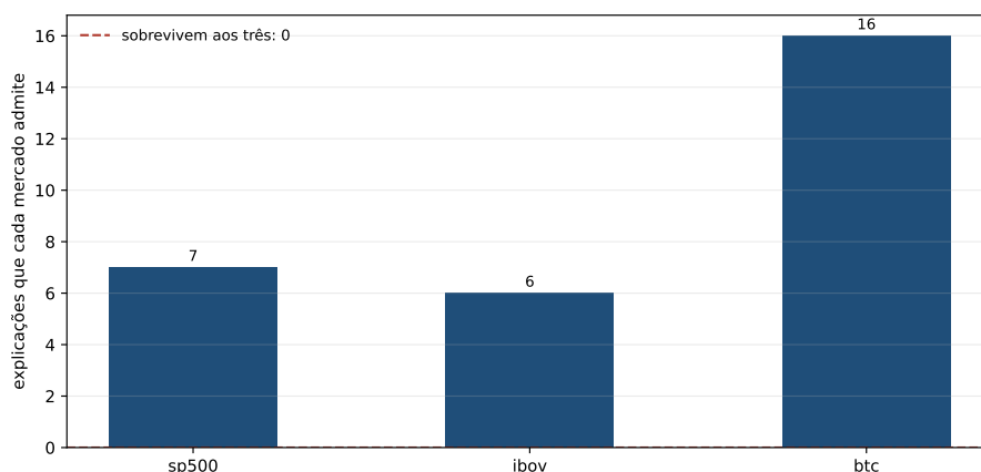
Figura 10.1: Quantas explicações cada mercado admite sozinho, numa varredura, e a linha da interseção. Cada barra é uma varredura só: a do mercado com mais dados vai de 0 a 7 em 10 sementes. A linha colada no eixo é a interseção — nenhuma explicação serve aos três —, e não uma barra que faltou.
