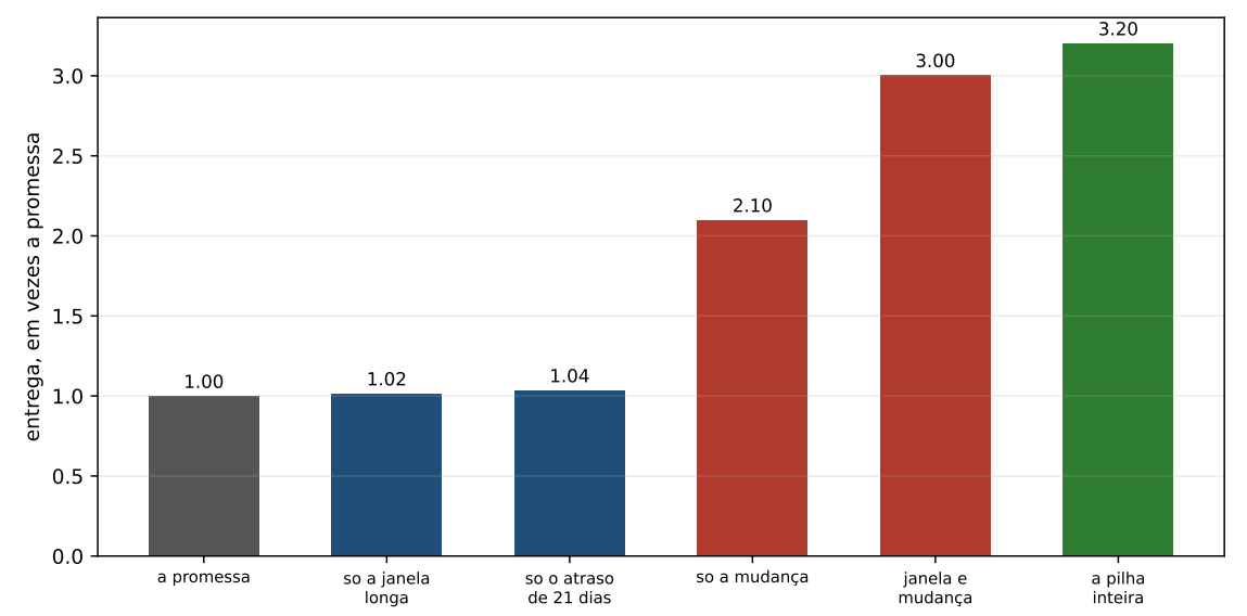
Figura 22.2: A entrega de cada buraco sozinho e a da pilha inteira, em vezes a promessa. A barra verde é a mais alta das seis, e o que essa altura diz é o que o livro inteiro conseguiu: os buracos não se somam, eles se encaixam.
