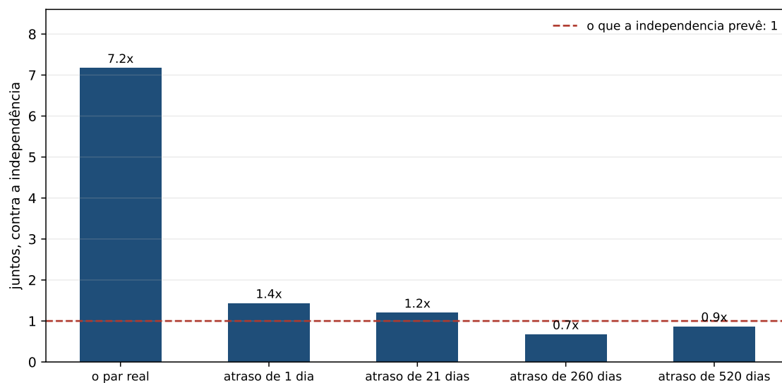
Figura 4.2: À esquerda de cada barra está o par como o mundo fez; as outras quatro são o mesmo par com o segundo mercado deslocado, e a linha tracejada é o que a independência prevê. Quase toda a dependência morre com um único dia de deslocamento.
