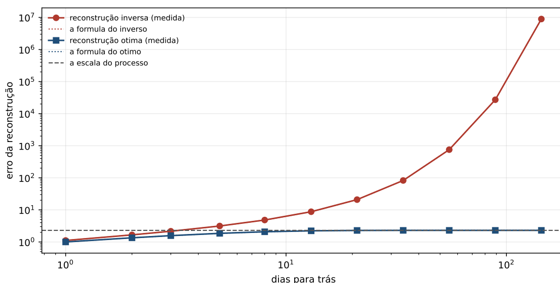
Figura 15.1: O erro das duas reconstruções contra os dias para trás, com a escala do processo como linha de referência. Os pontos são medidos e as linhas pontilhadas são as formas fechadas da proposição 15.1. Os dois eixos são logarítmicos, de modo que a reta do desenho vale uma potência.
