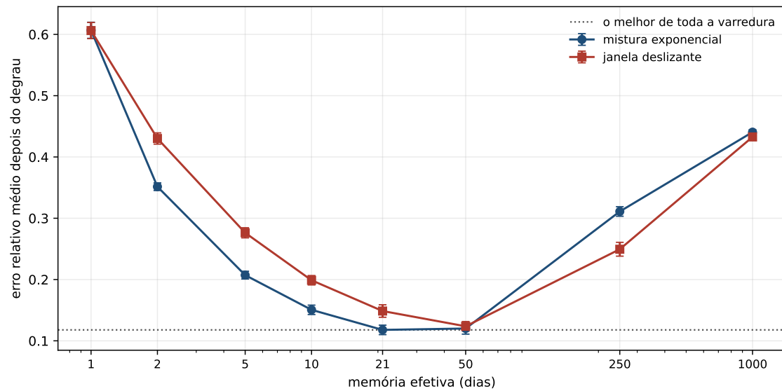
Figura 11.1: O erro depois do degrau contra a memória efetiva, nas duas formas de esquecer. A linha pontilhada é o melhor erro de toda a varredura. O eixo da memória é logarítmico: distâncias iguais no papel são multiplicações iguais no tempo de memória.
