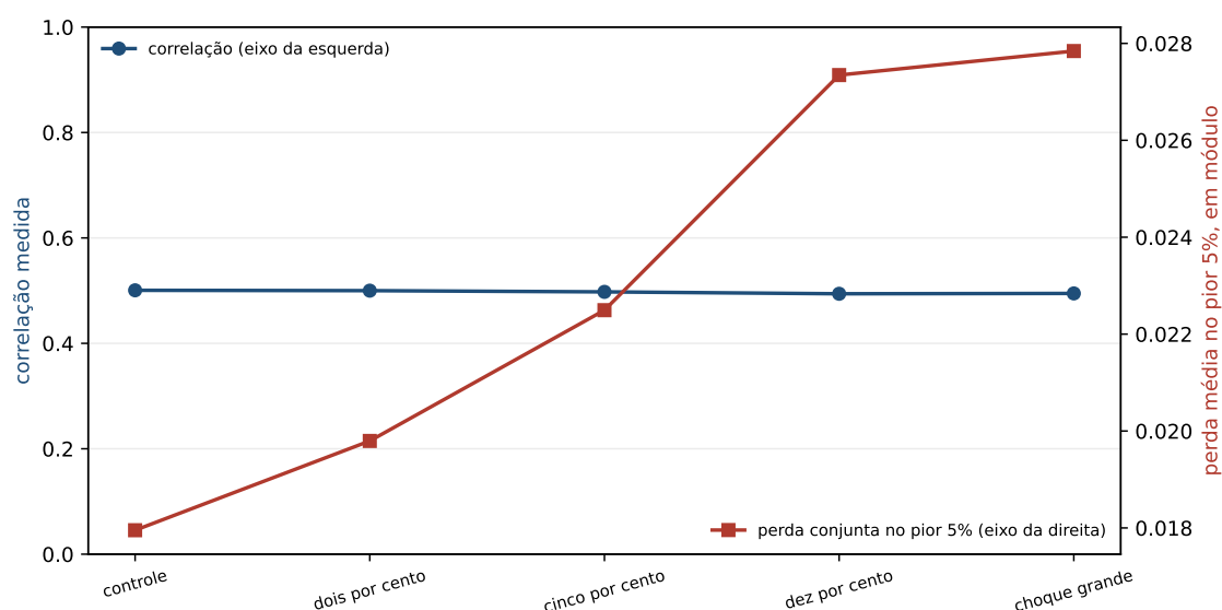
Figura 16.1: A correlação medida e a perda conjunta, contra os cinco mundos. Os dois eixos são diferentes de propósito, e as duas linhas se cruzam no meio do caminho: a reta é a correlação, que anda de 0,4941 a 0,5006, e a que sobe é a perda, que começa abaixo dela e termina acima.
