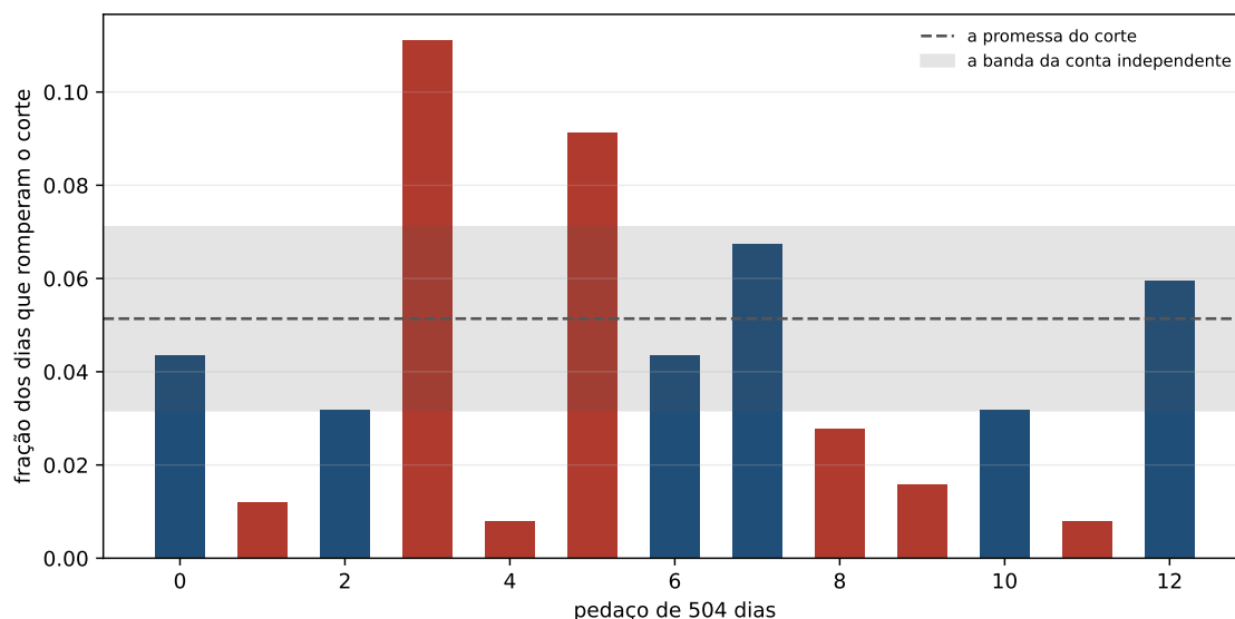
Figura 17.1: A entrega do corte em cada pedaço de 504 dias. A linha tracejada é a conta do corte e a faixa cinza é a banda de quem supõe dias independentes. As barras em vermelho são os pedaços que caem fora da banda.
