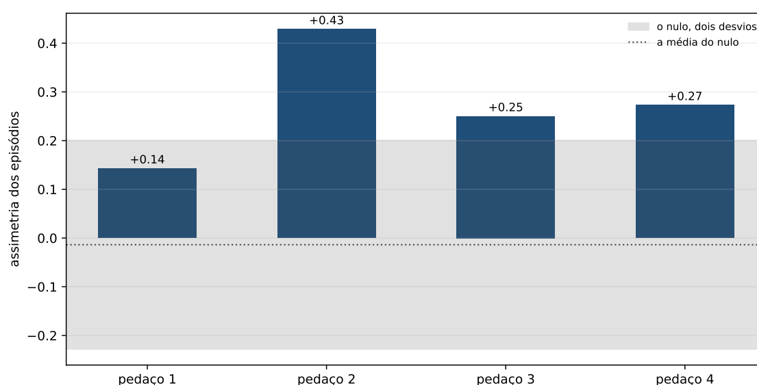
Figura 13.2: A assimetria em cada pedaço do par, contra a faixa do nulo. Os quatro pedaços têm 1613, 1613, 1612 e 1612 dias.
