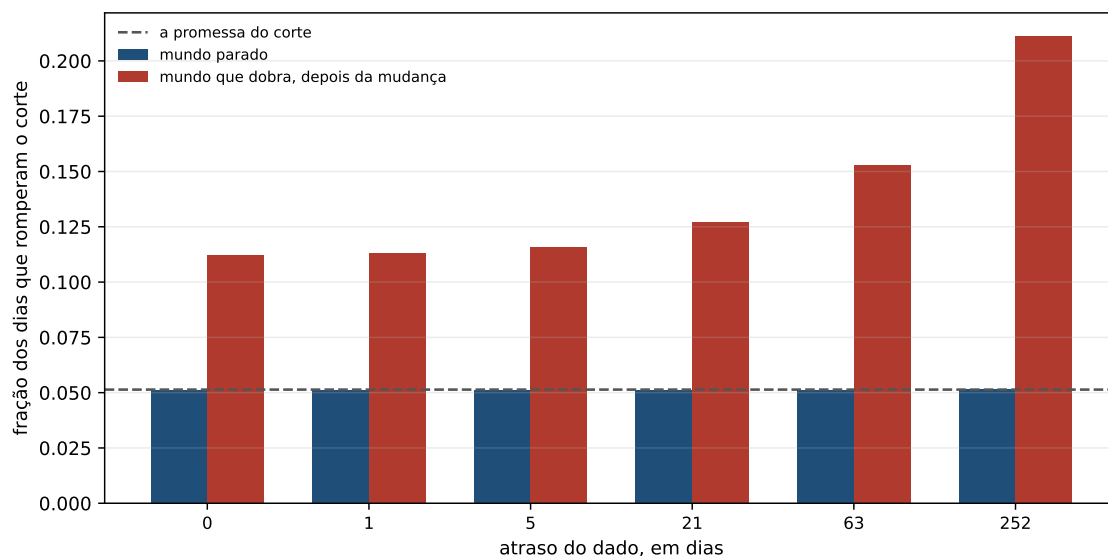
Figura 18.2: O mundo parado e o mundo que dobra, na janela que segue a mudança, por atraso. A barra azul é o controle: ela fica na promessa em todos os atrasos.
