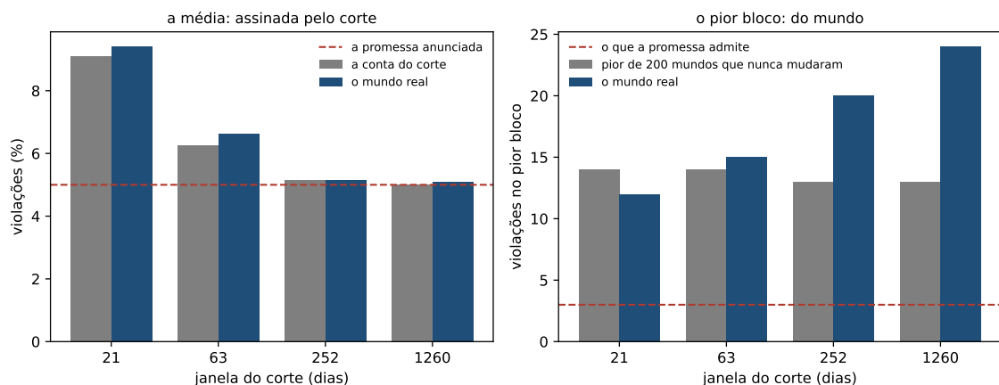
Figura 1.2: As duas leituras, nas quatro janelas. À esquerda, a média: a conta do corte e o mundo real andam juntos. À direita, o pior bloco: o mundo real contra o pior dos 200 mundos que nunca mudam.
