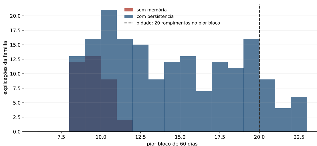
Figura 6.1: Até onde cada família alcança o agrupamento do dado. A linha tracejada é o pior bloco que a série produziu; as barras são quantos membros de cada família chegam a cada valor. A linha colada na borda faz o vazio à esquerda parecer margem apertada; é um muro, e não uma folga.
