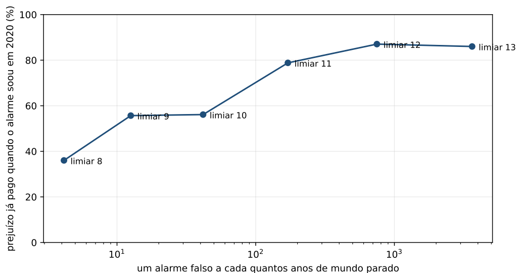
Figura 2.1: A troca em forma de curva: o eixo horizontal é a raridade do falso alarme, em escala logarítmica, e o vertical é o prejuízo já pago no tombo recente. A curva sobe depressa na esquerda e achata na direita.
