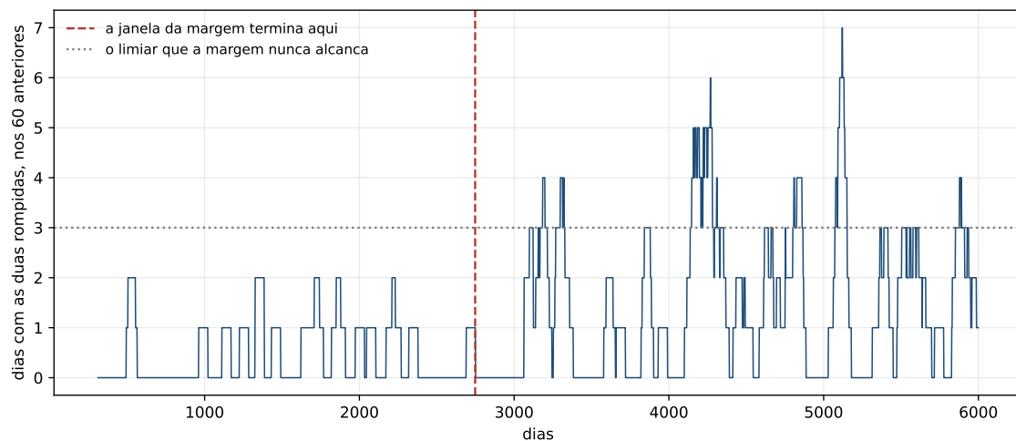
Figura 8.1: A contagem conjunta, dia a dia, com a janela da margem e o limiar que ela nunca alcança. Antes da linha, a série é quase colada no chão; depois, os picos ficam mais altos e mais próximos. A mudança não aparece como degrau: aparece como mais dentes na linha, e quem procura um salto na figura não o encontra.
