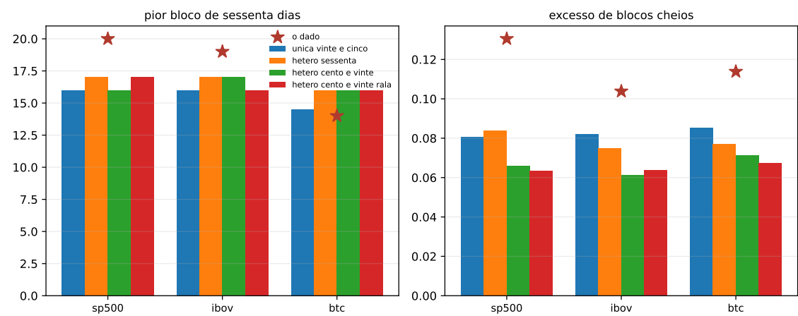
Figura 7.2: A mediana do pior bloco e a do excesso, por configuração e por mercado, com o valor do dado como estrela. As barras são medianas e as estrelas são pontos, sem dispersão desenhada. No painel do pior bloco as faixas de dez a noventa por cento se sobrepõem, de modo que a distância aparente entre barra e estrela é maior do que a distância entre as distribuições.
