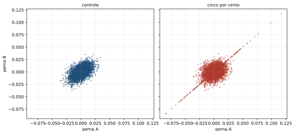
Figura 16.2: A nuvem das duas pernas no mundo gaussiano e no mundo com choque comum. O núcleo elíptico é o mesmo nos dois, e o que o segundo tem a mais são dois braços na diagonal, um para cada canto.
