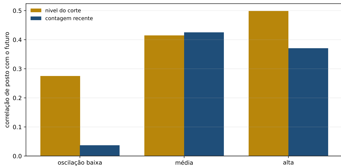
Figura 5.2: O nível do corte e a contagem recente medidos dentro de três faixas de oscilação, onde a oscilação de agora é quase a mesma. O nível não desaparece ao dividir por ela. A barra quase ausente da contagem na faixa calma não é defeito: a contagem é cega justamente onde nada acontece.
