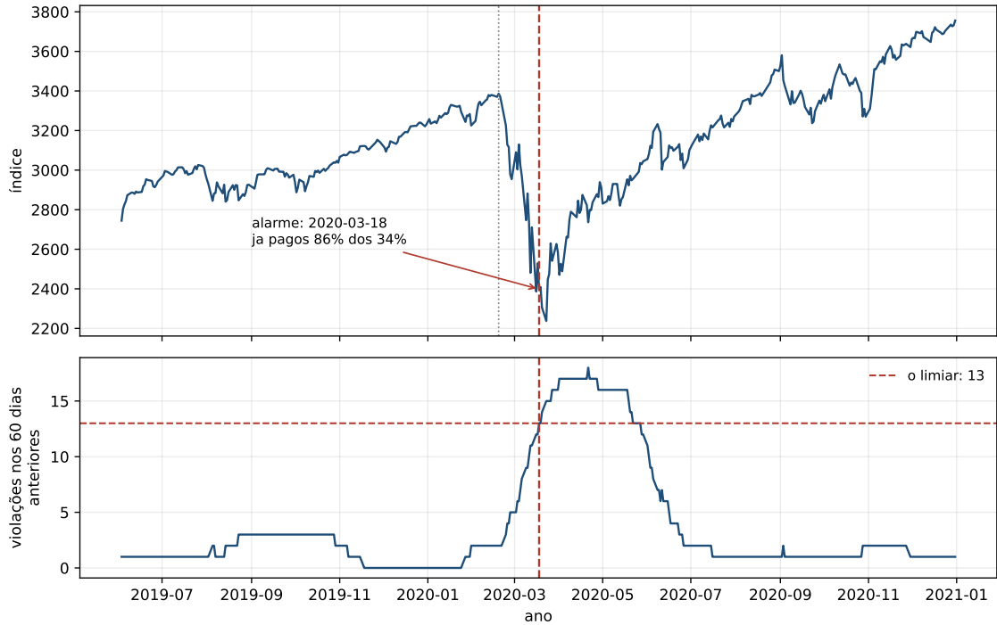
Figura 2.2: O alarme de 18 de março de 2020 visto dos dois lados. Em cima, o índice; embaixo, as violações dos 60 dias anteriores, com o limiar. As duas linhas contam a mesma história — e a de baixo conta depois da de cima.
