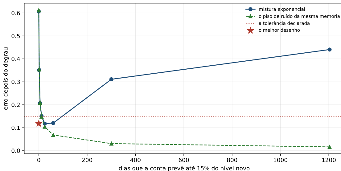
Figura 11.2: O erro depois do degrau contra os dias que a conta do cruzamento prevê até 0,15 do nível novo. A curva tracejada é o piso de ruído da mesma memória: onde ela alcança a curva de cima, o erro deixou de ser atraso e passou a ser tamanho de amostra.
