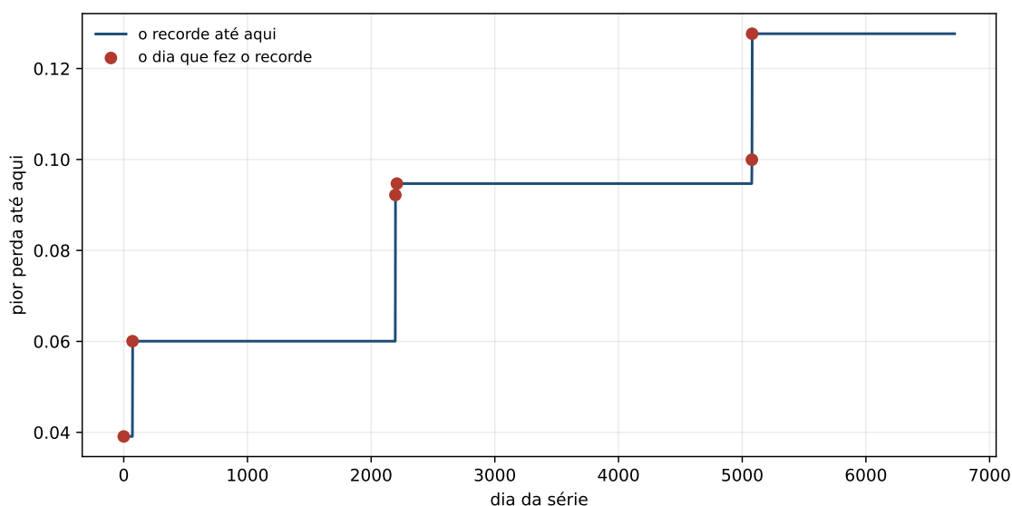
Figura 14.1: A escada do recorde no índice: a pior perda até cada dia, e os dias que ergueram o recorde. São poucos degraus, e cada um deles é um mundo que ainda não tinha sido visto.
