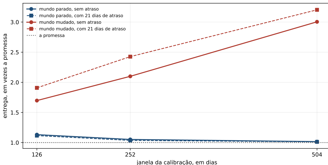
Figura 19.1: A entrega contra a janela da calibração, nos dois mundos e com e sem atraso. As duas curvas do mundo parado descem e as duas do mundo que muda sobem: o mesmo eixo, o sentido trocado.
