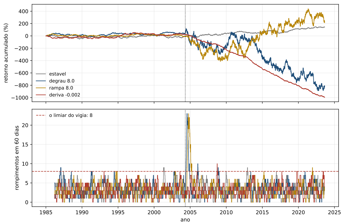
Figura 2.5: Quatro mundos de quarenta anos, cada um com a sua mudança no meio (linha pontilhada). Em cima, o retorno acumulado; embaixo, os rompimentos do corte em 60 dias, com o limiar do vigia: 8. A deriva é o único mundo que cai, e é o único em que a contagem não sobe.
