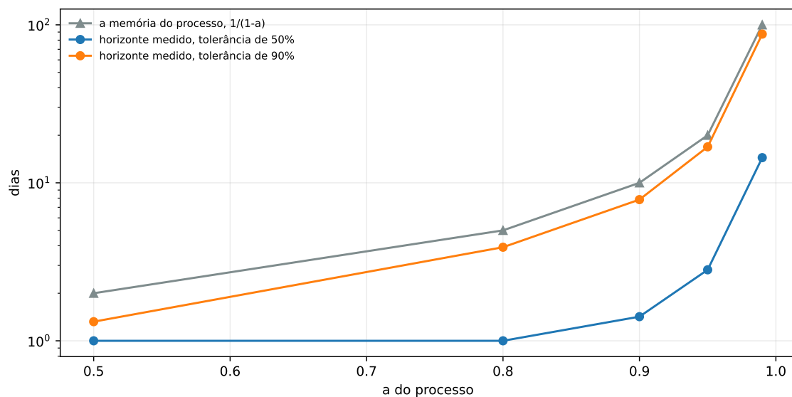
Figura 15.2: A memória do processo e os dois horizontes de recuperação, contra a . São três medidas do mesmo sistema, e cada uma responde a uma pergunta diferente — a curva mais alta é a da memória, e as outras duas são horizontes de recuperação. O eixo dos dias é logarítmico, porque a grandeza só age no fim da escala.
