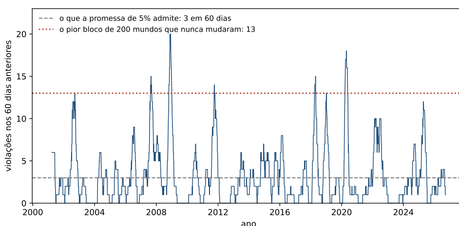
Figura 1.1: Violações nos 60 dias anteriores, dia a dia. A linha tracejada marca o que a promessa de 5% admite; a pontilhada marca o pior bloco que apareceu em 200 mundos que nunca mudam.
