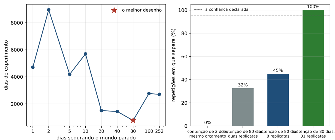
Figura 9.2: À esquerda, o preço do desenho que declara exatamente a diferença medida. À direita, a promessa do desenho verificada por repetição do experimento inteiro: a fração das repetições em que os dois intervalos de fato deixam de se cruzar.
