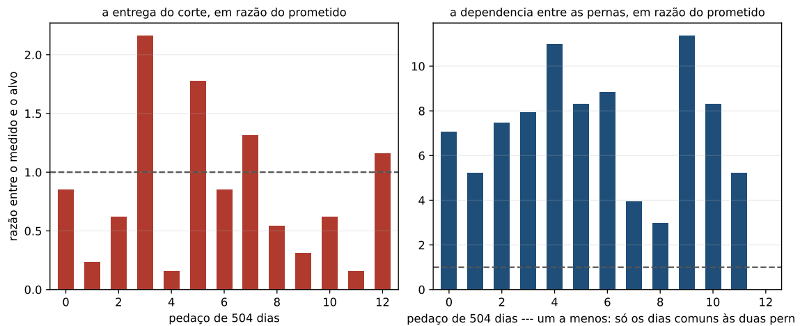
Figura 17.2: As duas conclusões no mesmo tamanho de pedaço, cada uma em razão do seu alvo. À esquerda, a entrega do corte, que atravessa a linha da promessa para os dois lados. À direita, a dependência, que fica sempre bem acima da independência.
