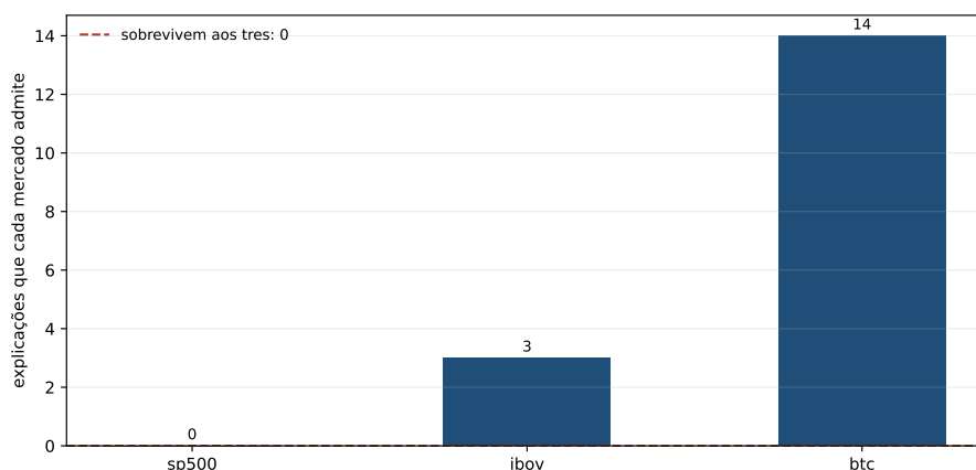
Figura 7.1: Quantas explicações cada mercado admite sozinho, e a linha da interseção. A primeira barra não aparece porque o valor dela é o zero: o mercado com mais dados é o que não admite explicação nenhuma. Barra ausente e barra que faltou têm a mesma cara, e a linha colada no eixo some.
