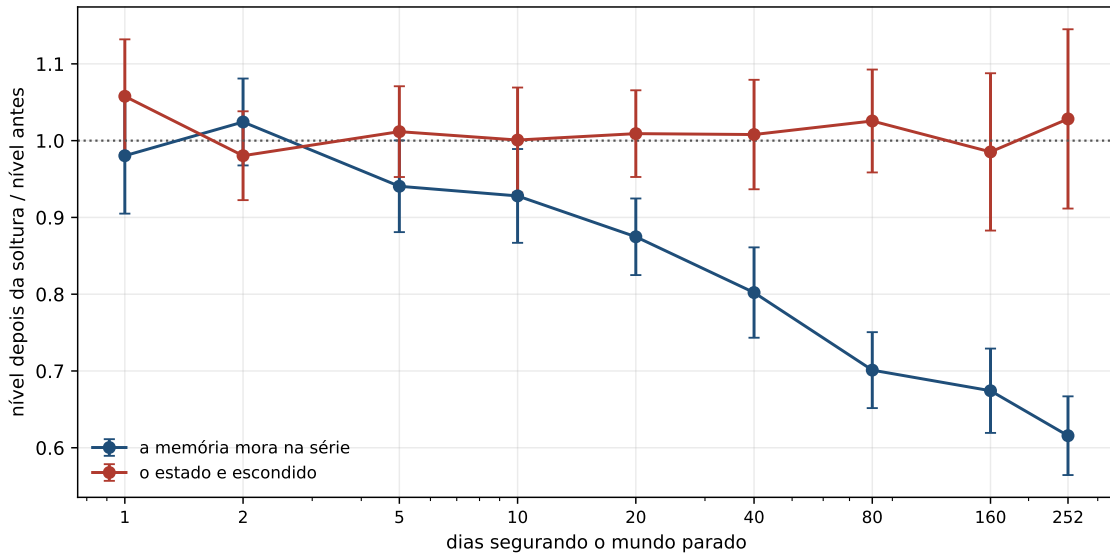
Figura 9.1: A resposta dos dois mundos contra o tempo de contenção, com as barras de dispersão desenhadas sobre 60 replicatas por ponto. A linha pontilhada é a resposta de um mundo que volta ao que era. O eixo horizontal é logarítmico, de modo que a distância entre as últimas marcas vale mais dias do que a figura sugere.
