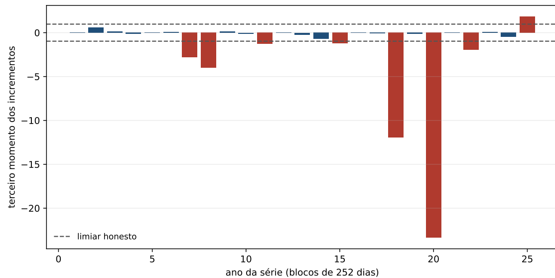
Figura 12.2: O terceiro momento dos incrementos, ano a ano, no índice americano, com o limiar honesto. As barras em vermelho são os anos em que o vigia alarmaria.
