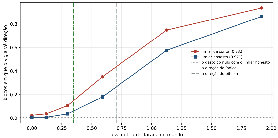
Figura 12.1: O acerto do vigia contra a direção declarada do mundo, nos dois limiares. As linhas verticais marcam a direção medida no índice e no Bitcoin, e a linha pontilhada é o que o vigia gasta à toa com o limiar honesto.
