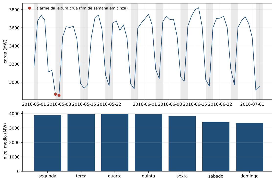
Figura 3.1: Nove semanas de carga dinamarquesa. Os fins de semana estão em cinza, e os dois pontos são os alarmes da leitura crua: os dois caem no cinza. Embaixo, o perfil semanal médio dos cinco anos — o desenho que a leitura crua estava medindo sem saber.
