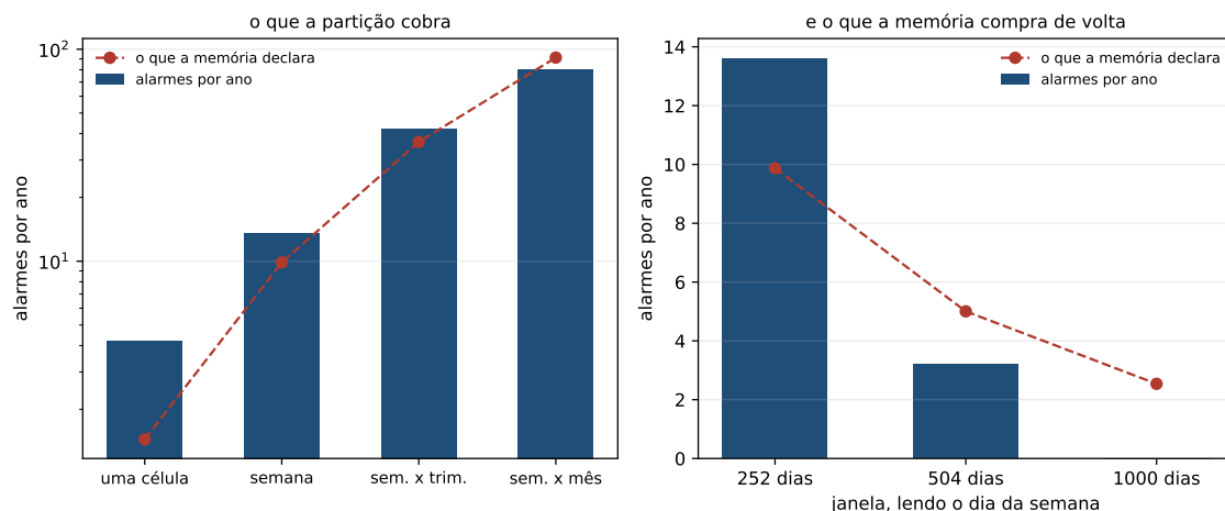
Figura 3.2: À esquerda, o que a partição cobra: alarmes por ano contra o que a memória declara, para as quatro leituras da tabela 3.2. O eixo dos alarmes é logarítmico, de modo que distâncias iguais no papel são multiplicações iguais no preço. À direita, o que a memória compra de volta, com a janela crescendo e a partição semanal fixa.
