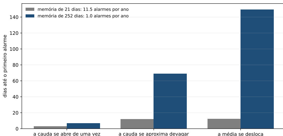
Figura 2.3: Dias até o primeiro alarme, por forma de mudança, em dois orçamentos: a memória de um mês, à esquerda de cada par, e a de um ano, à direita. O orçamento mais raro paga a diferença entre as formas.
