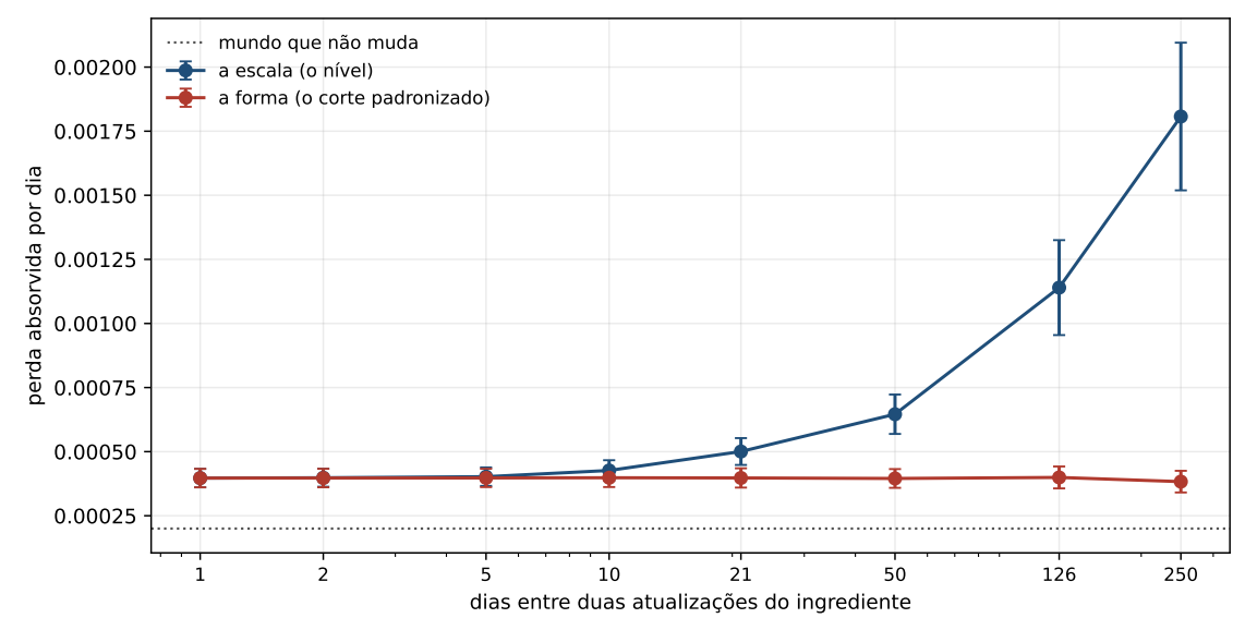
Figura 10.1: A perda absorvida contra o tempo entre duas atualizações, atualizando um ingrediente por vez. O eixo dos tempos é logarítmico, de modo que a distância entre as últimas marcas vale muito mais dias do que a figura sugere. A linha pontilhada é o mesmo desenho num mundo que não muda.
