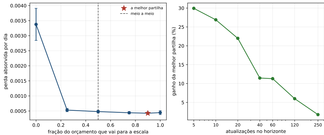
Figura 10.2: À esquerda, a perda contra a fração do orçamento que vai para a escala, com a dispersão entre mundos, o eixo da fração é linear, de modo que os três últimos pontos ficam amontoados à direita. À direita, o ganho da melhor partilha contra o tamanho do orçamento: a vantagem de escolher bem encolhe quando o orçamento engorda.
