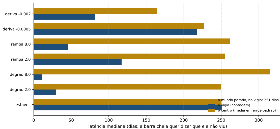
Figura 2.4: A latência mediana de cada instrumento, forma por forma: a contagem de rompimentos contra a média da janela em erros-padrão dela mesma. A linha tracejada é o que o mundo parado produz no primeiro deles, e a barra cheia é o instrumento que ficou sem alarme dentro do horizonte — duas barras que terminam no mesmo lugar não são empate, porque uma delas não chegou.
