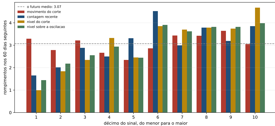
Figura 5.1: O futuro médio em cada décimo dos quatro sinais, com a média geral como linha. Três dos quatro sobem; o do movimento do corte atravessa o gráfico de lado. A leitura é seguir uma cor de ponta a ponta: comparar décimos vizinhos perde a tendência, que é o que a figura mostra.
