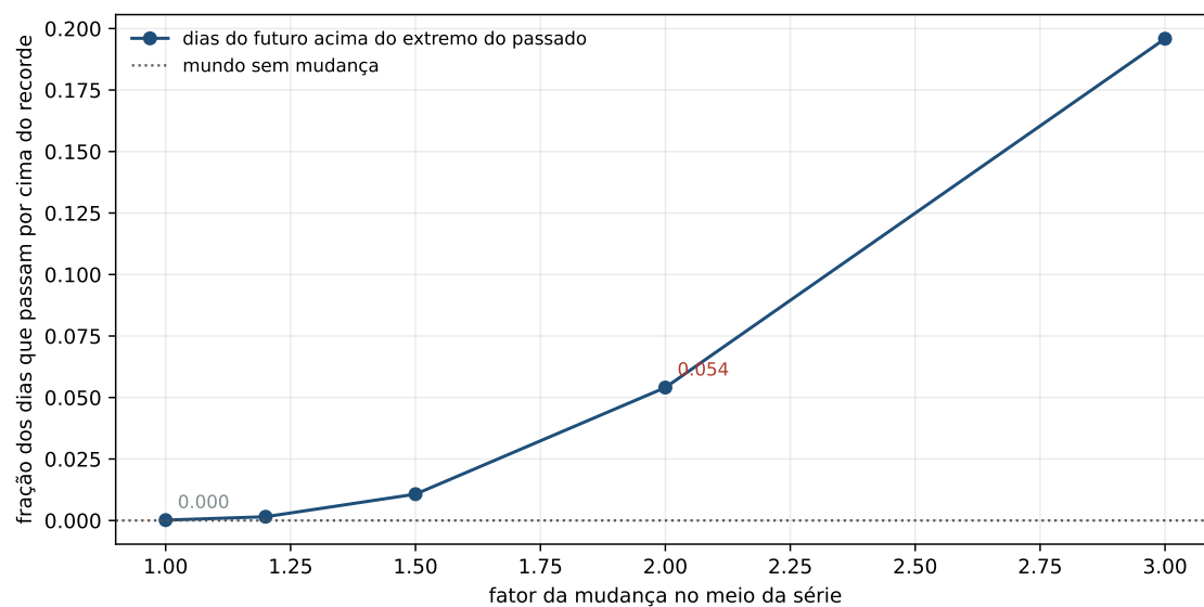
Figura 14.2: A fração dos dias seguintes que passam por cima do recorde de tudo o que veio antes, contra o tamanho da mudança. A linha pontilhada é o mundo que não muda.
