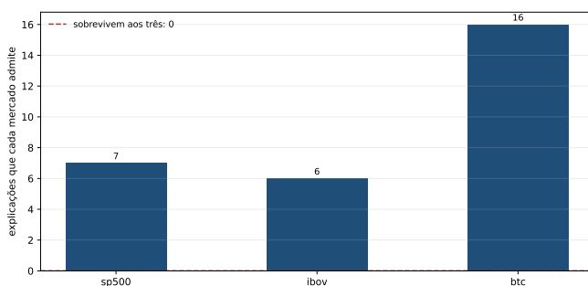
Figura 13.1: Quantas explicações cada mercado admite sozinho, numa varredura, e a linha da interseção. Cada barra é uma varredura só: a do mercado com mais dados vai de 0 a 7 em 10 sementes. A linha colada no eixo é a interseção — nenhuma explicação serve aos três —, e não uma barra que faltou.
