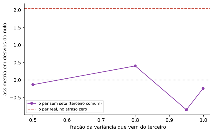
Figura 23.2: A assinatura em desvios do par sem seta — duas pernas independentes movidas por um terceiro comum, com as margens do par real — contra a fração da variância que vem do terceiro. A linha tracejada é o par real no atraso zero. Em nenhuma fração o par sem seta alcança a linha: a confusão sozinha não escreve a frase.
