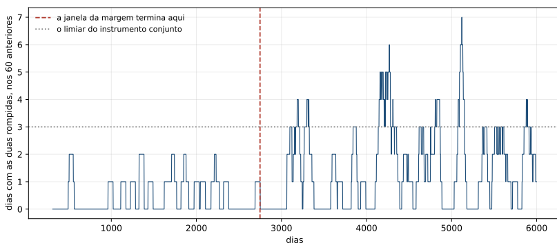
Figura 15.1: A contagem conjunta, dia a dia, com a janela da margem e o limiar do instrumento conjunto. Antes da linha, a série é quase colada no chão; depois, os picos ficam mais altos e mais próximos. A mudança não aparece como degrau: aparece como mais dentes na linha, e quem procura um salto na figura não o encontra.
