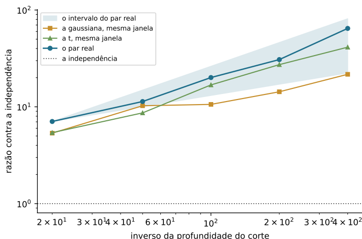
Figura 27.1: A razão contra a independência em cada profundidade, em log-log — a inclinação de cada curva é a taxa com que a junta cai. O par real (azul, com a faixa do intervalo por bootstrap de blocos) cresce de 7,06 a 64,56; a gaussiana da mesma janela (laranja) cresce menos; a t (verde) acompanha o par de perto. A linha pontilhada é a independência, que não cresce.
