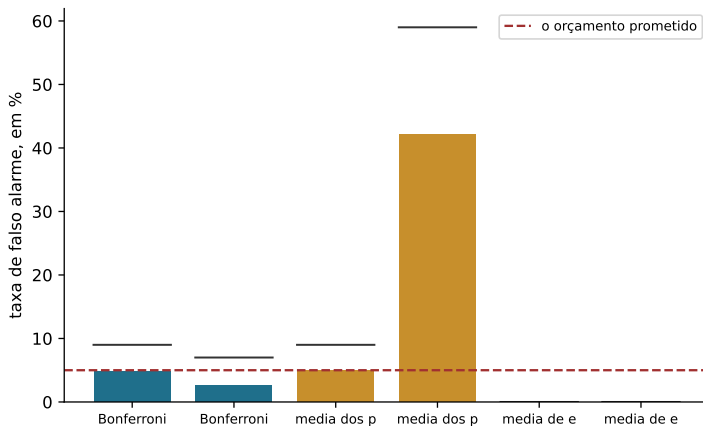
Figura 5.2: As três fusões nos dois mundos, contra o orçamento prometido (linha tracejada). A média dos p-valores entrega o combinado no mundo calado e oito vezes mais no que fala; Bonferroni e a média de e-values ficam abaixo da linha nos dois. O traço é o pior lote de sortes.
