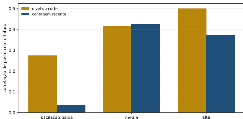
Figura 9.2: O nível do corte e a contagem recente medidos dentro de três faixas de oscilação, onde a oscilação de agora é quase a mesma. O nível não desaparece ao dividir por ela. A barra quase ausente da contagem na faixa calma não é defeito: a contagem é cega justamente onde nada acontece.
