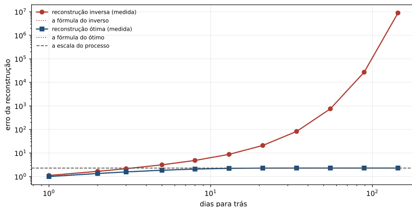
Figura 25.1: O erro das duas reconstruções contra os dias para trás, com a escala do processo como linha de referência. Os pontos são medidos e as linhas pontilhadas são as formas fechadas da proposição 25.1. Os dois eixos são logarítmicos, de modo que a reta do desenho vale uma potência.
