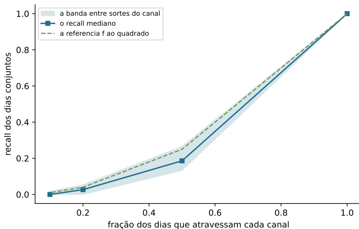
Figura 28.3: O recall dos dias conjuntos verdadeiros contra a fração dos dias que atravessam cada canal, com a banda entre sortes do canal — a incerteza aqui é qual dia atravessou, e não a reamostragem dos que vieram. A linha tracejada é a referência do quadrado: um dia conjunto só é visto se os dois canais o deixarem passar. O recall mediano fica abaixo dela desde a metade: a recalibração sobre séries com buracos perde além do que o canal corta.
