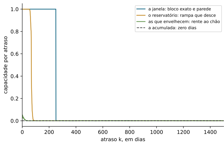
Figura 29.3: O perfil da capacidade por atraso. A janela é bloco exato com parede; o reservatório é rampa que desce — no atraso 68 a capacidade por atraso cai à metade do primeiro atraso; e as duas que envelhecem ficam rente ao chão desde o primeiro dia.
