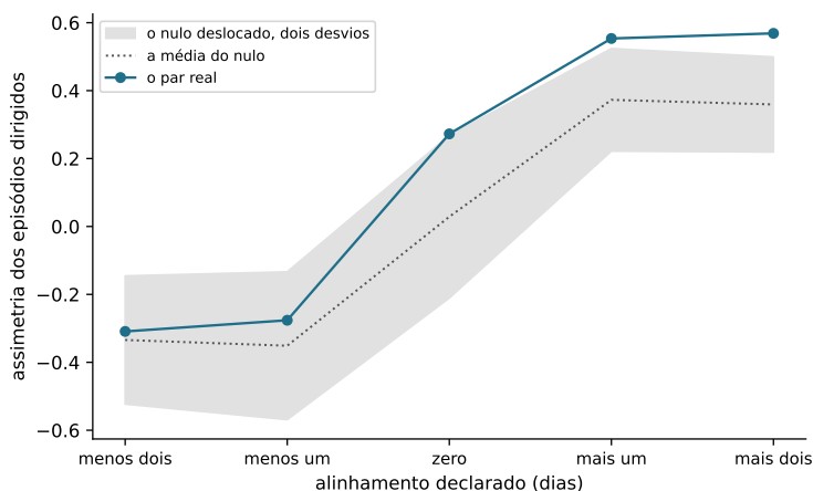
Figura 23.1: A assimetria dos episódios dirigidos no par real, contra o alinhamento declarado — com a faixa de dois desvios do nulo deslocado em cada ponto. No alinhamento do relógio declarado (menos um: o índice de ontem contra o Ibovespa de hoje) a assimetria troca de sinal e cai ao nulo; no alinhamento que dá ao Ibovespa a vantagem cronológica (mais um e mais dois) ela cresce acima de dois desvios. A ordem segue o head start, não a causa.
