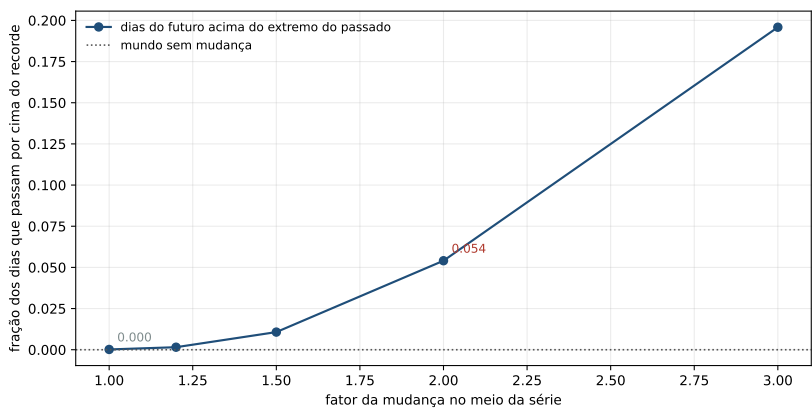
Figura 24.2: A fração dos dias seguintes que passam por cima do recorde de tudo o que veio antes, contra o tamanho da mudança. A linha pontilhada é o mundo que não muda.
