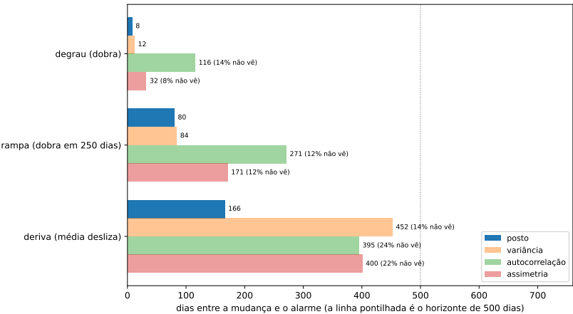
Figura 10.1: A mesma tabela em barras: três grupos de forma, quatro instrumentos, o posto em azul cheio e as pernas da receita em meio-tom. A linha pontilhada é o horizonte de 500 dias. No degrau a barra do posto é a menor de todas; na rampa, posto e variância são quase a mesma barra; na deriva, as três barras da receita são as mais longas do desenho.
