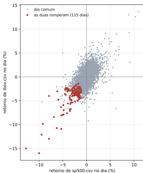
Figura 8.1: Os dois mercados, dia a dia. Cada ponto é um dia, com o retorno de um no eixo horizontal e o do outro no vertical; as linhas em zero partem o plano em quadrantes. Os 115 dias em que as duas pernas romperam estão todos no quadrante de baixo à esquerda, e nenhum em qualquer outro lugar do plano.
