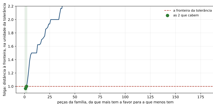
Figura 11.3: A folga de cada peça da família, da que mais tem a favor para a que menos tem. A linha tracejada é a fronteira da tolerância e a faixa verde, as 2 peças que o capítulo conta. A mais distante das 180 está a 6,5 tolerâncias.
