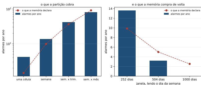
Figura 7.2: À esquerda, o que a partição cobra: alarmes por ano contra o que a memória declara, para as quatro leituras da tabela 7.2. O eixo dos alarmes é logarítmico, de modo que distâncias iguais no papel são multiplicações iguais no preço. À direita, o que a memória compra de volta, com a janela crescendo e a partição semanal fixa.
