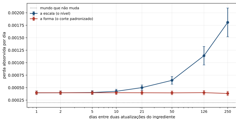
Figura 17.1: A perda absorvida contra o tempo entre duas atualizações, atualizando um ingrediente por vez. O eixo dos tempos é logarítmico, de modo que a distância entre as últimas marcas vale muito mais dias do que a figura sugere. A linha pontilhada é o mesmo desenho num mundo que não muda.
