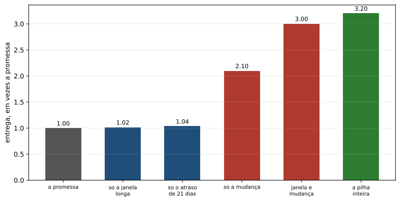
Figura 33.2: A entrega de cada buraco sozinho e a da pilha inteira, em vezes a promessa. A barra verde é a mais alta das seis, e o que essa altura diz é o que o livro inteiro perseguiu: os buracos não se somam, eles se encaixam.
