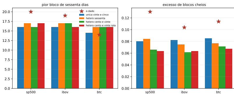
Figura 13.2: A mediana do pior bloco e a do excesso, por configuração e por mercado, com o valor do dado como estrela. As barras são medianas e as estrelas são pontos, sem dispersão desenhada. No painel do pior bloco as faixas de dez a noventa por cento se sobrepõem, de modo que a distância aparente entre barra e estrela é maior do que a distância entre as distribuições.
