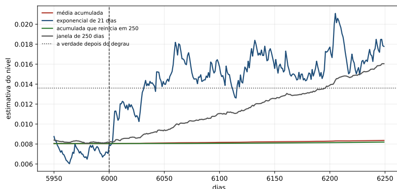
Figura 29.2: Os quatro estimadores em torno do dia do degrau, contra a verdade. Depois dele a exponencial de vinte e um dias reage e oscila em volta da linha; a janela sobe em rampa, porque vai sendo preenchida por dias novos; e a média acumulada e a que reinicia ficam paradas — elas carregam tanto passado que o degrau quase não as move dentro do horizonte da decisão.
