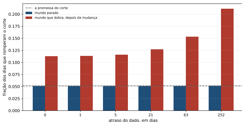
Figura 31.2: O mundo parado e o mundo que dobra, por atraso — o parado medido na série inteira e o que dobra na janela que segue a mudança. A barra azul é o controle: ela fica na promessa em todos os atrasos.
