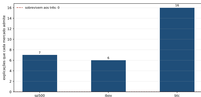
Figura 13.1: Quantas explicações cada mercado admite sozinho, numa varredura, e a linha da interseção. Cada barra é uma varredura só: a do mercado com mais dados vai de 0 a 7 em 10 sementes. A linha colada no eixo é a interseção — nenhuma explicação serve aos três —, e não uma barra que faltou.
