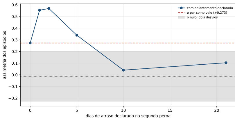
Figura 22.1: A assimetria contra o atraso declarado na segunda perna. A faixa cinza é o nulo a dois desvios sem deslocamento, a linha tracejada é o par como veio, e a curva é o par com o atraso declarado — que o nulo também sofre, e é o que o texto mede.
