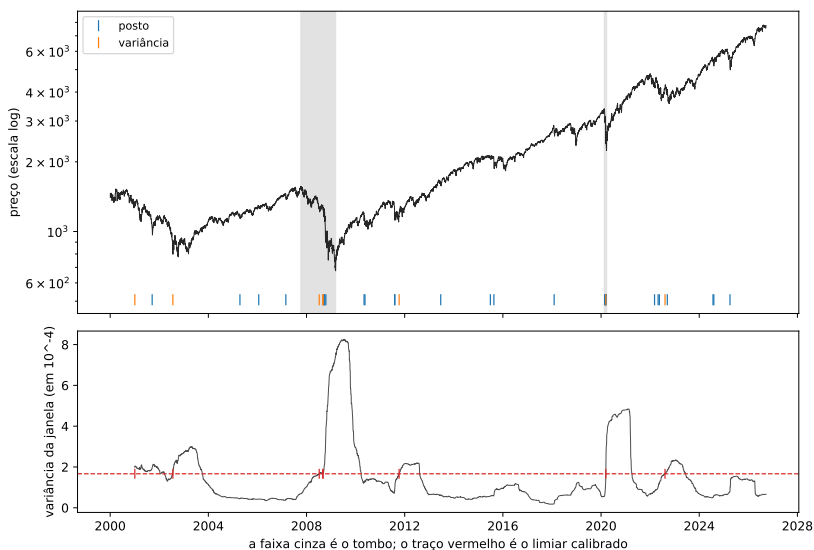
Figura 10.2: O S&P 500 em escala log com os dois tombos em faixa cinza, as marcas de alarme na base — o posto em azul, a variância em laranja — e, embaixo, a variância da janela com o limiar calibrado em traço vermelho. Os dois instrumentos se acumulam nas mesmas regiões de turbulência; na faixa de 2020, a marca do posto cai nos primeiros dias e a da variância vem perto do fim da faixa.
