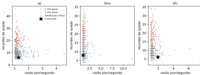
Figura 12.2: A decisão: a nuvem de mundos de cada família (a razão contra a contagem de marcas) e a estrela do mercado, nos três painéis. As estrelas caem na parte baixa das nuvens do t e sempre abaixo das nuvens da ramificação, que moram acima das marcas que os mercados fazem. No Bitcoin, a estrela está à direita da nuvem cinza — o t de oito graus não faz razão de 1,956: o teto dele é 1,514.
