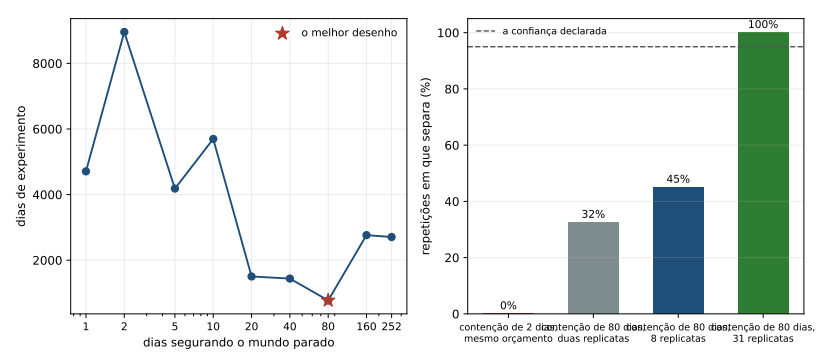
Figura 16.2: À esquerda, o preço do desenho que declara exatamente a diferença medida. À direita, a promessa do desenho verificada por repetição do experimento inteiro: a fração das repetições em que os dois intervalos de fato deixam de se cruzar.
