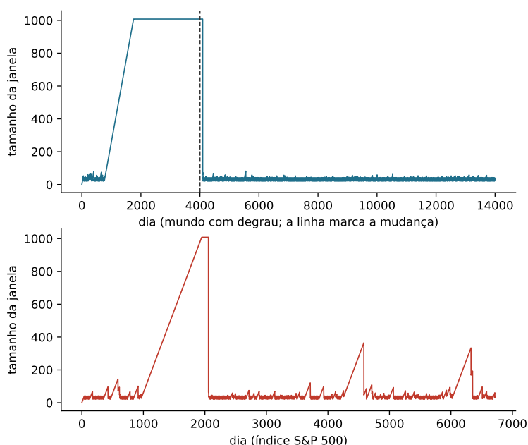
Figura 20.2: O tamanho que o dado escolhe, dia a dia: acima, um mundo com degrau (a linha pontilhada marca a mudança) — a janela despenca do máximo e nunca mais envelhece: oscila rente ao chão declarado; abaixo, o índice real — a janela quase não consegue crescer, e termina colada perto do chão de 21 dias.
