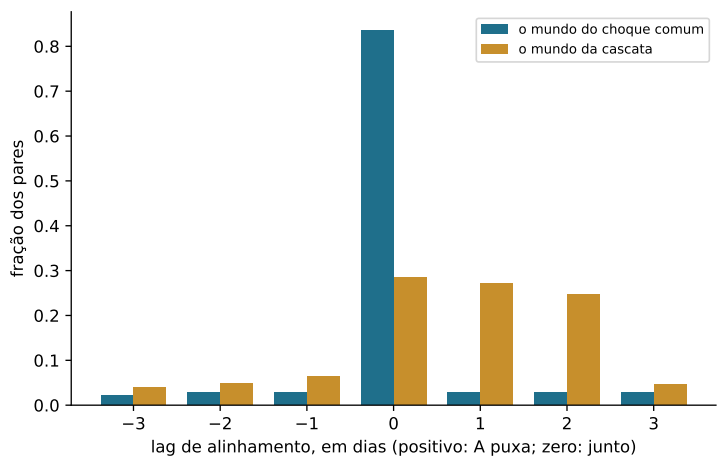
Figura 23.3: Os histogramas de alinhamento dos dois mundos, na mesma contagem conjunta. O choque concentra quase tudo no zero; a cascata espalha entre o zero, o um e o dois — o atraso da propagação é visível no alinhamento. O que o histograma não devolve é a fração de B que depende de A: esse número não mora em nenhuma barra.
