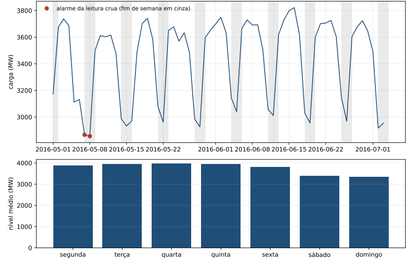
Figura 7.1: Nove semanas de carga dinamarquesa. Os fins de semana estão em cinza, e os dois pontos são os alarmes da leitura crua: os dois caem no cinza. Embaixo, o perfil semanal médio dos cinco anos — o desenho que a leitura crua estava medindo sem saber.
