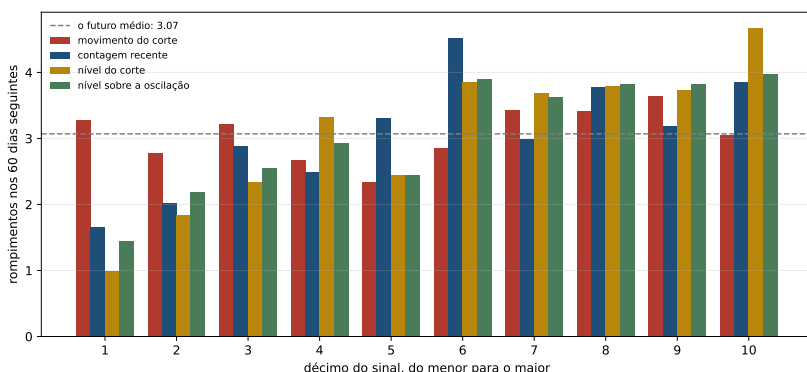
Figura 9.1: O futuro médio em cada décimo dos quatro sinais, com a média geral como linha. Três dos quatro sobem; o do movimento do corte atravessa o gráfico de lado. A leitura é seguir uma cor de ponta a ponta: comparar décimos vizinhos perde a tendência, que é o que a figura mostra.
