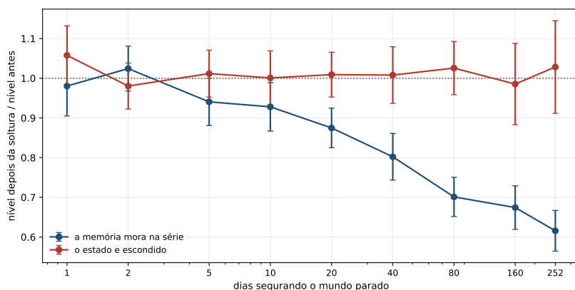
Figura 16.1: A resposta dos dois mundos contra o tempo de contenção, com as barras de dispersão desenhadas sobre 60 replicatas por ponto. A linha pontilhada é a resposta de um mundo que volta ao que era. O eixo horizontal é logarítmico, de modo que a distância entre as últimas marcas vale mais dias do que a figura sugere.
