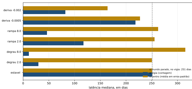
Figura 6.2: A latência mediana de cada instrumento, forma por forma: a contagem de rompimentos contra a média da janela em erros-padrão dela mesma. A linha tracejada é o que o mundo parado produz no primeiro deles, e duas barras que terminam no mesmo lugar merecem cuidado: o mundo parado não é uma forma de mudança, e é ele que reaparece em toda forma.
