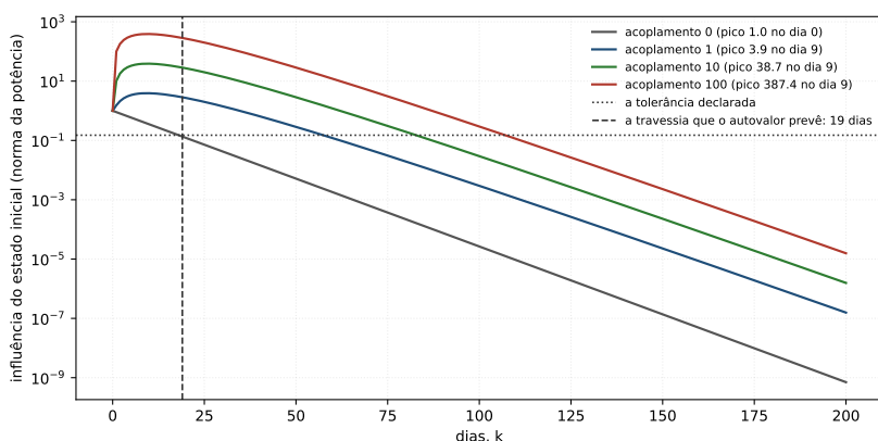
Figura 25.3: A influência do estado inicial, dia a dia, para os quatro acoplamentos. O eixo vertical é logarítmico, de modo que uma queda exponencial sai reta: só a curva do acoplamento zero é reta, e as outras três sobem antes de descer, virando todas no mesmo dia. A linha tracejada marca os 19 dias que o autovalor prevê e a pontilhada, a tolerância de 0,15.
