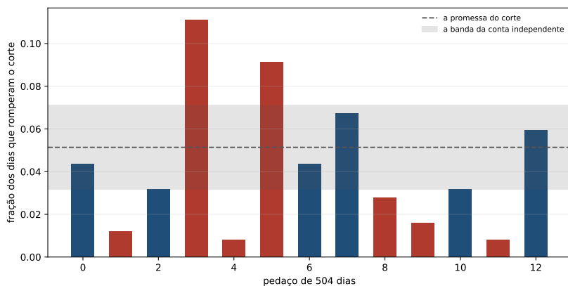
Figura 30.1: A entrega do corte em cada pedaço de 504 dias. A linha tracejada é a conta do corte e a faixa cinza é a banda de quem supõe dias independentes. As barras em vermelho são os pedaços que caem fora da banda.
