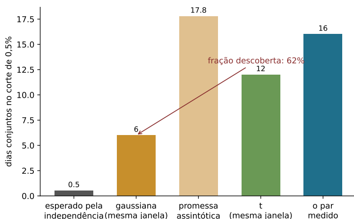
Figura 27.2: Dias conjuntos no corte de meio por cento: o esperado pela independência, o que a gaussiana da mesma janela entrega, o que a extrapolação assintótica promete, o que a t da mesma janela entrega, e o medido no par. A seta marca a fração descoberta de quem dimensionou a proteção pela gaussiana da janela.
