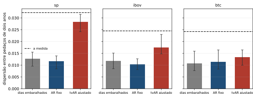
Figura 14.3: A escada da mesma tabela, em barras: a barra do ajuste que anda é a mais alta no índice e quase toca a linha da medida; no Ibovespa fica no meio do caminho; no Bitcoin as três ficam juntas e longe da linha. As barras são medianas de reamostras, com a faixa entre décimos.
