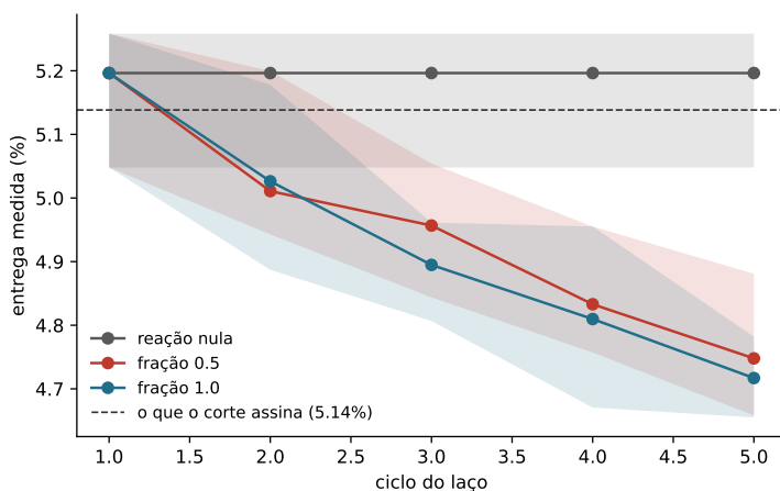
Figura 18.1: A entrega ciclo a ciclo quando a venda cai no próprio dia do rompimento (atraso zero): mediana entre mundos e faixa dos vinte aos oitenta por cento, para a reação nula e as duas frações vendidas, contra a linha do que o corte assina. A reação puxa a entrega para baixo ciclo a ciclo; a faixa entre mundos mal se estreita.
