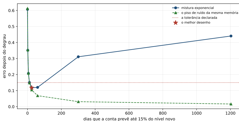
Figura 19.2: O erro depois do degrau contra os dias que a conta do cruzamento prevê até 0,15 do nível novo. A curva tracejada é o piso de ruído da mesma memória: onde ela alcança a curva de cima, o erro deixou de ser atraso e passou a ser tamanho de amostra.
