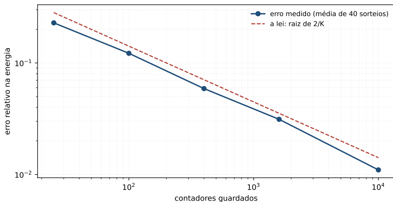
Figura 32.2: O erro do esboço contra o número de contadores guardados, nas duas escalas logarítmicas, com a reta da lei ao lado. As duas linhas são paralelas , e a medida fica abaixo da lei em toda a extensão: a média de uma estimativa simétrica custa cerca de oito décimos do desvio dela, e é isso que a distância entre as duas linhas mede.
