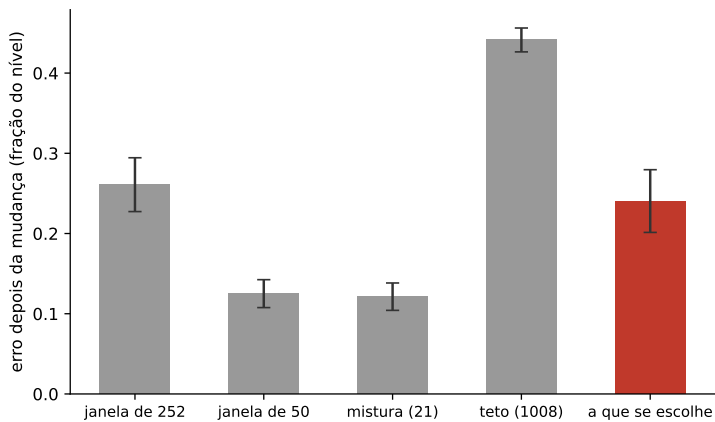
Figura 20.1: O erro no ano seguinte à mudança, cinco concorrentes, mediana e dispersão entre mundos. A que se escolhe sozinha (vermelha) cai do teto para a vizinhança da janela de um ano — e para ali não desce: a escolha certa para este mundo, a janela de cinquenta dias, fica a mais de três dispersões de distância.
