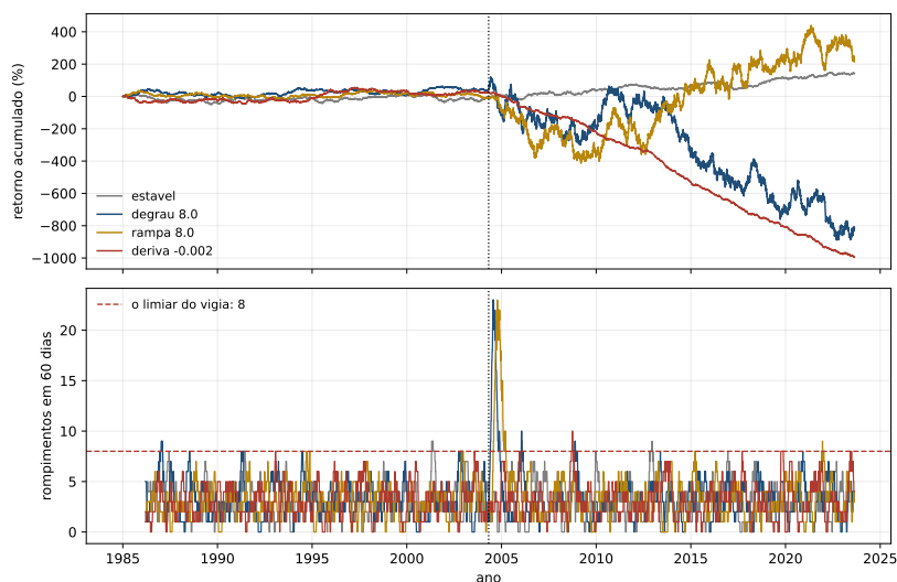
Figura 6.3: Três mundos de quarenta anos com a mudança no meio (linha pontilhada), e o mundo parado como chão. Em cima, o retorno acumulado; embaixo, os rompimentos do corte em 60 dias, com o limiar do vigia. A deriva é o único mundo que cai, e é o único em que a contagem não sobe.
