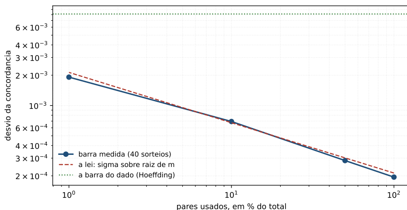
Figura 8.3: A barra do sorteio contra a fração dos pares que se conta, nas duas escalas logarítmicas, com a lei ao lado, e a barra do dado como linha no alto. A linha medida quase coincide com a lei em toda a extensão, e a linha do dado fica acima das duas: o que a economia de pares custa é pequeno diante do que o mercado já cobra.
