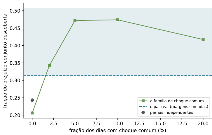
Figura 28.2: A fração do prejuízo conjunto que as margens somadas deixam descoberta, contra a fração dos dias com choque comum na família do capítulo da margem (com a correlação total do par, 0,589). A linha tracejada é o par real com o seu intervalo; o ponto escuro, as pernas independentes. O descoberto cresce com o choque e satura quando o choque deixa de ser cauda.
