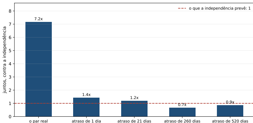
Figura 8.2: A barra da esquerda é o par como o mundo fez; as outras quatro são o mesmo par com o segundo mercado deslocado, e a linha tracejada é o que a independência prevê. Quase toda a dependência morre com um único dia de deslocamento.
