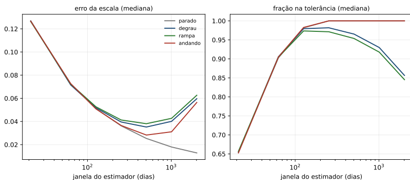
Figura 14.1: A varredura, forma por forma. À esquerda, o erro mediano da escala contra a janela do estimador: as formas que mudam fazem vale, com o fundo em quinhentos e quatro dias e subida de novo em seguida; o mundo parado desce sem virar. À direita, a fração de dias dentro da tolerância declarada: a tolerância não separa as formas — quem separa é o erro.
