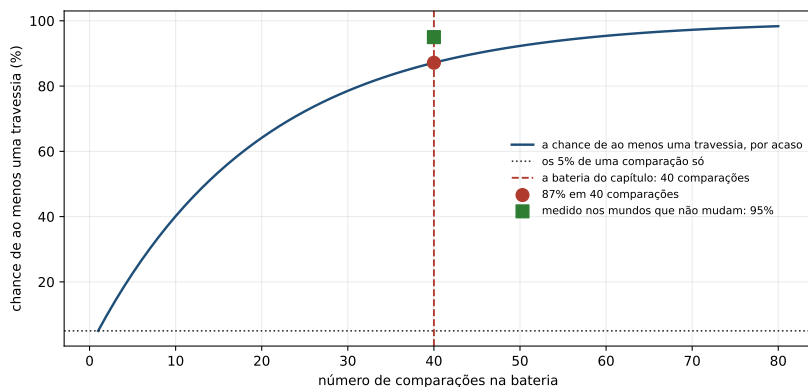
Figura 9.3: A barra de uma comparação e a barra da bateria. A curva é a chance de ao menos uma travessia por acaso, contra o número de comparações; a linha tracejada marca as 40 comparações do capítulo, e o ponto quadrado é o que a bateria mediu nos mundos que não mudam.
