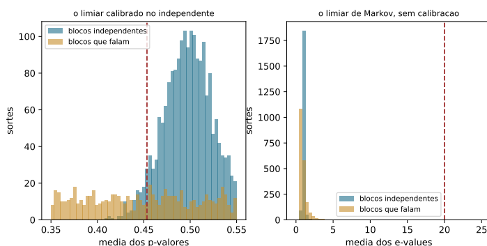
Figura 5.3: Por que uma rompe e as outras não. À esquerda, a média dos p-valores nos dois mundos: o mundo que fala é mais largo, e a massa à esquerda do limiar calibrado — o falso alarme — cresce de graça. À direita, a média dos e-values nos mesmos mundos: as duas distribuições ficam longe do limiar vermelho.
