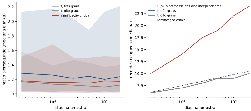
Figura 12.1: A razão entre os dois piores dias (esquerda) e a contagem de marcas (direita), contra o tamanho da amostra, em mediana e faixa: o t de três graus em azul, o de oito em cinza, a ramificação crítica em vermelho, e o harmônico tracejado — a promessa dos dias independentes. As três curvas da esquerda são horizontais; na direita, as duas do t andam coladas no tracejado e a da ramificação sobe sozinha para o dobro.
