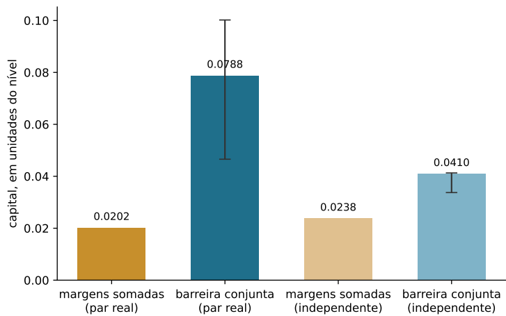
Figura 28.1: O capital que cobre a perda da carteira no nível prometido, em unidades do nível: as margens somadas e a barreira conjunta, no par real e nas pernas independentes, com o intervalo por reamostragem em blocos do dia nas barras conjuntas. A barreira correta do par real custa 3,901 vezes as margens somadas; nas independentes, 1,724.
