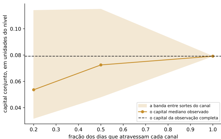
Figura 28.4: O capital conjunto observado contra a fração do canal, nas frações em que ele pode ser lido, com a banda entre sortes e a linha da observação completa. Na metade a banda já engole a linha: o capital não fica mais barato — fica ilegível. O décimo fica de fora do eixo: em quase todas as sortes o quantil nem existe — e o ponto do quinto só existe porque a mediana é lida nas sortes em que deu.
