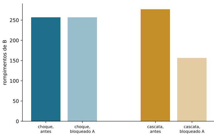
Figura 23.4: A intervenção: os rompimentos de B antes e depois do bloqueio de A, nos dois mundos. A barra clara do choque não desce — zero mortas; a da cascata desce quase à metade: a fração que dependia de A, que nenhum alinhamento devolvia.
