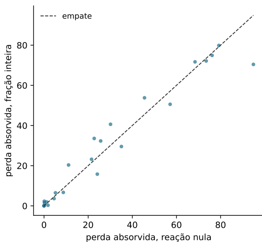
Figura 18.2: O preço pareado por mundo: a perda absorvida com a venda inteira no dia do rompimento contra a da reação nula, um ponto por mundo, na diagonal de empate. Os pontos caem onde a dispersão entre mundos manda: o efeito que a entrega vê é do tamanho do ruído na moeda da partilha.
