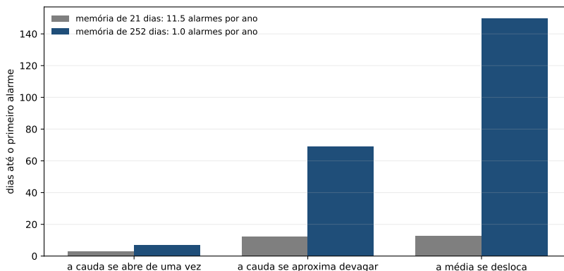
Figura 6.1: Dias até o primeiro alarme, por forma de mudança, em dois orçamentos: a memória de um mês, à esquerda de cada par, e a de um ano, à direita. O orçamento mais raro paga a diferença entre as formas.
