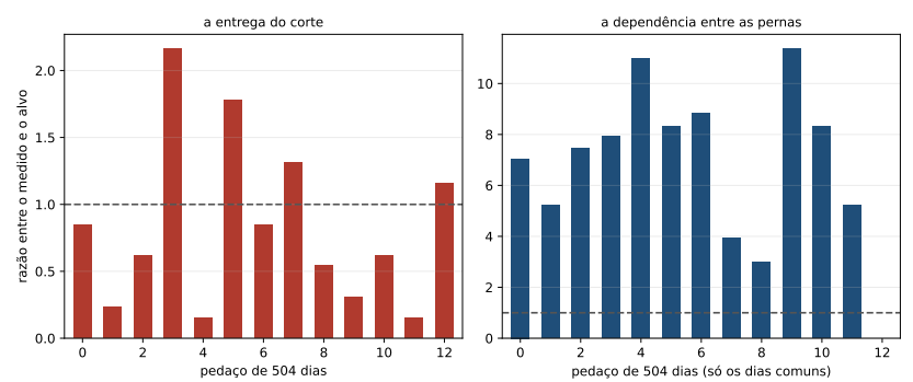
Figura 30.2: As duas conclusões no mesmo tamanho de pedaço, cada uma em razão do seu alvo. À esquerda, a entrega do corte, que atravessa a linha da promessa para os dois lados. À direita, a dependência, que fica sempre bem acima da independência.
