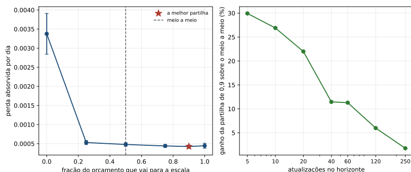
Figura 17.2: À esquerda, a perda contra a fração do orçamento que vai para a escala, com a dispersão entre mundos. O eixo da fração é linear, de modo que os três últimos pontos ficam amontoados à direita. À direita, o ganho da melhor partilha de 0,9 do orçamento para a escala contra o tamanho do orçamento: a vantagem de escolher bem encolhe quando o orçamento engorda.
