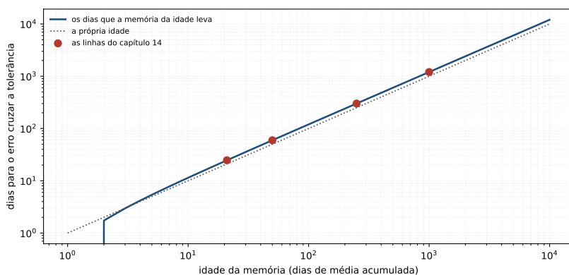
Figura 28.1: Os dias que a memória da idade leva para cruzar a tolerância, contra a idade dela. Os dois eixos são logarítmicos; a linha pontilhada é a própria idade, e os pontos são as quatro linhas que o capítulo da memória já publicava. A curva e a reta são paralelas, e é isso que faz do caso um caso sem conserto.
