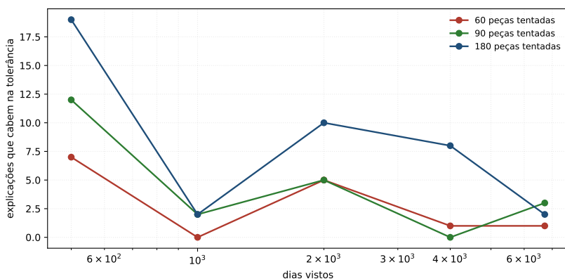
Figura 31.1: As explicações que cabem, contra os dias vistos, uma curva por tamanho de família. O eixo dos dias é logarítmico. A queda é a tendência, e não a regra: entre mil e quatro mil dias as curvas sobem e descem, e no extremo longo a família de 90 peças passa a de 180 — 3 contra 2.
