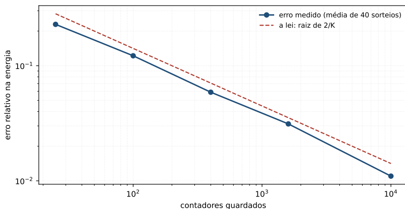
Figura 31.2: O erro do esboço contra o número de contadores guardados, nas duas escalas logarítmicas, com a reta da lei ao lado. As duas linhas são paralelas , e a medida fica abaixo da lei em toda a extensão: a média de uma estimativa simétrica custa cerca de oito décimos do desvio dela, e é isso que a distância entre as duas linhas mede.
