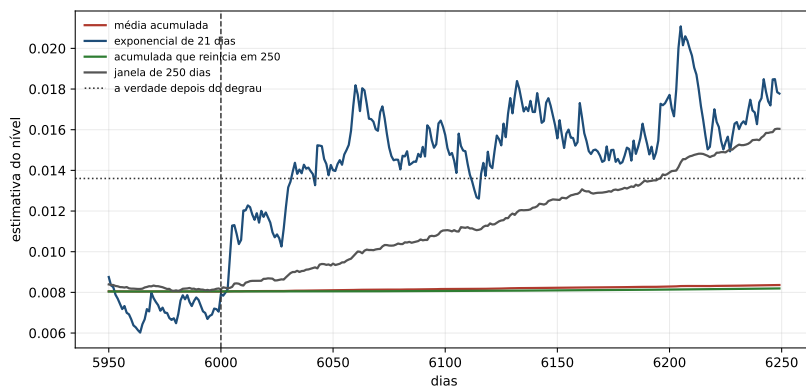
Figura 28.2: Os quatro estimadores em torno do dia do degrau, contra a verdade. Depois dele a exponencial de vinte e um dias reage e oscila em volta da linha; a janela sobe em rampa, porque vai sendo preenchida por dias novos; e a média acumulada e a que reinicia ficam paradas — elas carregam tanto passado que o degrau quase não as move dentro do horizonte da decisão.
