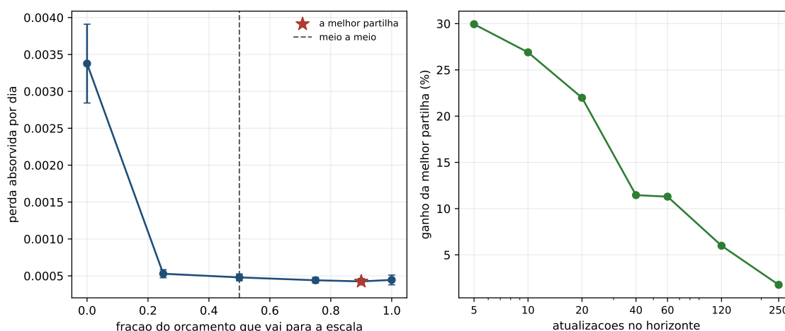
Figura 10.2: À esquerda, a perda contra a fração do orçamento que vai para a escala, com a dispersão entre mundos. À direita, o ganho da melhor partilha contra o tamanho do orçamento: a vantagem de escolher bem encolhe quando o orçamento engorda.
