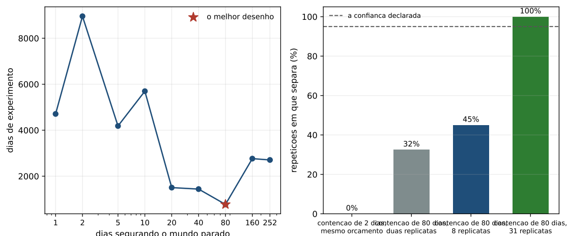
Figura 9.2: À esquerda, o preço do desenho que declara exatamente a diferença medida. À direita, a promessa do desenho verificada por repetição do experimento inteiro: a fração das repetições em que os dois intervalos de fato deixam de se cruzar.
