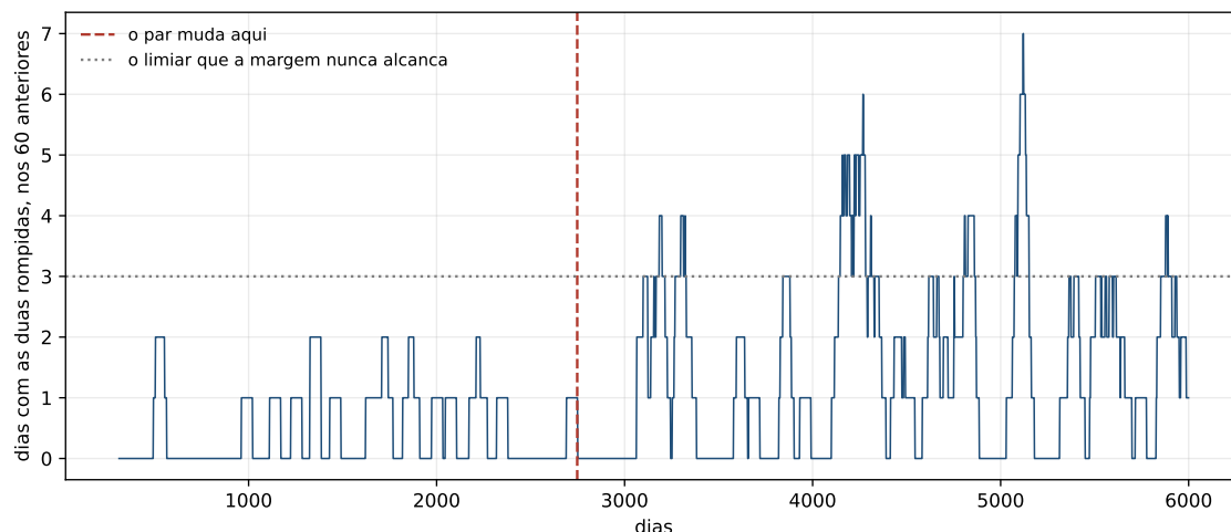
Figura 8.1: A contagem conjunta, dia a dia, com o dia da mudança e o limiar do meio. Antes da linha, a série é quase colada no chão; depois, os picos ficam mais altos e mais próximos. A mudança não aparece como degrau: aparece como mais dentes na linha, e quem procura um salto na figura não o encontra.
