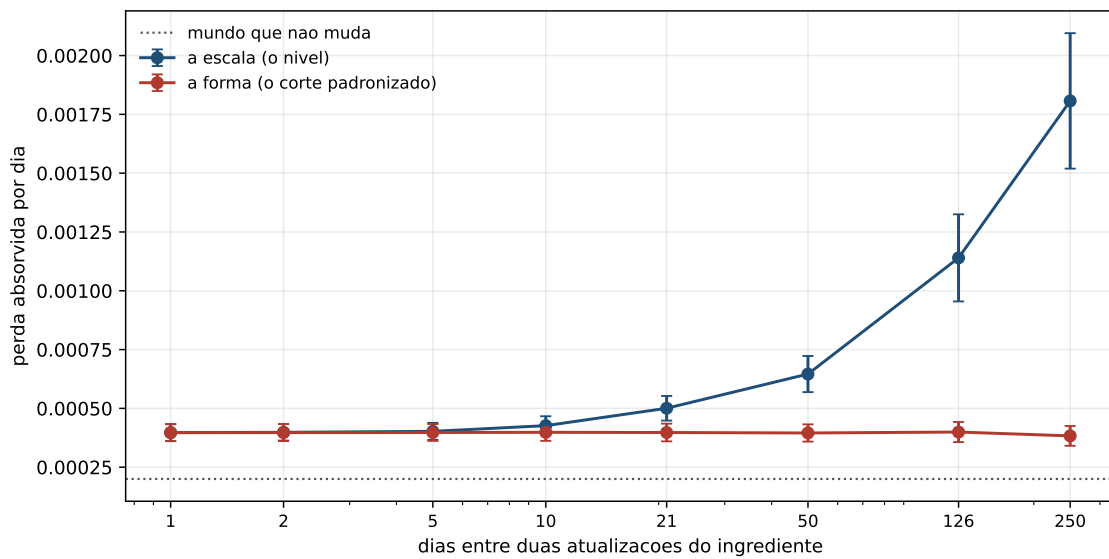
Figura 10.1: A perda absorvida contra o tempo entre duas atualizações, atualizando um ingrediente por vez. A linha pontilhada é o mesmo desenho num mundo que não muda.
