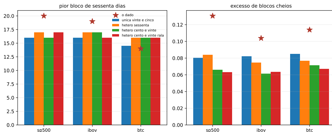
Figura 7.2: A mediana do pior bloco e a do excesso, por configuração e por mercado, com o valor do dado como estrela. As barras são medianas e as estrelas são pontos, sem dispersão desenhada: as faixas de dez a noventa por cento se sobrepõem, de modo que a distância aparente entre barra e estrela é maior do que a distância entre as distribuições.
