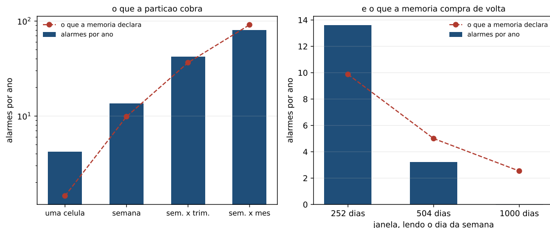
Figura 3.2: À esquerda, o que a partição cobra: alarmes por ano contra o que a memória declara, para as quatro leituras da tabela 3.2. À direita, o que a memória compra de volta, com a janela crescendo e a partição semanal fixa.
