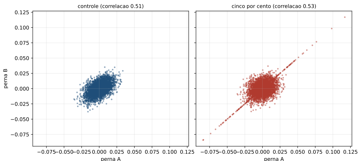
Figura 16.2: A nuvem das duas pernas no mundo gaussiano e no mundo com choque comum. O núcleo elíptico é o mesmo nos dois, e o que o segundo tem a mais é um braço na diagonal, que vai até os cantos.
