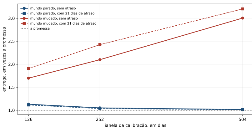
Figura 28.1: A entrega contra a janela da calibração, nos dois mundos e com e sem atraso. As duas curvas do mundo parado descem e as duas do mundo que muda sobem: o mesmo eixo, o sentido trocado.
