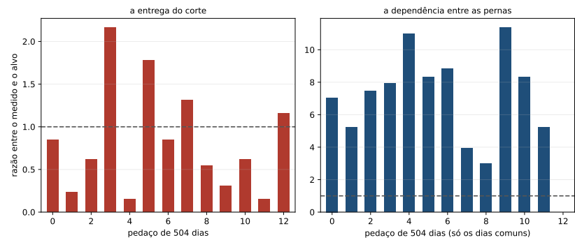
Figura 25.2: As duas conclusões no mesmo tamanho de pedaço, cada uma em razão do seu alvo. À esquerda, a entrega do corte, que atravessa a linha da promessa para os dois lados. À direita, a dependência, que fica sempre bem acima da independência.
