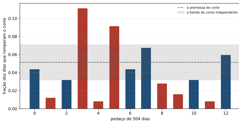
Figura 25.1: A entrega do corte em cada pedaço de 504 dias. A linha tracejada é a conta do corte e a faixa cinza é a banda de quem supõe dias independentes. As barras em vermelho são os pedaços que caem fora da banda.
