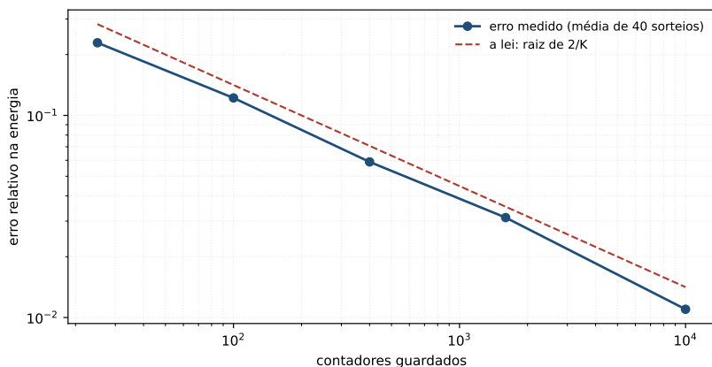
Figura 27.2: O erro do esboço contra o número de contadores guardados, nas duas escalas logarítmicas, com a reta da lei ao lado. As duas linhas são paralelas , e a medida fica abaixo da lei em toda a extensão: a média de uma estimativa simétrica custa cerca de oito décimos do desvio dela, e é isso que a distância entre as duas linhas mede.
