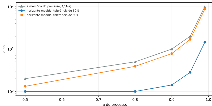
Figura 22.2: A memória do processo e os dois horizontes de recuperação, contra a . São três medidas do mesmo sistema, e cada uma responde a uma pergunta diferente — a curva mais alta é a da memória, e as outras duas são horizontes de recuperação. O eixo dos dias é logarítmico, porque a grandeza só age no fim da escala.
