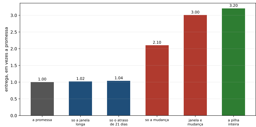
Figura 28.2: A entrega de cada buraco sozinho e a da pilha inteira, em vezes a promessa. A barra verde é a mais alta das seis, e o que essa altura diz é o que o livro inteiro perseguiu: os buracos não se somam, eles se encaixam.
