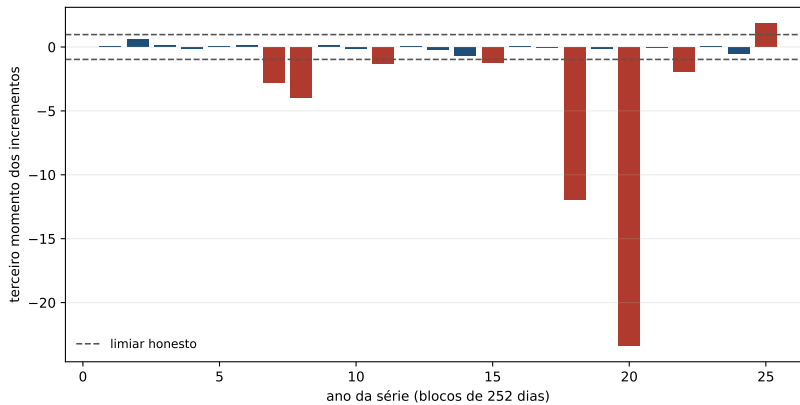
Figura 19.2: O terceiro momento dos incrementos, ano a ano, no índice americano, com o limiar honesto. As barras em vermelho são os anos em que o vigia alarmaria.
