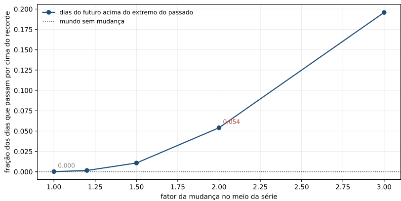
Figura 21.2: A fração dos dias seguintes que passam por cima do recorde de tudo o que veio antes, contra o tamanho da mudança. A linha pontilhada é o mundo que não muda.
