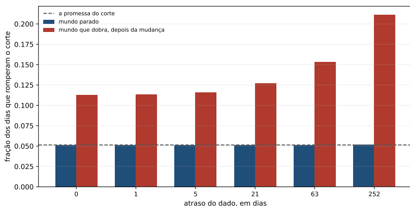
Figura 26.2: O mundo parado e o mundo que dobra, por atraso — o parado medido na série inteira e o que dobra na janela que segue a mudança. A barra azul é o controle: ela fica na promessa em todos os atrasos.
