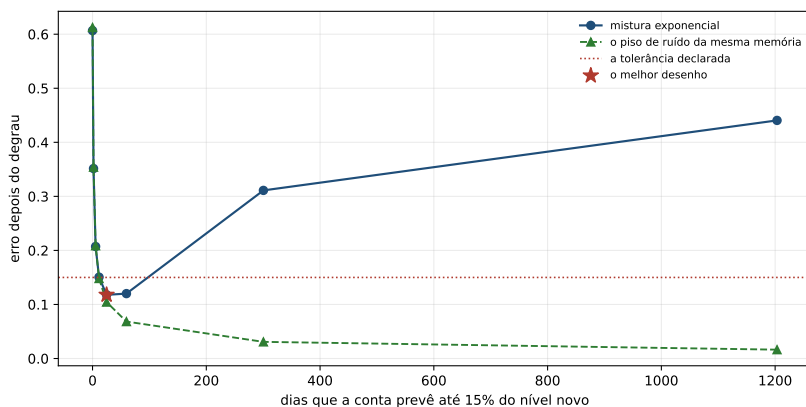
Figura 18.2: O erro depois do degrau contra os dias que a conta do cruzamento prevê até 0,15 do nível novo. A curva tracejada é o piso de ruído da mesma memória: onde ela alcança a curva de cima, o erro deixou de ser atraso e passou a ser tamanho de amostra.
