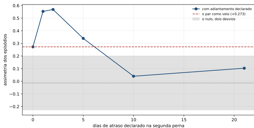
Figura 20.1: A assimetria contra o atraso declarado na segunda perna. A faixa cinza é o nulo a dois desvios sem deslocamento, a linha tracejada é o par como veio, e a curva é o par com o atraso declarado — que o nulo também sofre, e é o que o texto mede.
