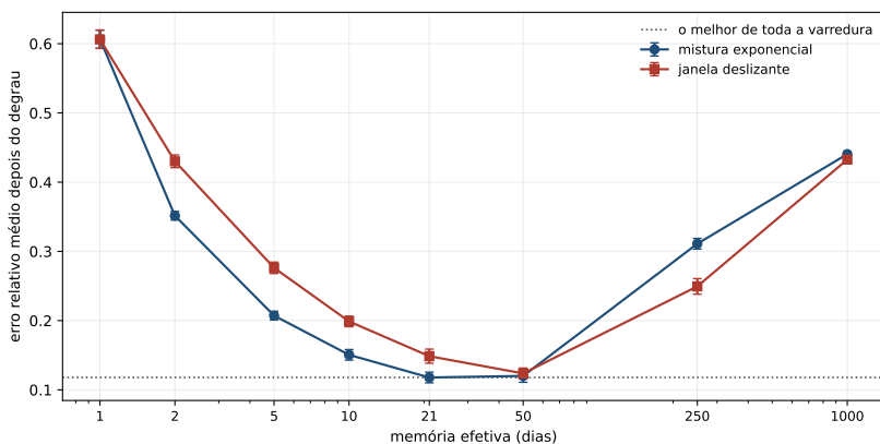
Figura 18.1: O erro depois do degrau contra a memória efetiva, nas duas formas de esquecer. A linha pontilhada é o melhor erro de toda a varredura. O eixo da memória é logarítmico: distâncias iguais no papel são multiplicações iguais no tempo de memória.
