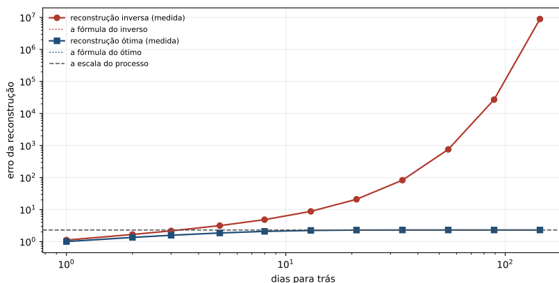
Figura 22.1: O erro das duas reconstruções contra os dias para trás, com a escala do processo como linha de referência. Os pontos são medidos e as linhas pontilhadas são as formas fechadas da proposição 22.1. Os dois eixos são logarítmicos, de modo que a reta do desenho vale uma potência.
