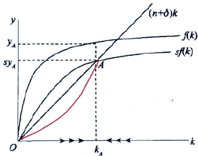
图 20—4 新古典模型的稳态
