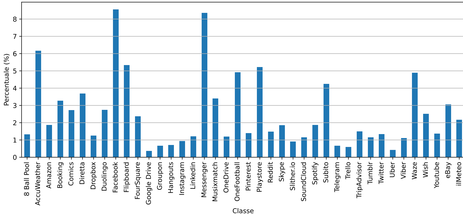
Distribuzione percentuale classi - Dataset 50k
