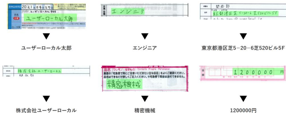
手書きOCR
